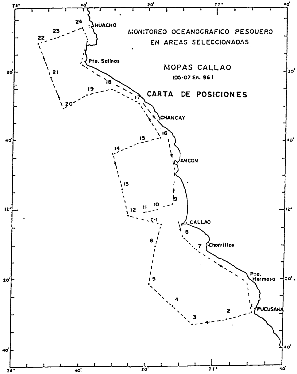
Fig. 12. Carta de trayecto y estaciones. MOPAS Callao (05-07 Ene. 1996).
