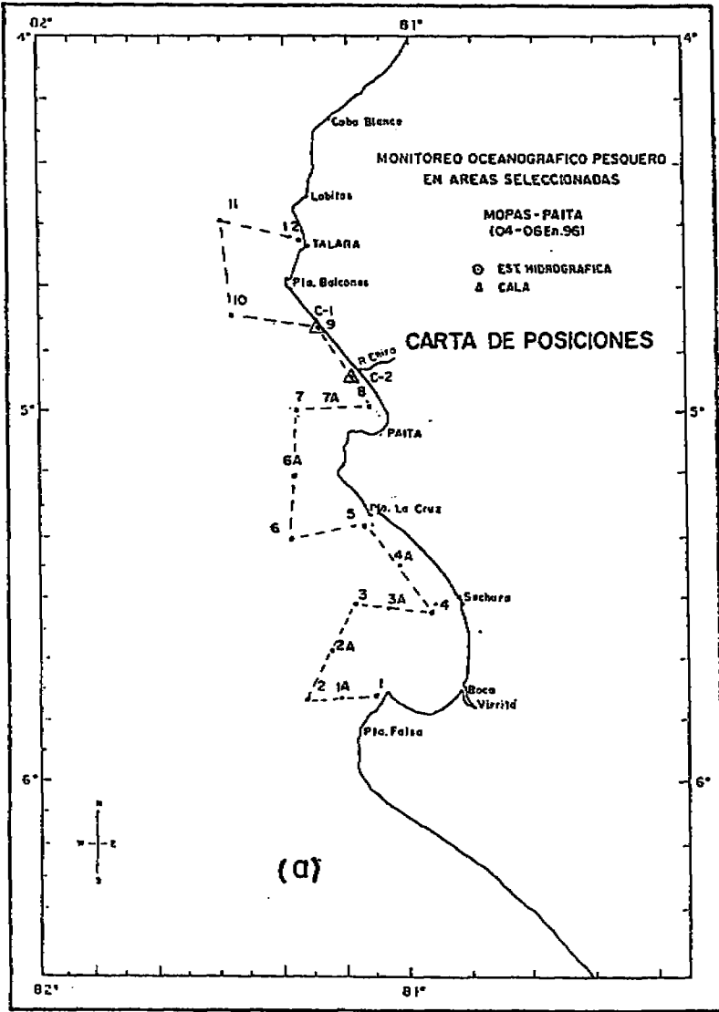
Fig. 1. Carta de trayecto y estaciones (a) y distribución de la Temperatura Superficial (b). MOPAS Paita (04-06 Enero 1996).
