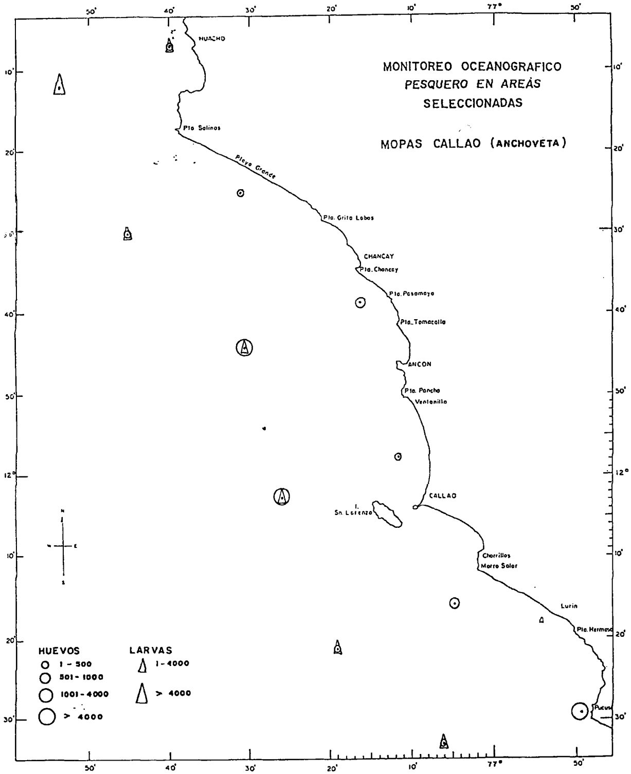
Fig. 16. Distribución y abundancia de huevos y larvas de anchoveta en el Callao - MOPAS 9601.
