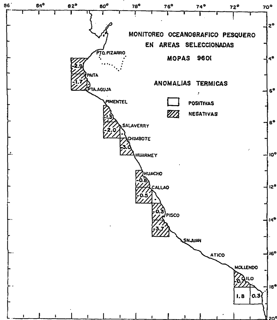
Fig. 4. Anomalías Térmicas (°C) respecto al promedio patrón de Enero.
