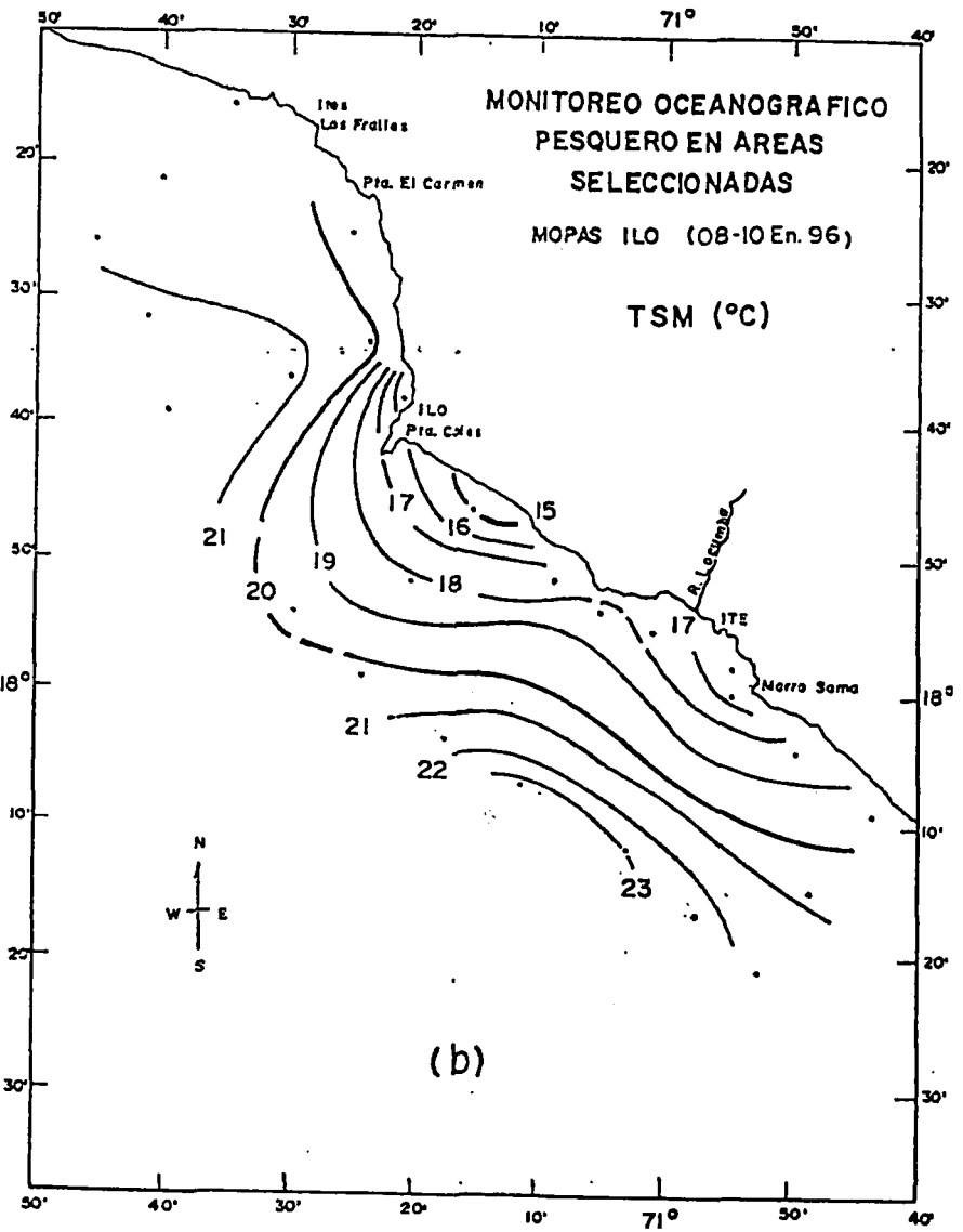
Fig. 22. Carta de trayecto y estaciones (a) y distribución de la Temperatura Superficial de amr (b). MOPAS Ilo (08-10 Ene. 1996).
