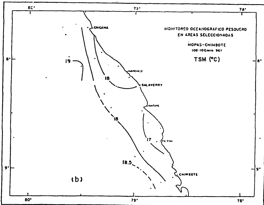
Fig. 7. Carta de trayecto y estaciones (a) y distribución de la Temperatura (b). MOPAS Chimbote (08-10 Ene. 1996).
