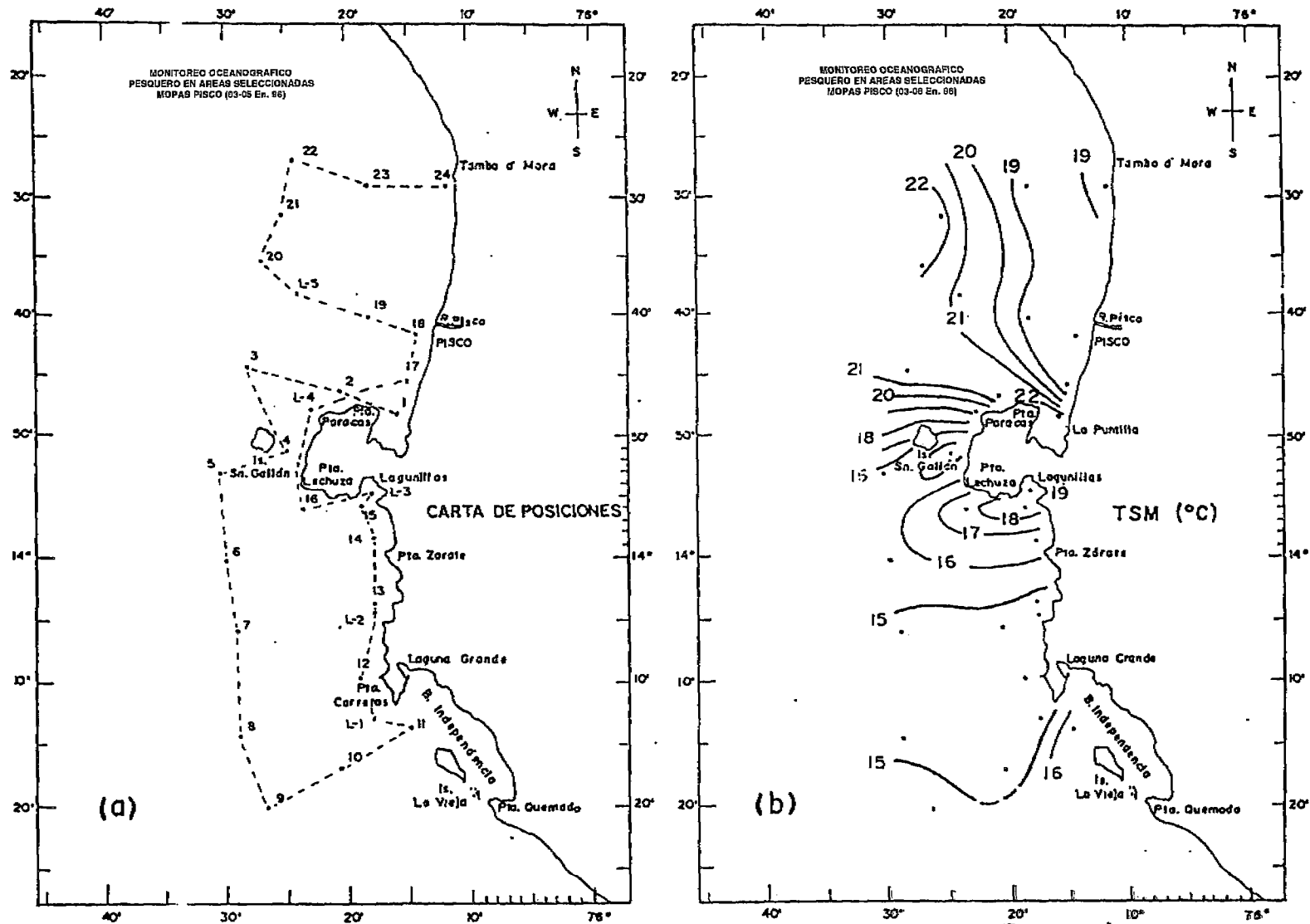
Fig. 17. Carta de trayecto y estaciones (a) y distribución de la Temperatura Superficial del mar. MOPAS Pisco (03-05 Ene. 96).
