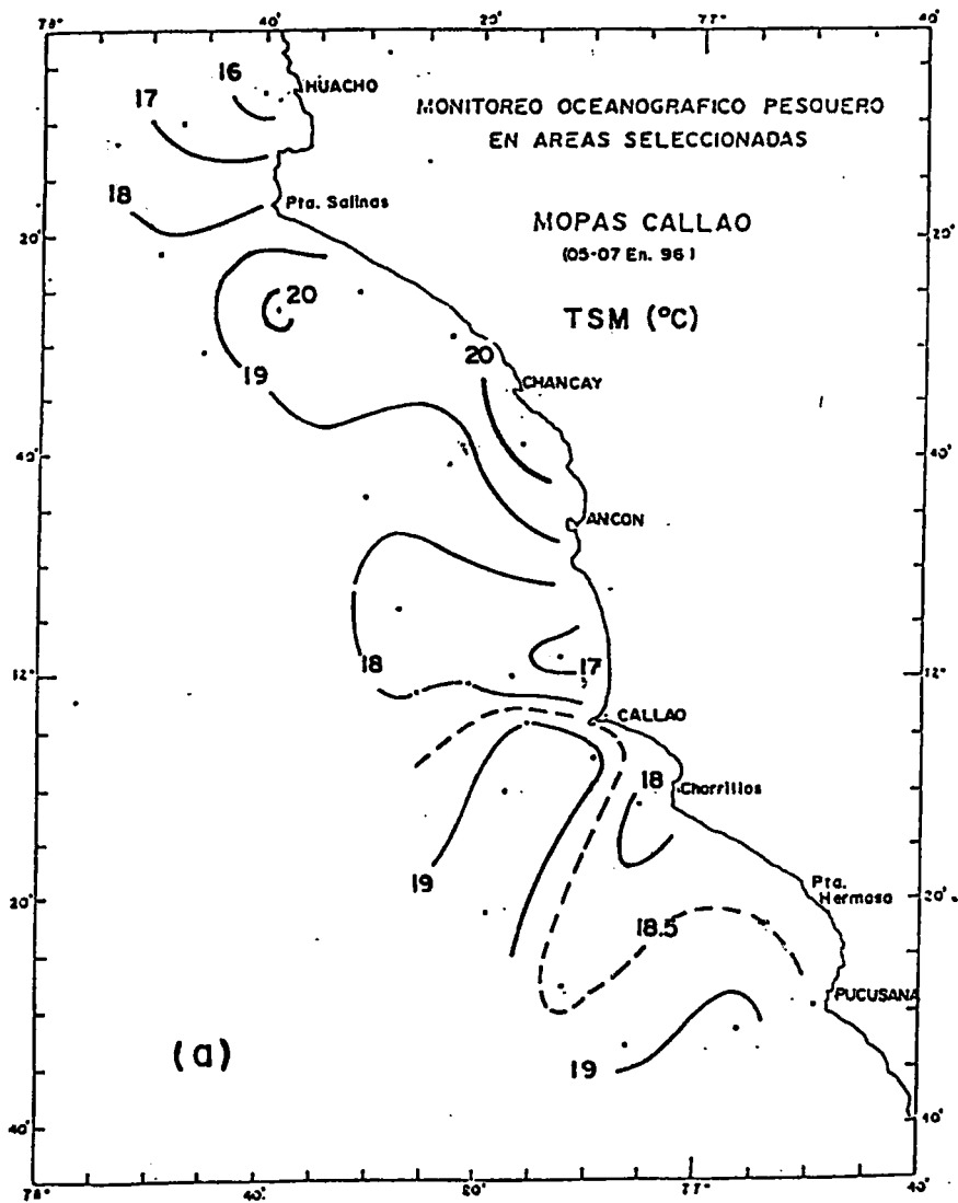
Fig. 13. Distribución de la Temperatura (a) y Salinidad (b), en la superficie del mar MOPAS Callao (05-07 Ene. 1996).
