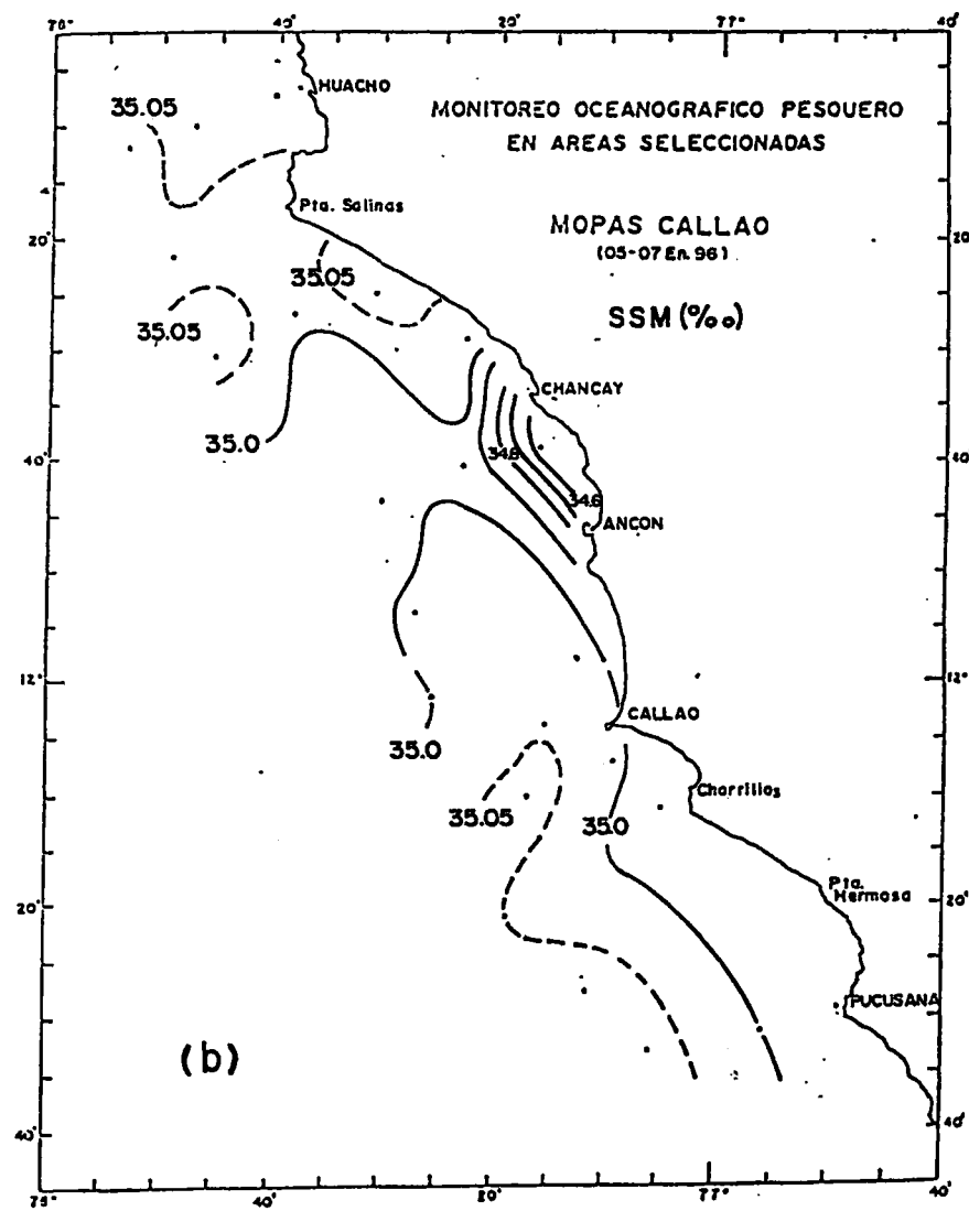
Fig. 13. Distribución de la Temperatura (a) y Salinidad (b), en la superficie del mar MOPAS Callao (05-07 Ene. 1996).
