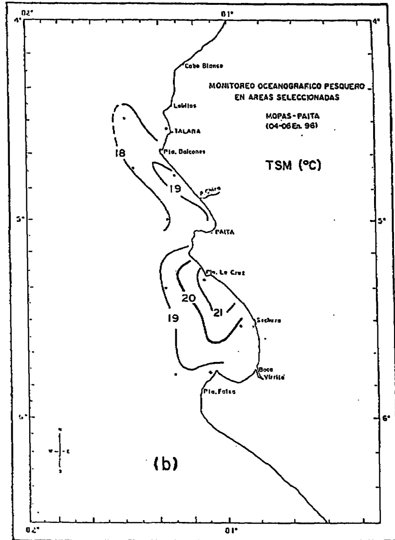
Fig. 1. Carta de trayecto y estaciones (a) y distribución de la Temperatura Superficial (b). MOPAS Paita (04-06 Enero 1996).
