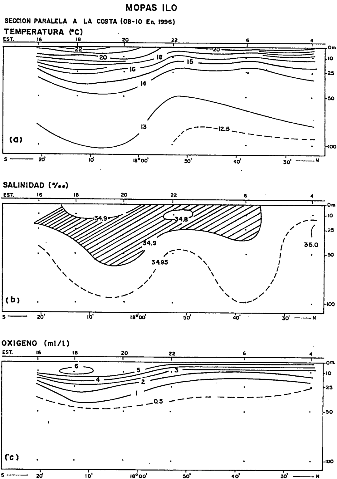
Fig. 24. Secciones Verticales de Temperatura, Salinidad y Oxígeno, alrededor de las 15 mn frente a Ilo, con datos del MOPAS ILO (08-10 Ene. 1996).
