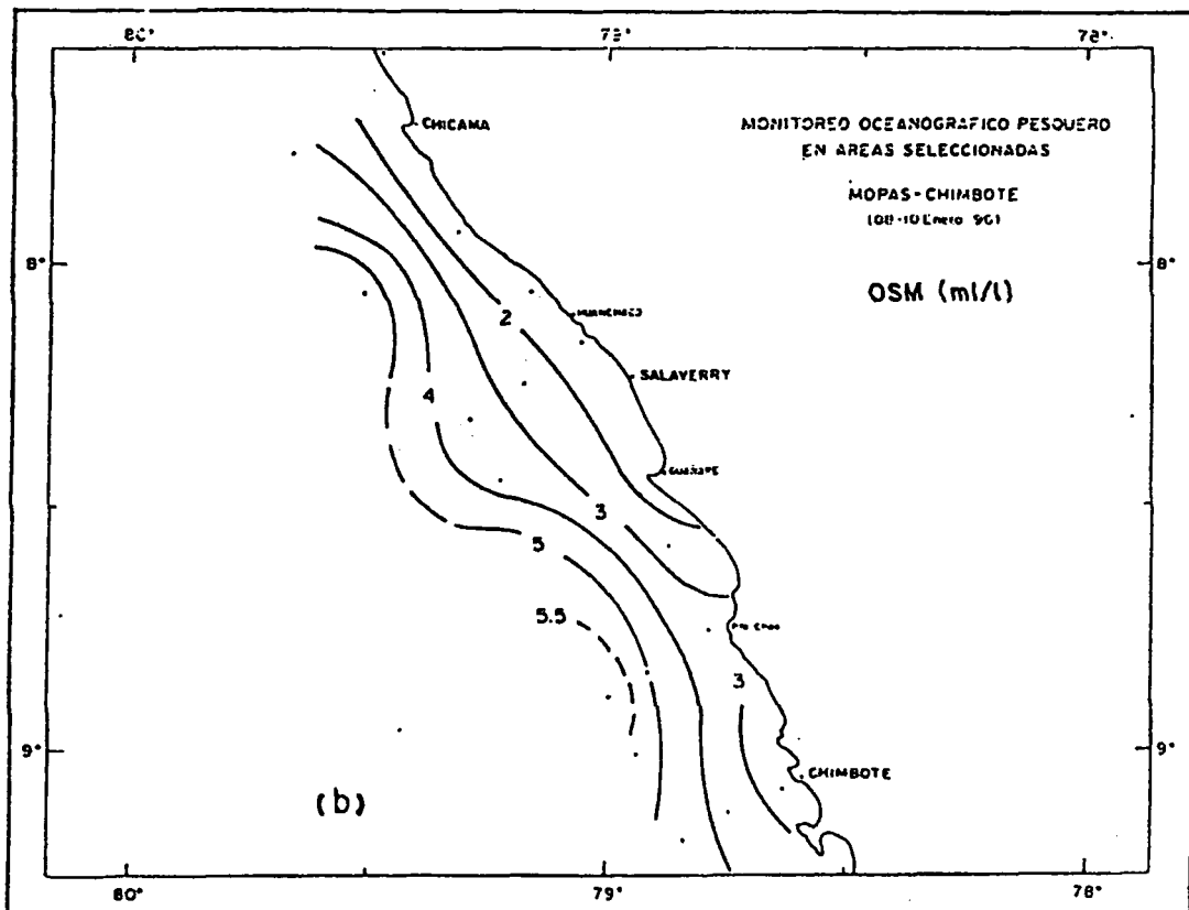
Fig. 8. Distribución de la Salinidad (a) y Oxígeno (b), en la superficie del mar. MOPAS Chimbote (08-10 Ene. 1996).
