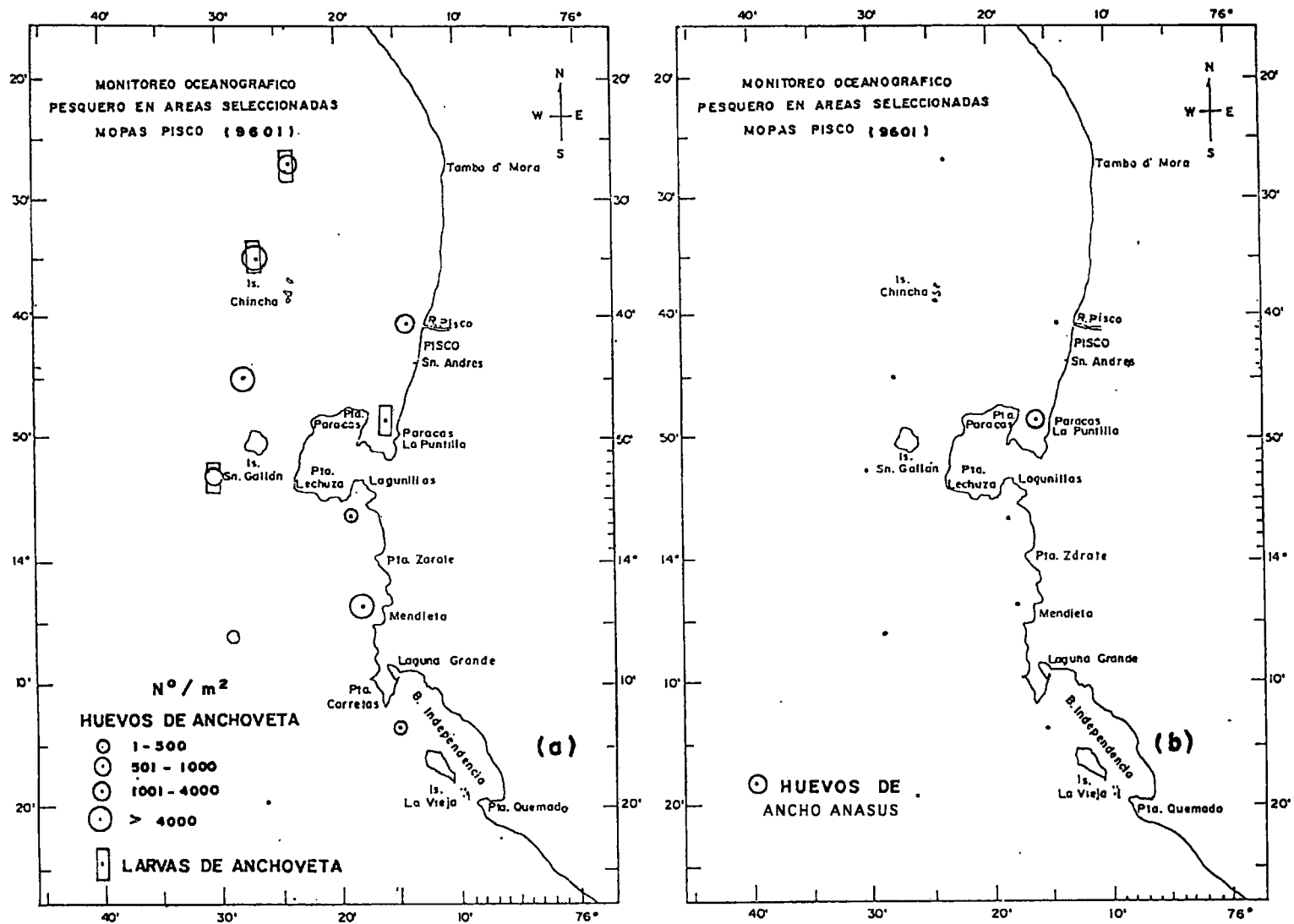
Fig. 21. Distribución y abundancia de huevos y larvas de anchoveta (a) y huevos de anchoa nasus (b) en Pisco - MOPAS 9601.
