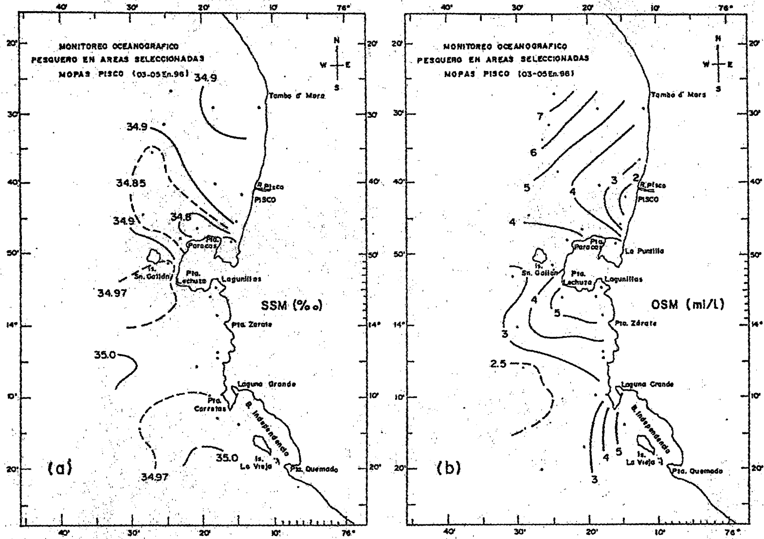
Fig. 18. Distribución de la Salinidad (a) y Oxígeno (b) en la superficie del mar. MOPAS Pisco (03-05 Ene. 96).
