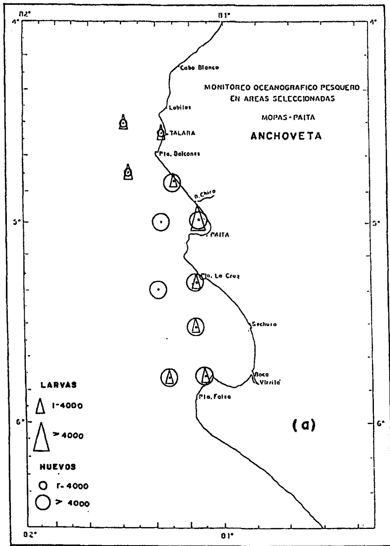
Fig. 6. Distribución y abundancia de huevos y larvas de anchoveta (a) y de sardina (b) en Paita - MOPAS 9601.
