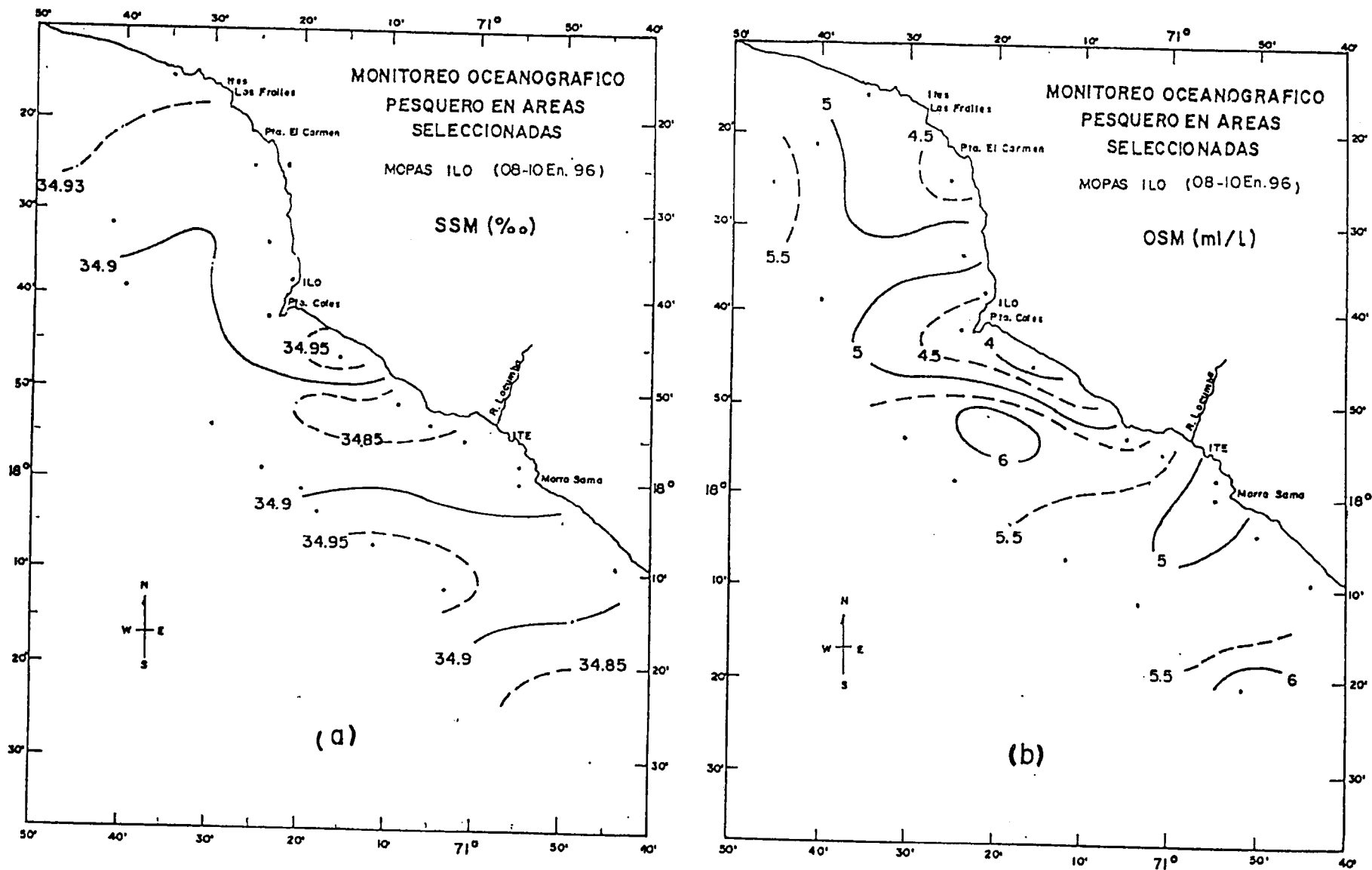
Fig. 23. Distribución de la Salinidad (a) y Oxígeno (b) en la superficie del mar. MOPAS Ilo (08-10 Ene. 96).
