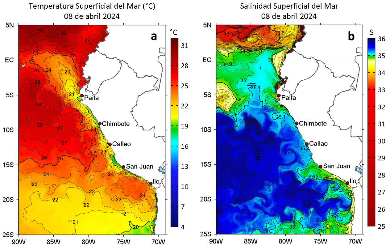
Figura 2. a) Temperatura superficial del mar (°C) y b) Salinidad superficial del mar para el 08 de abril de 2024. Datos: OSTIA-UKMO-L4-GLOB-v2.0 (UK Met Office, 2012; Donlon et al, 2012) y del GLOBAL_ANALYSISFORECAST_PHY_001_024 (Lellouche, J. M. et al, 2013), respectivamente.
