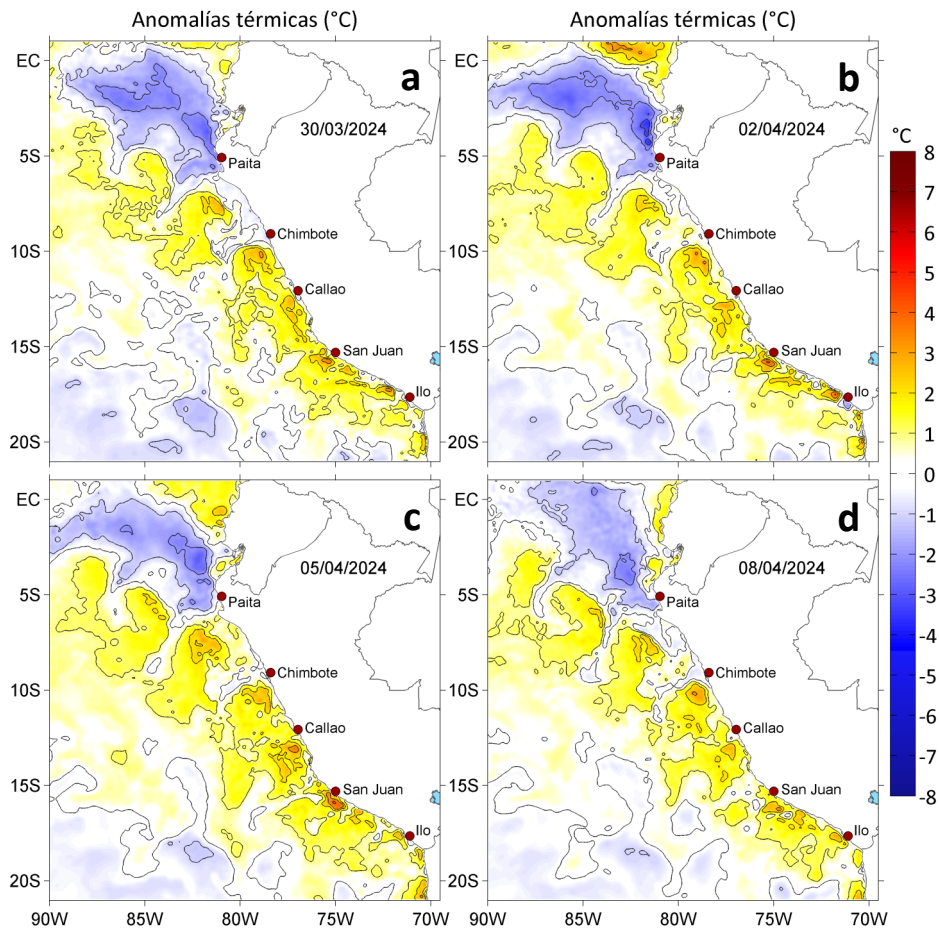
Figura 3. Anomalías de la temperatura superficial del mar (°C) para el a) 30 de marzo, b) 02, c) 05 y d) 08 de abril de 2024. Las anomalías se calcularon respecto de la climatología para el periodo 1991-2020. Datos: OSTIA-UKMO-L4-GLOB-v2.0 (UK Met Office, 2012; Donlon et al, 2012).
