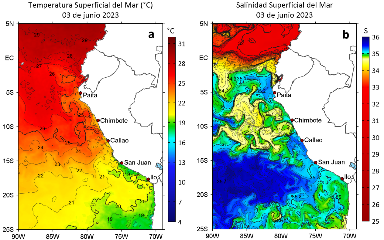
Figura 2. a) Temperatura superficial del mar ( ^{\circ}\text{C} ) y b) Salinidad superficial del mar para el 03 de junio de 2023. Datos: OSTIA-UKMO-L4-GLOB-v2.0 (UK Met Office, 2012; Donlon et al, 2012) y del GLOBAL_ANALYSISFORECAST_PHY_001_024 (Lellouche, J. M. et al, 2013), respectivamente.
