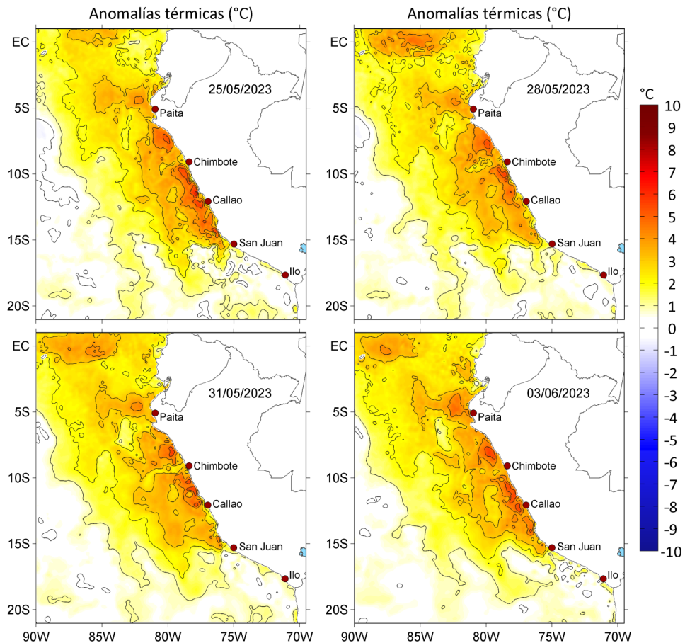
Figura 3. Anomalías de la temperatura superficial del mar ( ^{\circ}\text{C} ) para el a) 25, b) 28 y c) 31 de mayo, así como para el d) 03 de junio de 2023. Las anomalías se calcularon respecto de la climatología para el periodo 2007-2016. Datos: OSTIA-UKMO-L4-GLOB-v2.0 (UK Met Office, 2012; Donlon et al, 2012).
