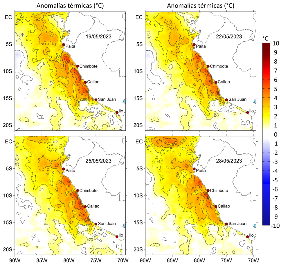
Figura 3. Anomalías de la temperatura superficial del mar ( ^{\circ}\text{C} ) para el a) 19, b) 22, c) 25 y d) 28 de mayo de 2023. Las anomalías se calcularon respecto de la climatología para el periodo 2007-2016. Datos: OSTIA-UKMO-L4-GLOB-v2.0 (UK Met Office, 2012; Donlon et al, 2012).
