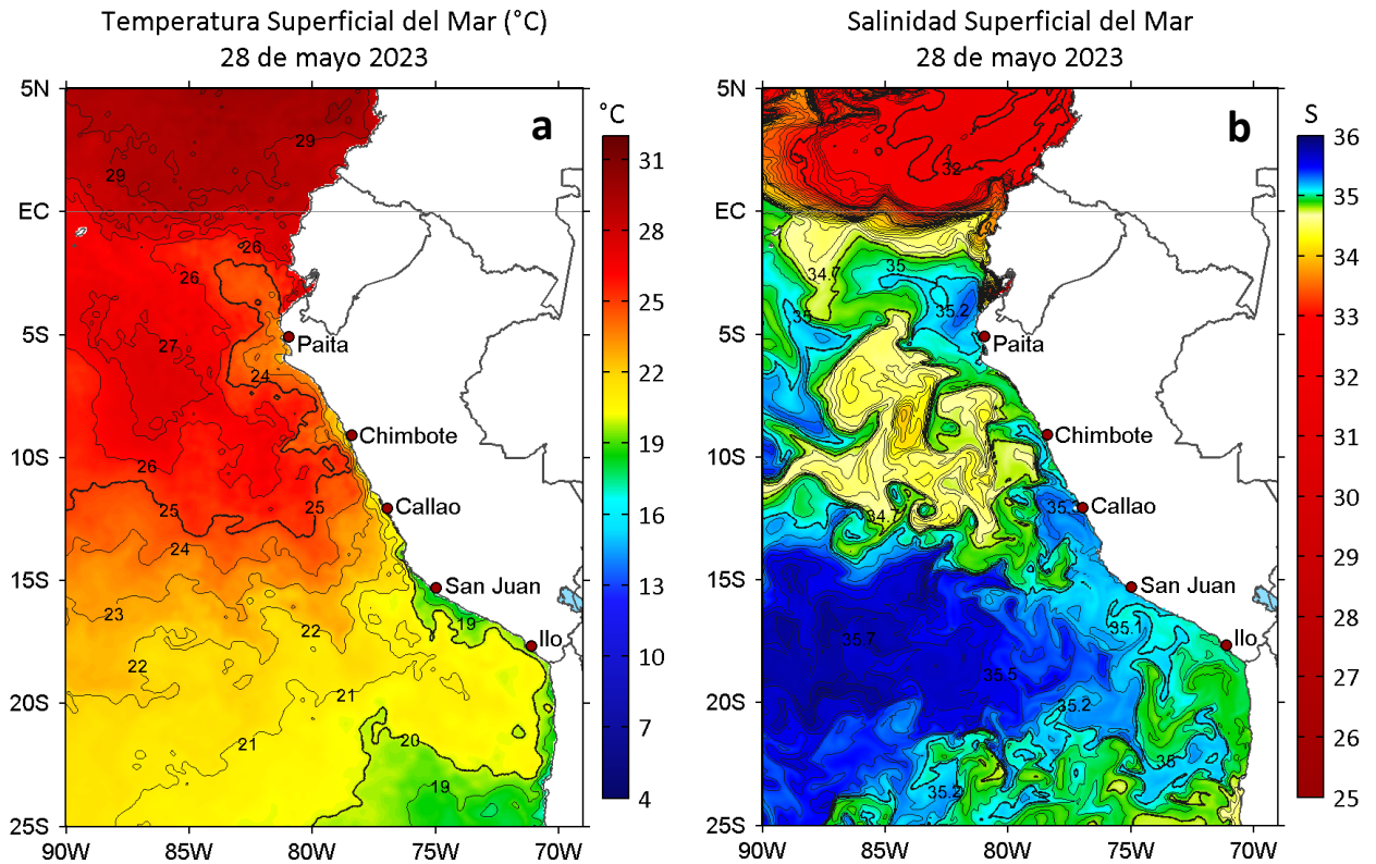
Figura 2. a) Temperatura superficial del mar ( ^{\circ}\text{C} ) y b) Salinidad superficial del mar para el 28 de mayo de 2023. Datos: OSTIA-UKMO-L4-GLOB-v2.0 (UK Met Office, 2012; Donlon et al, 2012) y del GLOBAL_ANALYSISFORECAST_PHY_001_024 (Lellouche, J. M. et al, 2013), respectivamente.
