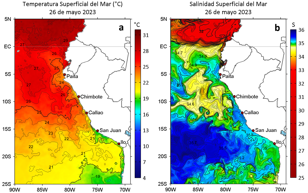
Figura 2. a) Temperatura superficial del mar ( ^{\circ}\text{C} ) y b) Salinidad superficial del mar para el 26 de mayo de 2023. Datos: OSTIA-UKMO-L4-GLOB-v2.0 (UK Met Office, 2012; Donlon et al, 2012) y del GLOBAL_ANALYSISFORECAST_PHY_001_024 (Lellouche, J. M. et al, 2013), respectivamente.
