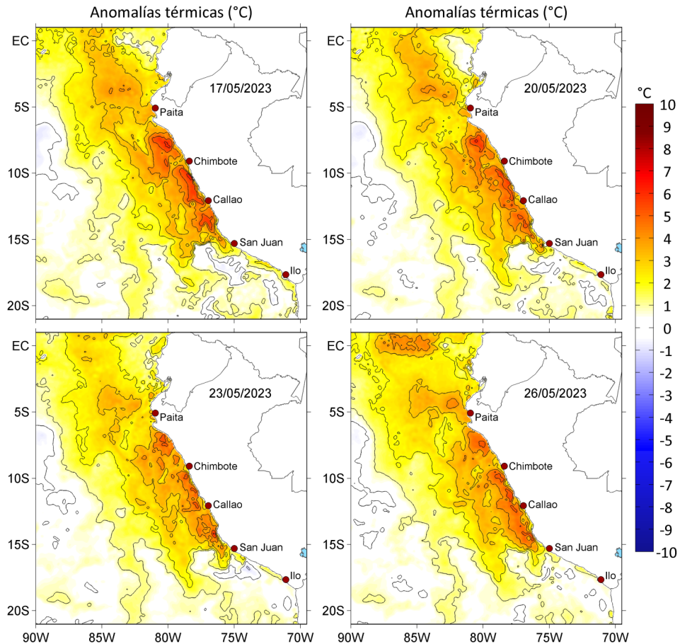
Figura 3. Anomalías de la temperatura superficial del mar ( ^{\circ}\text{C} ) para el a) 17, b) 20, c) 23 y d) 26 de mayo de 2023. Las anomalías se calcularon respecto de la climatología para el periodo 2007-2016. Datos: OSTIA-UKMO-L4-GLOB-v2.0 (UK Met Office, 2012; Donlon et al, 2012).
