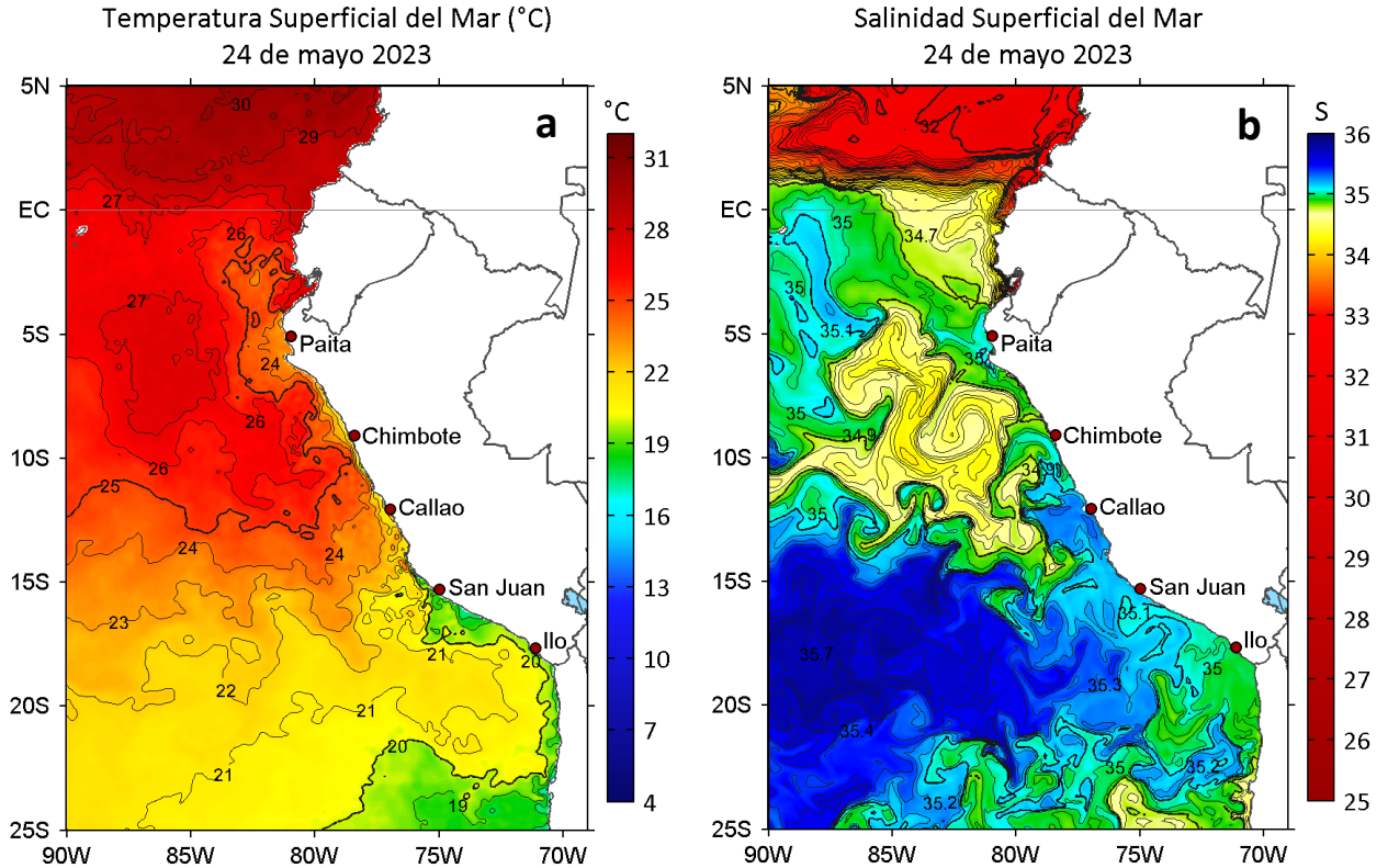
Figura 2. a) Temperatura superficial del mar ( ^{\circ}\text{C} ) y b) Salinidad superficial del mar para el 24 de mayo de 2023. Datos: OSTIA-UKMO-L4-GLOB-v2.0 (UK Met Office, 2012; Donlon et al, 2012) y del GLOBAL_ANALYSISFORECAST_PHY_001_024 (Lellouche, J. M. et al, 2013), respectivamente.
