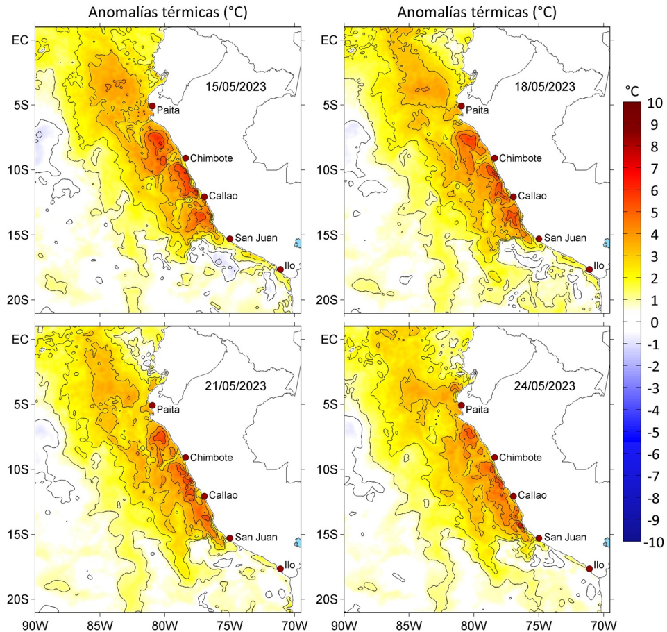
Figura 3. Anomalías de la temperatura superficial del mar ( ^{\circ}\text{C} ) para el a) 15, b) 18, c) 21 y d) 24 de mayo de 2023. Las anomalías se calcularon respecto de la climatología para el periodo 2007-2016. Datos: OSTIA-UKMO-L4-GLOB-v2.0 (UK Met Office, 2012; Donlon et al, 2012).
