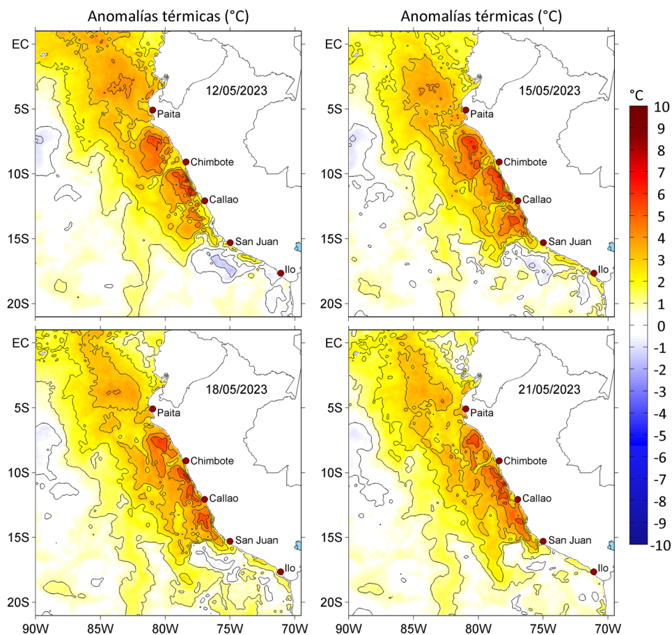
Figura 3. Anomalías de la temperatura superficial del mar ( ^{\circ}\text{C} ) para el a) 12, b) 15, c) 18 y d) 21 de mayo de 2023. Las anomalías se calcularon respecto de la climatología para el periodo 2007-2016. Datos: OSTIA-UKMO-L4-GLOB-v2.0 (UK Met Office, 2012; Donlon et al, 2012).
