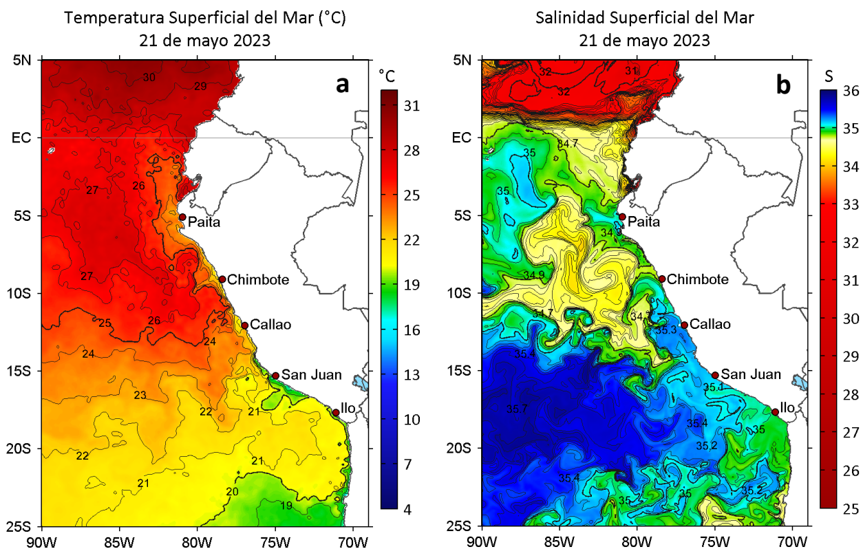
Figura 2. a) Temperatura superficial del mar ( ^{\circ}\text{C} ) y b) Salinidad superficial del mar para el 21 de mayo de 2023. Datos: OSTIA-UKMO-L4-GLOB-v2.0 (UK Met Office, 2012; Donlon et al, 2012) y del GLOBAL_ANALYSISFORECAST_PHY_001_024 (Lellouche, J. M. et al, 2013), respectivamente.
