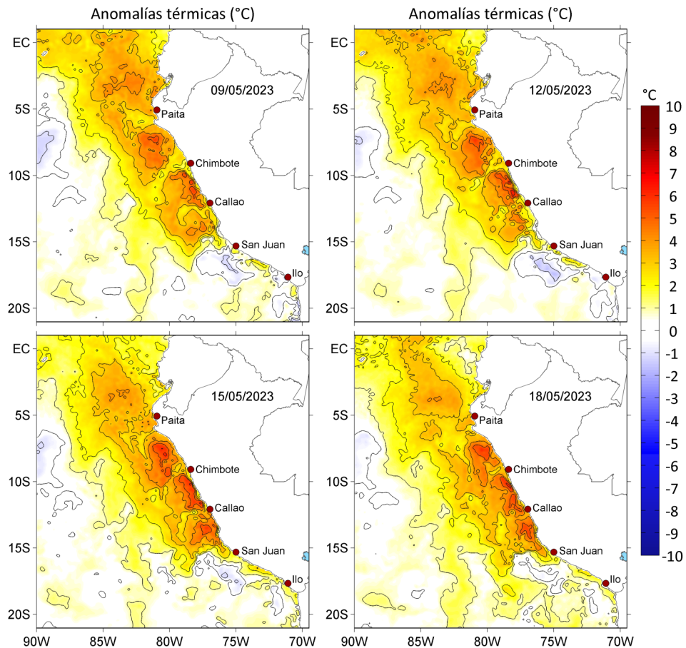
Figura 3. Anomalías de la temperatura superficial del mar ( ^{\circ}\text{C} ) para el a) 09, b) 12, c) 15 y d) 18 de mayo de 2023. Las anomalías se calcularon respecto de la climatología para el periodo 2007-2016. Datos: OSTIA-UKMO-L4-GLOB-v2.0 (UK Met Office, 2012; Donlon et al, 2012).
