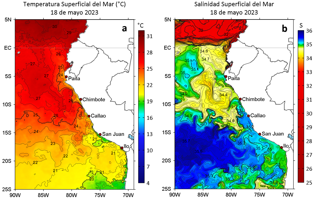
Figura 2. a) Temperatura superficial del mar ( ^{\circ}\text{C} ) y b) Salinidad superficial del mar para el 18 de mayo de 2023. Datos: OSTIA-UKMO-L4-GLOB-v2.0 (UK Met Office, 2012; Donlon et al, 2012) y del GLOBAL_ANALYSISFORECAST_PHY_001_024 (Lellouche, J. M. et al, 2013), respectivamente.
