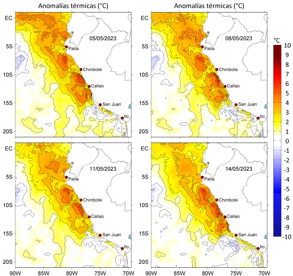
Figura 3. Anomalías de la temperatura superficial del mar (°C) para el a) 05, b) 08, c) 11 y d) 14 de mayo de 2023. Las anomalías se calcularon respecto de la climatología para el periodo 2007-2016. Datos: OSTIA-UKMO-L4-GLOB-v2.0 (UK Met Office, 2012; Donlon et al, 2012).
