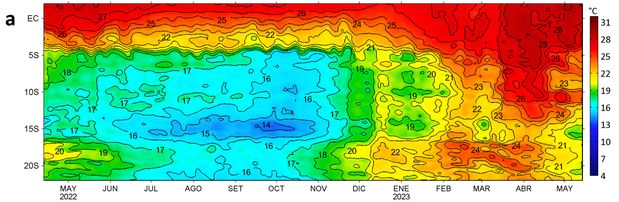
Anomalías de la Temperatura Superficial del mar (°C), franja costera de 60 m.n. 13 de abril 2022 - 14 de mayo 2023
