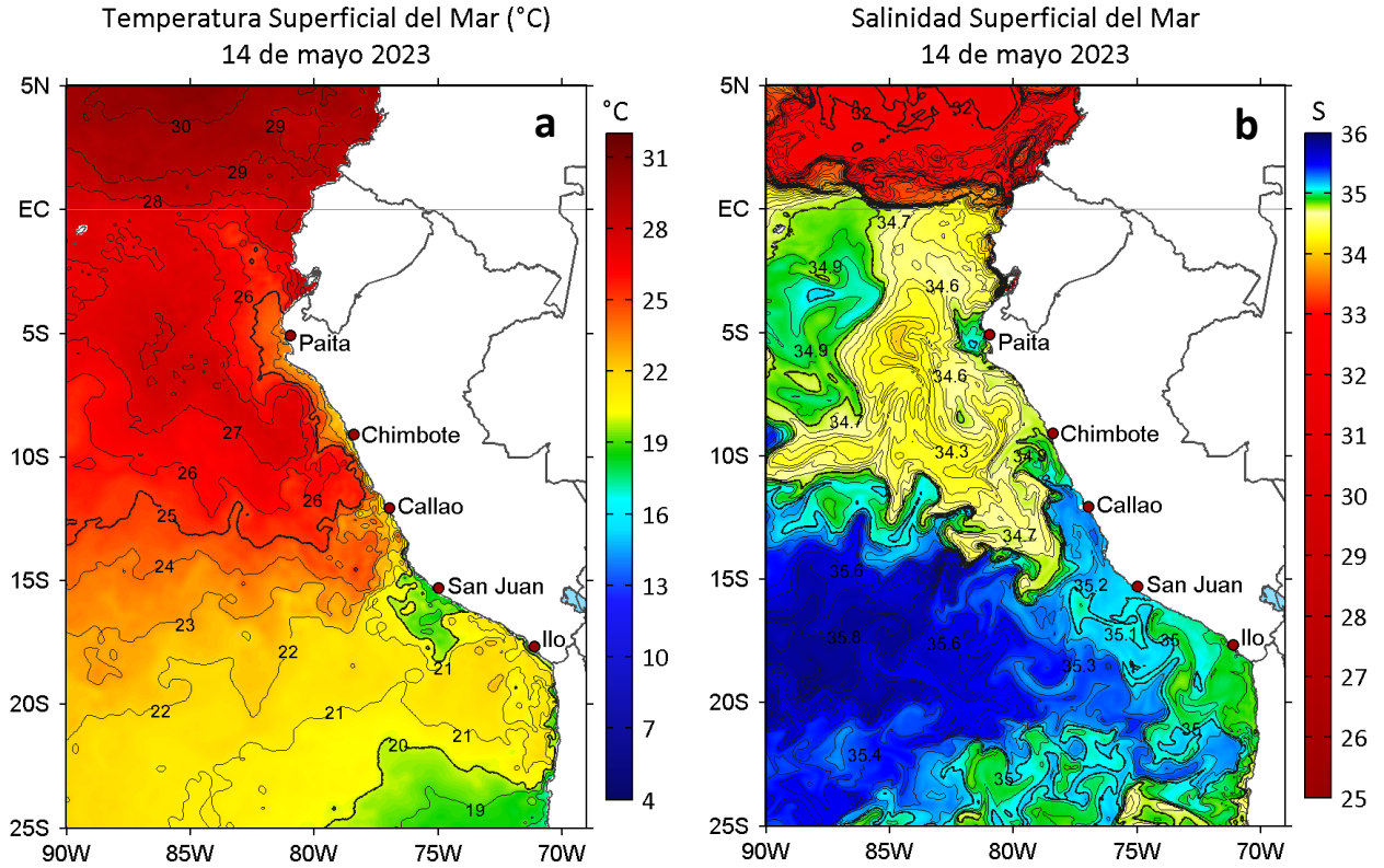
Figura 2. a) Temperatura superficial del mar (°C) y b) Salinidad superficial del mar para el 14 de mayo de 2023. Datos: OSTIA-UKMO-L4-GLOB-v2.0 (UK Met Office, 2012; Donlon et al, 2012) y del GLOBAL_ANALYSISFORECAST_PHY_001_024 (Lellouche, J. M. et al, 2013), respectivamente.
