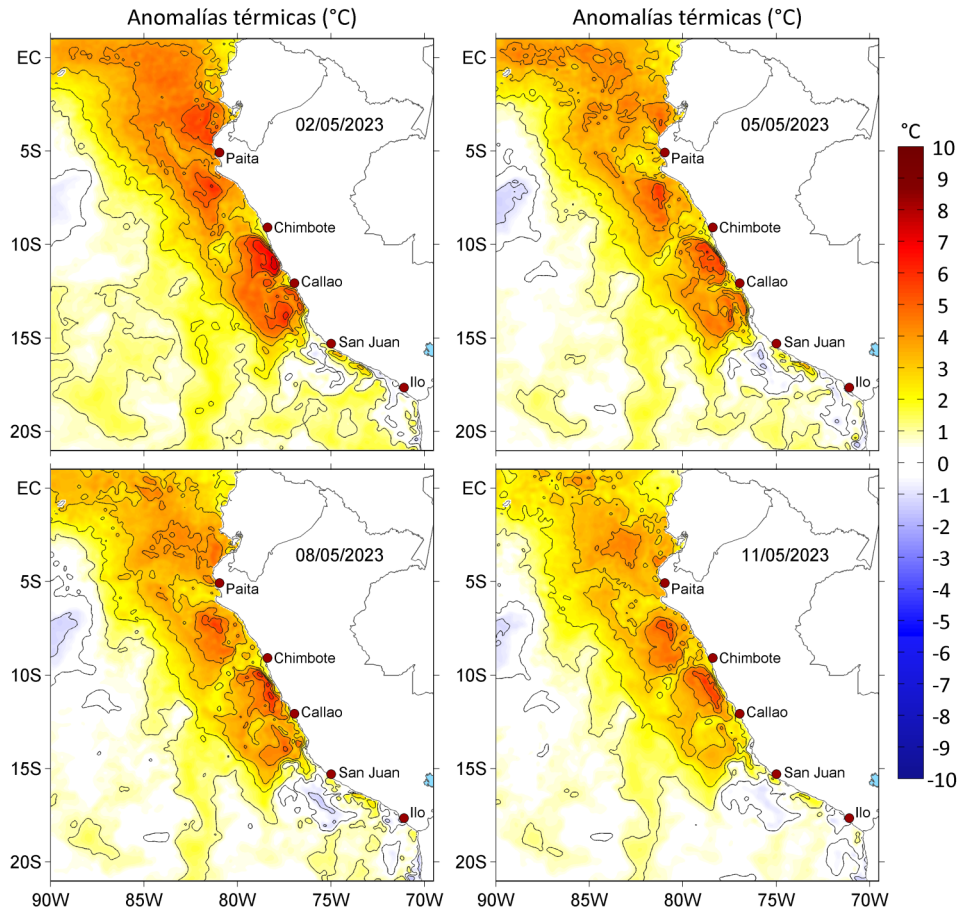
Figura 3. Anomalías de la temperatura superficial del mar ( ^{\circ}\text{C} ) para el a) 02, b) 05, c) 08 y d) 11 de mayo de 2023. Las anomalías se calcularon respecto de la climatología para el periodo 2007-2016. Datos: OSTIA-UKMO-L4-GLOB-v2.0 (UK Met Office, 2012; Donlon et al, 2012).
