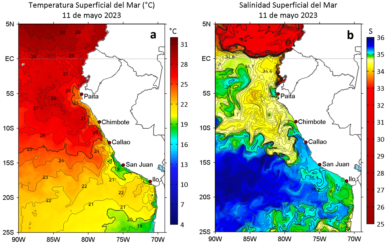
Figura 2. a) Temperatura superficial del mar ( ^{\circ}\text{C} ) y b) Salinidad superficial del mar para el 11 de mayo de 2023. Datos: OSTIA-UKMO-L4-GLOB-v2.0 (UK Met Office, 2012; Donlon et al, 2012) y del GLOBAL_ANALYSISFORECAST_PHY_001_024 (Lellouche, J. M. et al, 2013), respectivamente.
