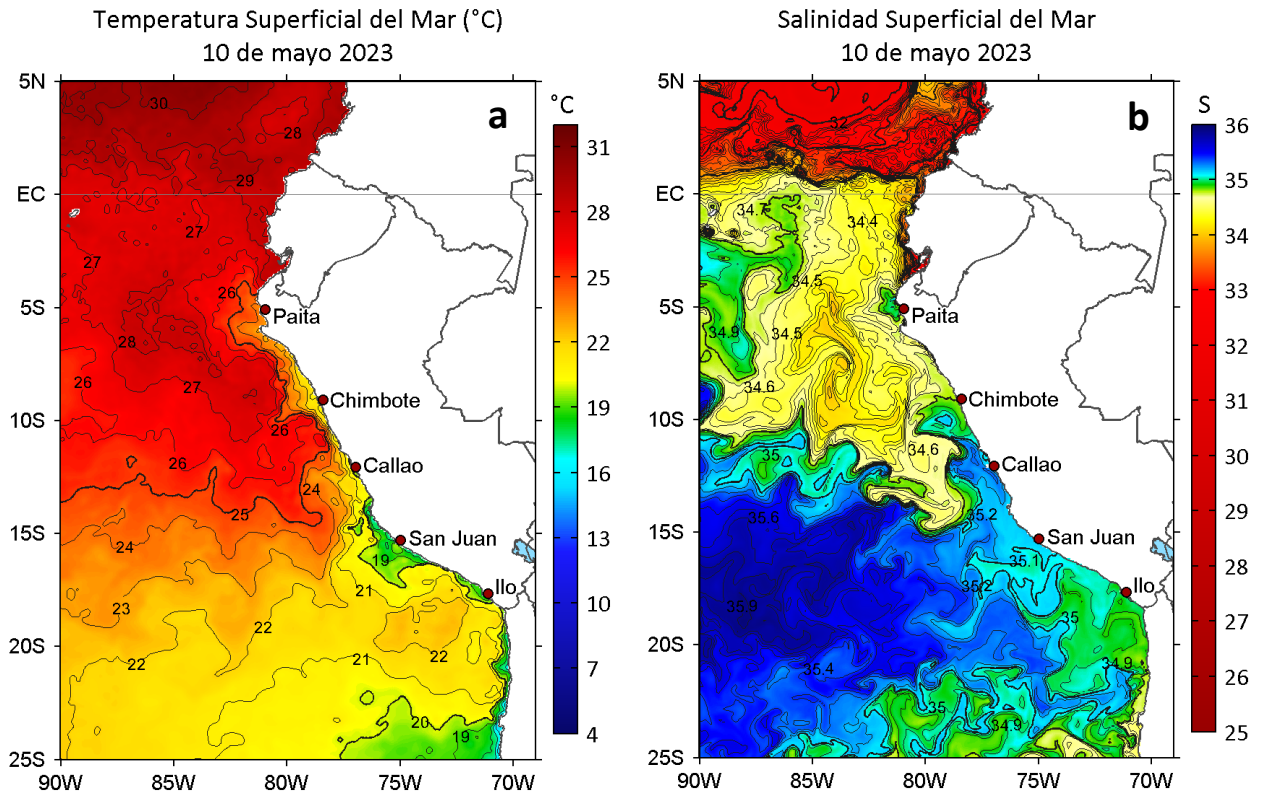
Figura 2. a) Temperatura superficial del mar (°C) y b) Salinidad superficial del mar para el 10 de mayo de 2023. Datos: OSTIA-UKMO-L4-GLOB-v2.0 (UK Met Office, 2012; Donlon et al, 2012) y del GLOBAL_ANALYSISFORECAST_PHY_001_024 (Lellouche, J. M. et al, 2013), respectivamente.
