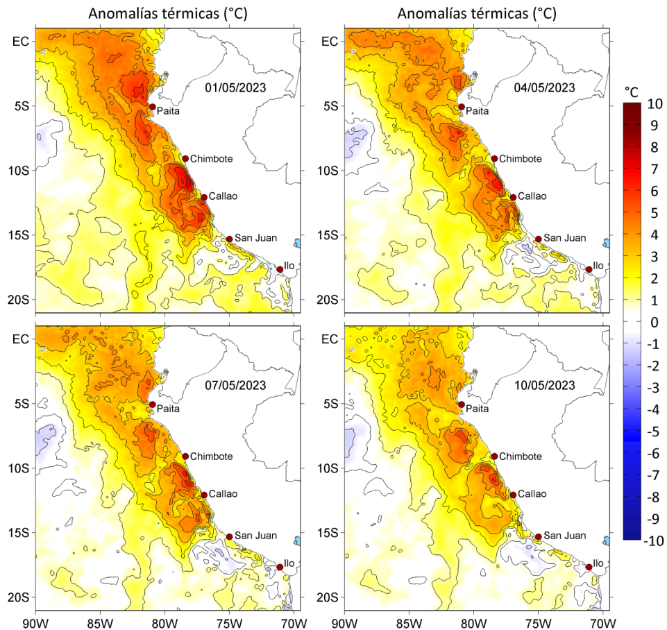
Figura 3. Anomalías de la temperatura superficial del mar (°C) para el a) 01, b) 04, c) 07 y d) 10 de mayo de 2023. Las anomalías se calcularon respecto de la climatología para el periodo 2007-2016. Datos: OSTIA-UKMO-L4-GLOB-v2.0 (UK Met Office, 2012; Donlon et al, 2012).
