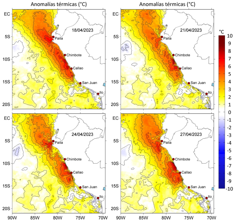
Figura 3. Anomalías de la temperatura superficial del mar (°C) para el a) 18, b) 21, c) 24 y d) 27 de abril de 2023. Las anomalías se calcularon respecto de la climatología para el periodo 2007-2016. Datos: OSTIA-UKMO-L4-GLOB-v2.0 (UK Met Office, 2012; Donlon et al, 2012).
