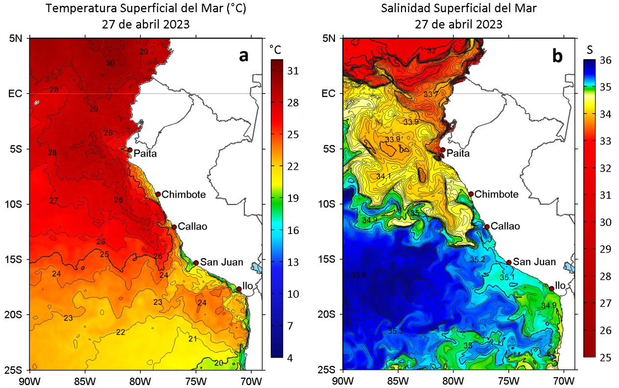
Figura 2. a) Temperatura superficial del mar (°C) y b) Salinidad superficial del mar para el 27 de abril de 2023, respectivamente. Datos: OSTIA-UKMO-L4-GLOB-v2.0 (UK Met Office, 2012; Donlon et al, 2012) y del GLOBAL_ANALYSIS_FORECAST_PHY_001_024 (Lellouche, J. M. et al, 2013), respectivamente.
