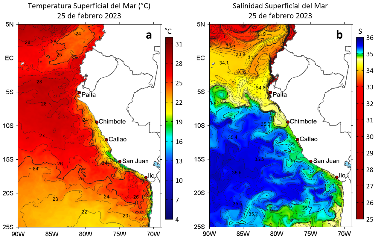
Figura 2. a) Temperatura superficial del mar (C) y b) Salinidad superficial del mar para el 25 de febrero de 2023. Datos: OSTIA-UKMO-L4-GLOB-v2.0 (UK Met Office, 2012; Donlon et al, 2012) y del GLOBAL_ANALYSIS_FORECAST_PHY_001_024 (Lellouche, J. M. et al, 2013), respectivamente.
