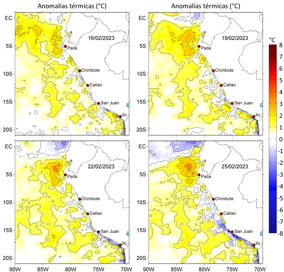
Figura 3. Anomalías de la temperatura superficial del mar (°C) para el a) 16, b) 19, c) 22 y d) 25 de febrero de 2023. Las anomalías se calcularon respecto de la climatología para el periodo 2007-2016. Datos: OSTIA-UKMO-L4-GLOB-v2.0 (UK Met Office, 2012; Donlon et al, 2012).
