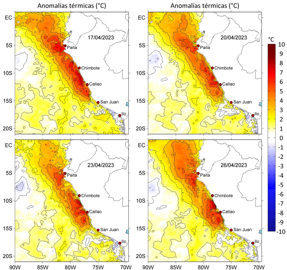
Figura 3. Anomalías de la temperatura superficial del mar (°C) para el a) 17, b) 20, c) 23 y d) 26 de abril de 2023. Las anomalías se calcularon respecto de la climatología para el periodo 2007-2016. Datos: OSTIA-UKMO-L4-GLOB-v2.0 (UK Met Office, 2012; Donlon et al, 2012).
