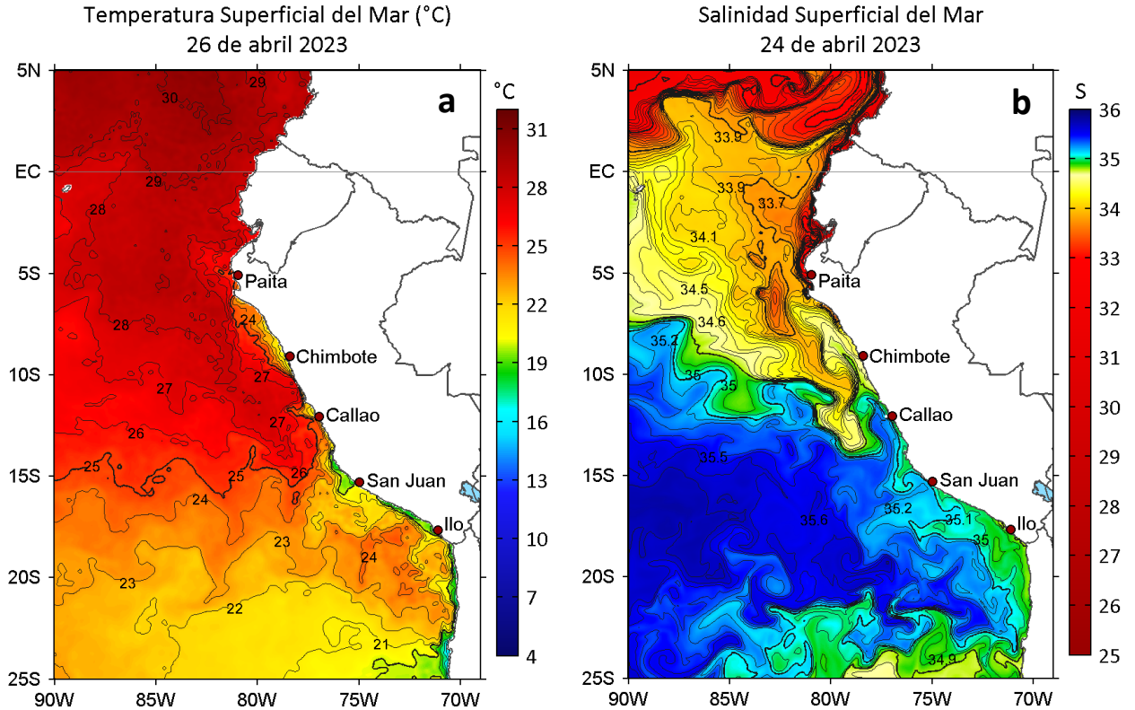
Figura 2. a) Temperatura superficial del mar (°C) y b) Salinidad superficial del mar para el 26 y 24 de abril de 2023, respectivamente. Datos: OSTIA-UKMO-L4-GLOB-v2.0 (UK Met Office, 2012; Donlon et al, 2012) y del GLOBAL_ANALYSIS_FORECAST_PHY_001_024 (Lellouche, J. M. et al, 2013), respectivamente.
