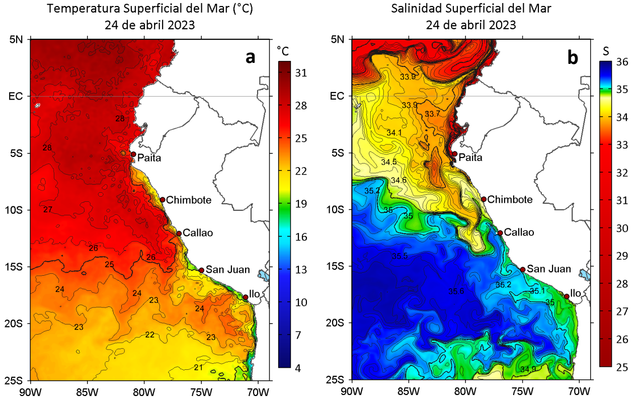
Figura 2. a) Temperatura superficial del mar ( ^{\circ}\text{C} ) y b) Salinidad superficial del mar para el 24 de abril de 2023. Datos: OSTIA-UKMO-L4-GLOB-v2.0 (UK Met Office, 2012; Donlon et al, 2012) y del GLOBAL_ANALYSIS_FORECAST_PHY_001_024 (Lellouche, J. M. et al, 2013), respectivamente.
