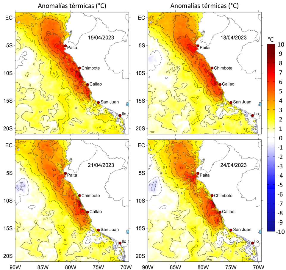
Figura 3. Anomalías de la temperatura superficial del mar ( ^{\circ}\text{C} ) para el a) 15, b) 18, c) 21 y d) 24 de abril de 2023. Las anomalías se calcularon respecto de la climatología para el periodo 2007-2016. Datos: OSTIA-UKMO-L4-GLOB-v2.0 (UK Met Office, 2012; Donlon et al, 2012).
