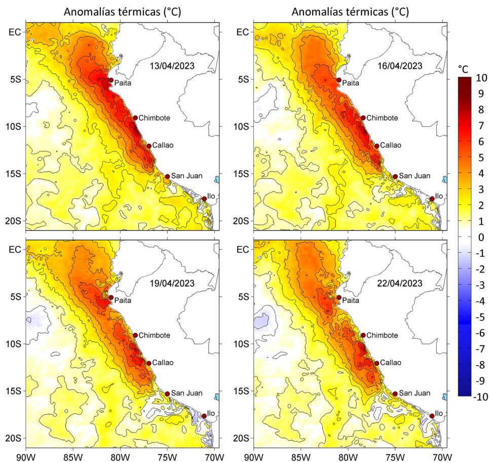
Figura 3. Anomalías de la temperatura superficial del mar ( ^{\circ}\text{C} ) para el a) 13, b) 16, c) 19 y d) 22 de abril de 2023. Las anomalías se calcularon respecto de la climatología para el periodo 2007-2016. Datos: OSTIA-UKMO-L4-GLOB-v2.0 (UK Met Office, 2012; Donlon et al, 2012).
