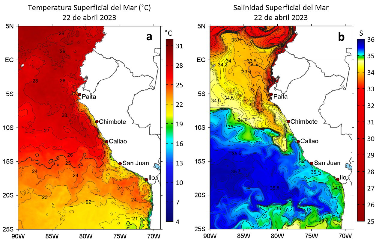
Figura 2. a) Temperatura superficial del mar ( ^{\circ}\text{C} ) y b) Salinidad superficial del mar para el 22 de abril de 2023. Datos: OSTIA-UKMO-L4-GLOB-v2.0 (UK Met Office, 2012; Donlon et al, 2012) y del GLOBAL_ANALYSIS_FORECAST_PHY_001_024 (Lellouche, J. M. et al, 2013), respectivamente.
