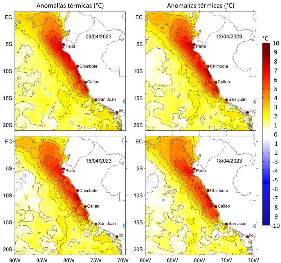
Figura 3. Anomalías de la temperatura superficial del mar ( ^{\circ}\text{C} ) para el a) 09, b) 12, c) 15 y d) 18 de abril de 2023. Las anomalías se calcularon respecto de la climatología para el periodo 2007-2016. Datos: OSTIA-UKMO-L4-GLOB-v2.0 (UK Met Office, 2012; Donlon et al, 2012).
