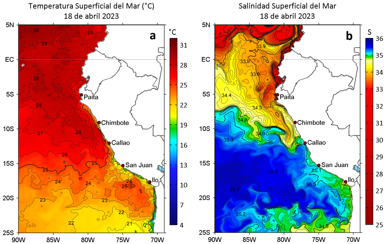
Figura 2. a) Temperatura superficial del mar ( ^{\circ}\text{C} ) y b) Salinidad superficial del mar para el 18 de abril de 2023. Datos: OSTIA-UKMO-L4-GLOB-v2.0 (UK Met Office, 2012; Donlon et al, 2012) y del GLOBAL_ANALYSIS_FORECAST_PHY_001_024 (Lellouche, J. M. et al, 2013), respectivamente.
