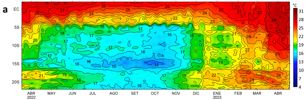
Anomalías de la Temperatura Superficial del mar (°C), franja costera de 60 m.n. 18 de marzo 2022 - 18 de abril 2023
