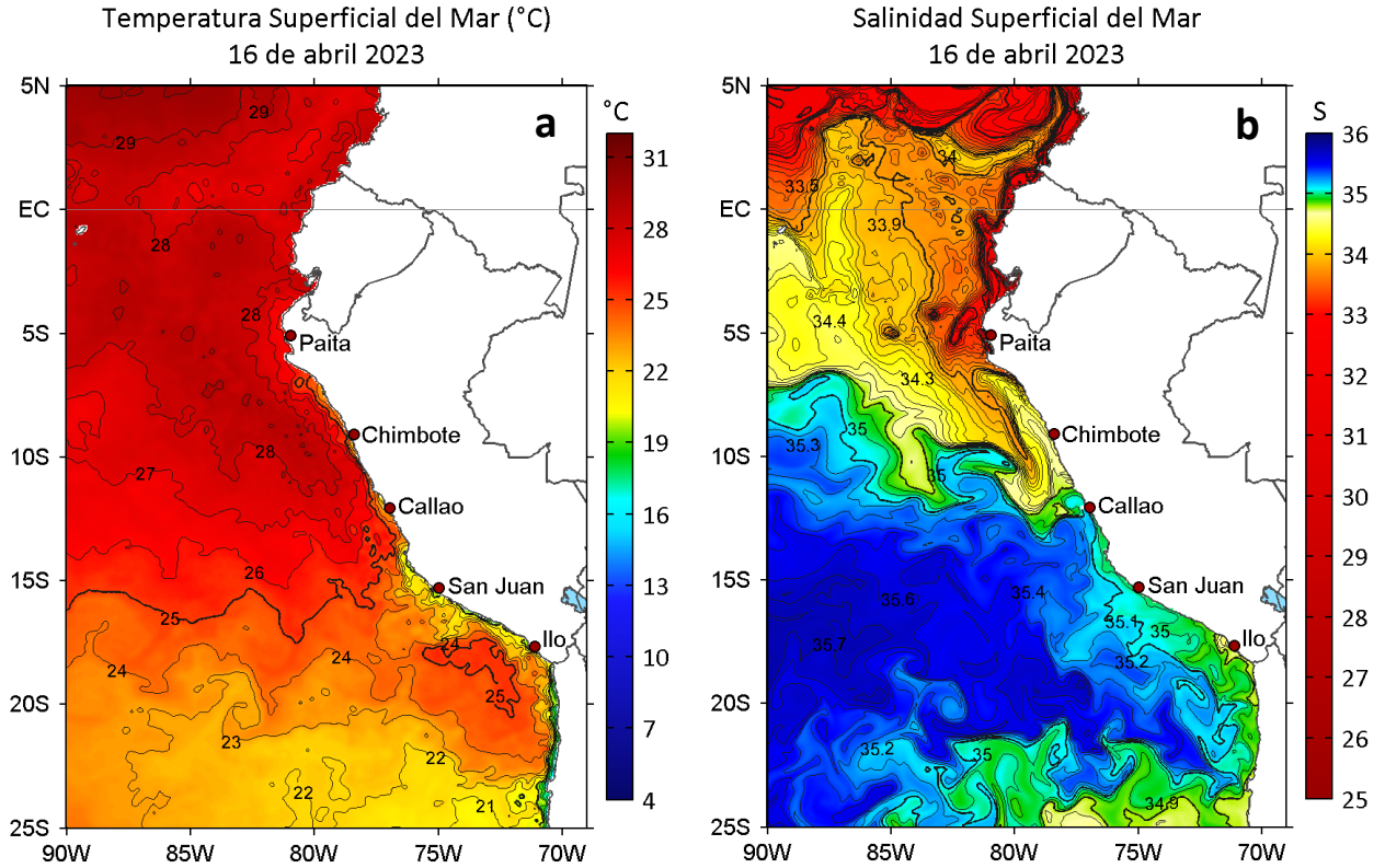
Figura 2. a) Temperatura superficial del mar ( ^{\circ}\text{C} ) y b) Salinidad superficial del mar para el 16 de abril de 2023. Datos: OSTIA-UKMO-L4-GLOB-v2.0 (UK Met Office, 2012; Donlon et al, 2012) y del GLOBAL_ANALYSIS_FORECAST_PHY_001_024 (Lellouche, J. M. et al, 2013), respectivamente.
