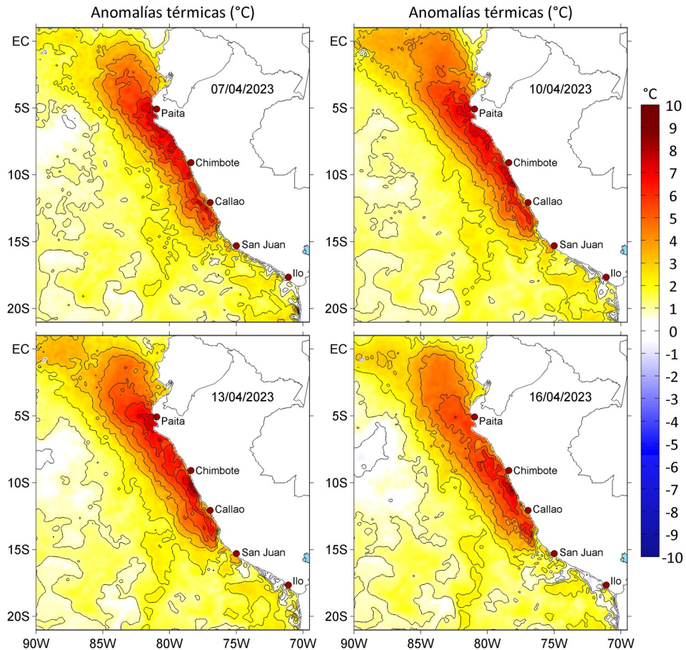
Figura 3. Anomalías de la temperatura superficial del mar ( ^{\circ}\text{C} ) para el a) 07, b) 10, c) 13 y d) 16 de abril de 2023. Las anomalías se calcularon respecto de la climatología para el periodo 2007-2016. Datos: OSTIA-UKMO-L4-GLOB-v2.0 (UK Met Office, 2012; Donlon et al, 2012).
