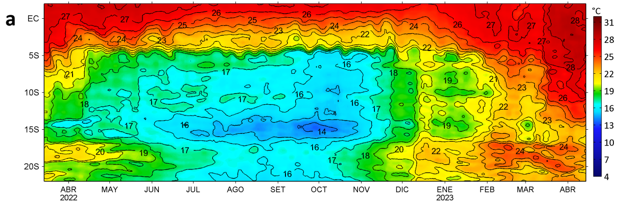
Anomalías de la Temperatura Superficial del mar (°C), franja costera de 60 m.n. 14 de marzo 2022 - 14 de abril 2023
