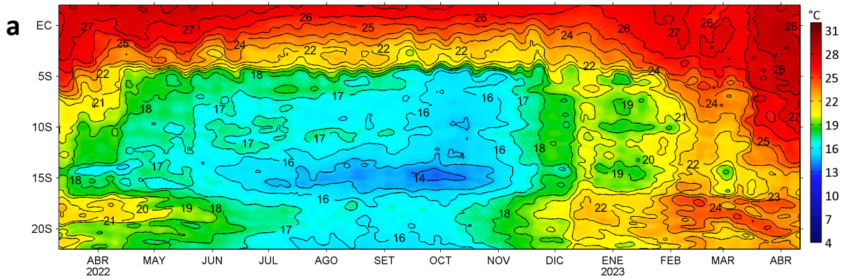
Anomalías de la Temperatura Superficial del mar (°C), franja costera de 60 m.n. 11 de marzo 2022 - 11 de abril 2023
