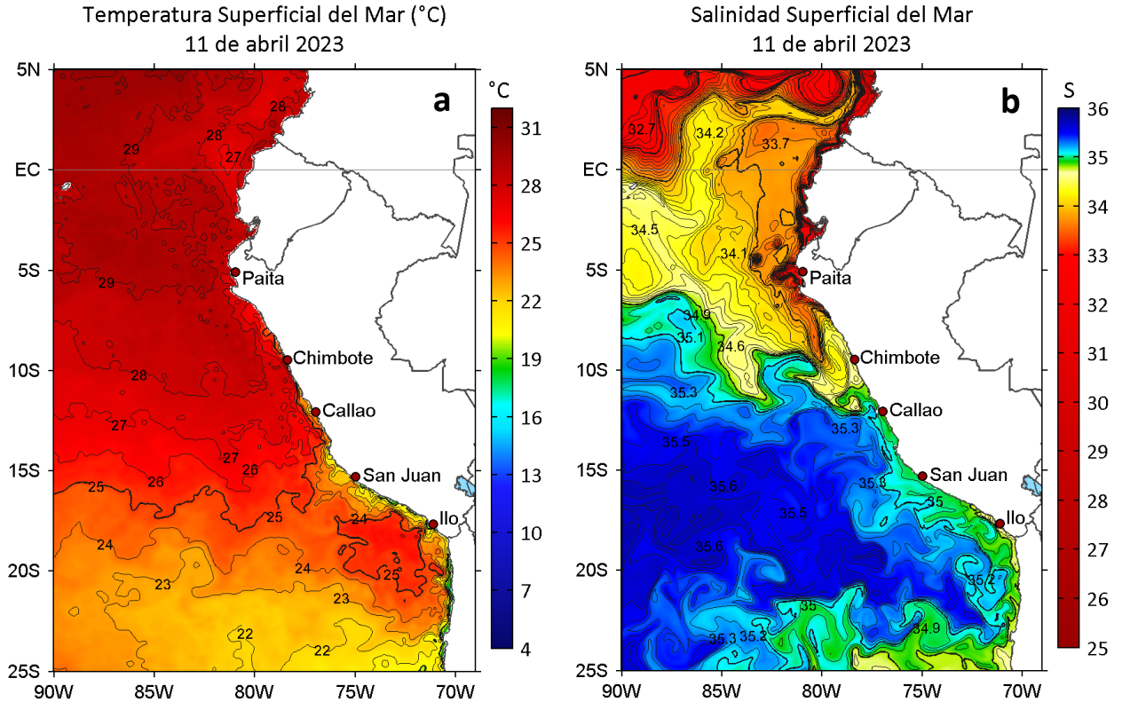
Figura 2. a) Temperatura superficial del mar ( ^{\circ}\text{C} ) y b) Salinidad superficial del mar para el 11 de abril de 2023. Datos: OSTIA-UKMO-L4-GLOB-v2.0 (UK Met Office, 2012; Donlon et al, 2012) y del GLOBAL_ANALYSIS_FORECAST_PHY_001_024 (Lellouche, J. M. et al, 2013), respectivamente.
