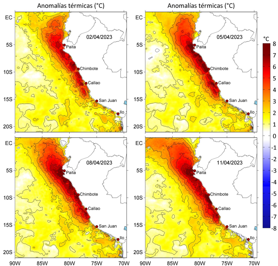
Figura 3. Anomalías de la temperatura superficial del mar ( ^{\circ}\text{C} ) para el a) 02, b) 05, c) 08 y d) 11 de abril de 2023. Las anomalías se calcularon respecto de la climatología para el periodo 2007-2016. Datos: OSTIA-UKMO-L4-GLOB-v2.0 (UK Met Office, 2012; Donlon et al, 2012).
