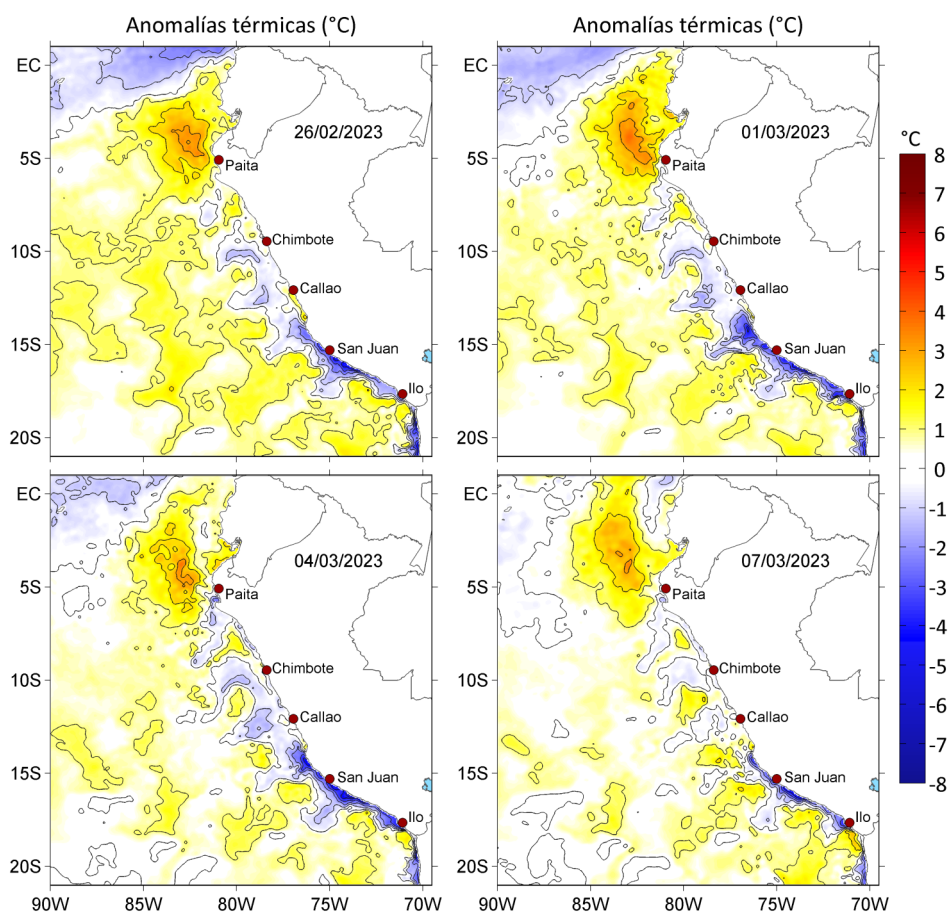
Figura 3. Anomalías de la temperatura superficial del mar ( ^{\circ}\text{C} ) para el a) 26 de febrero, b) 01, c) 04 y d) 07 de marzo de 2023. Las anomalías se calcularon respecto de la climatología para el periodo 2007-2016. Datos: OSTIA-UKMO-L4-GLOB-v2.0 (UK Met Office, 2012; Donlon et al, 2012).
