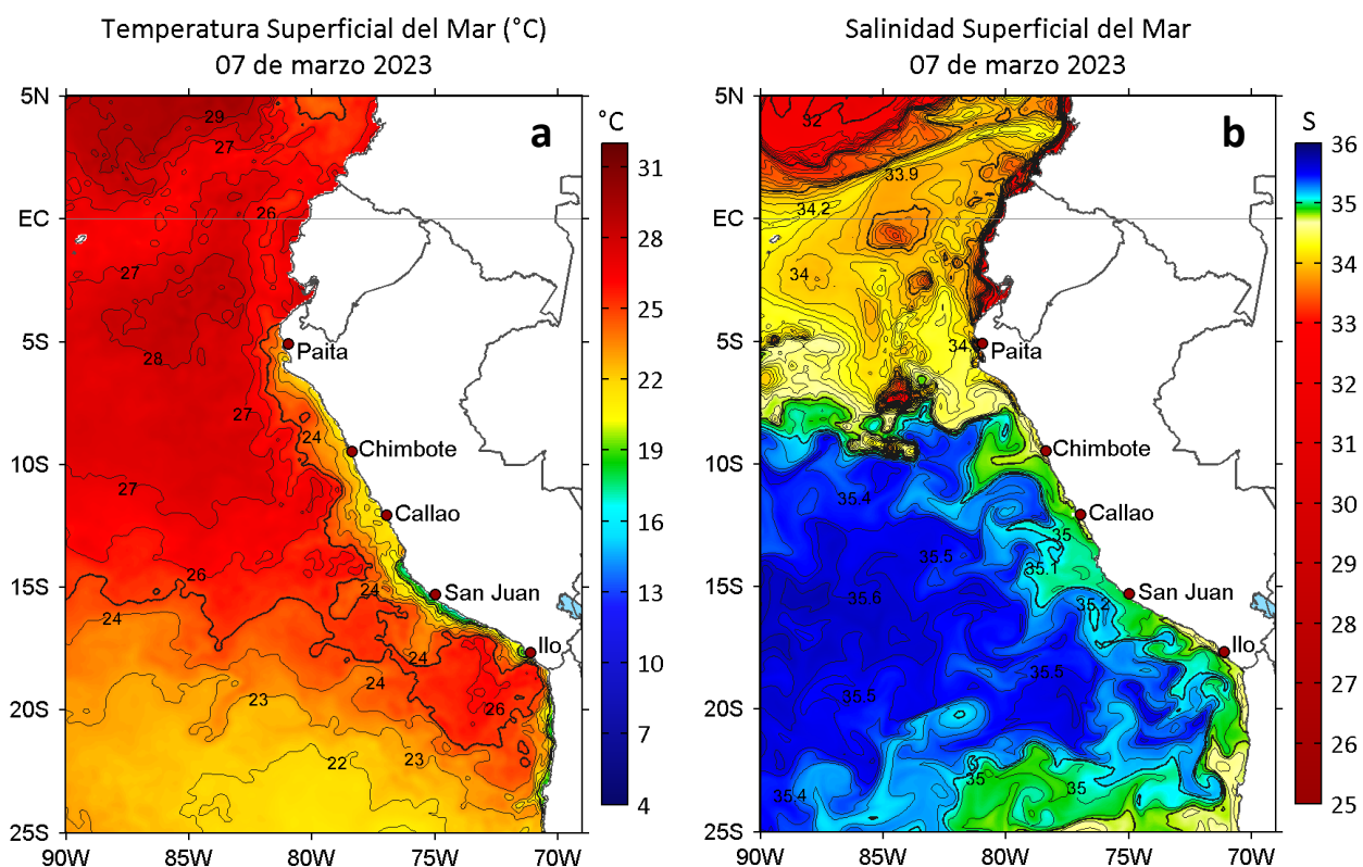
Figura 2. a) Temperatura superficial del mar ( ^{\circ}\text{C} ) y b) Salinidad superficial del mar para el 07 de marzo de 2023. Datos: OSTIA-UKMO-L4-GLOB-v2.0 (UK Met Office, 2012; Donlon et al, 2012) y del GLOBAL_ANALYSIS_FORECAST_PHY_001_024 (Lellouche, J. M. et al, 2013), respectivamente.
