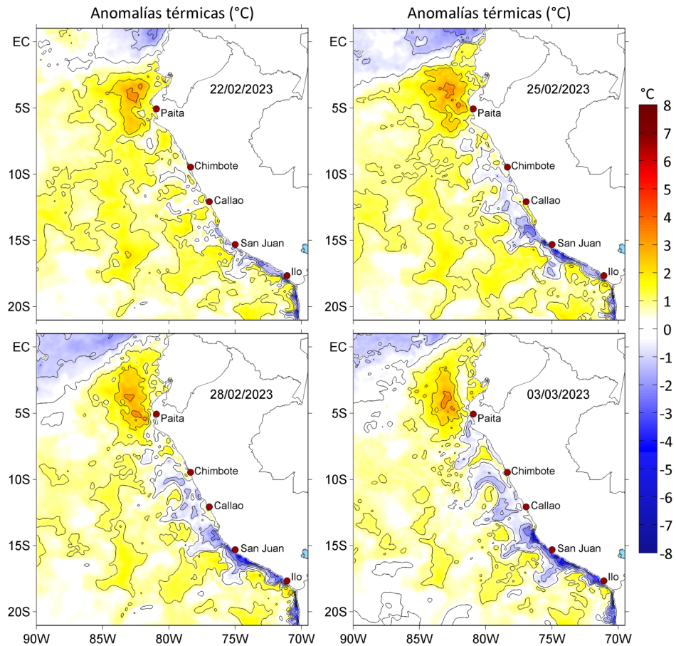
Figura 3. Anomalías de la temperatura superficial del mar ( ^{\circ}\text{C} ) para el a) 22, b) 25 y c) 28 de febrero, así como para el d) 03 de marzo de 2023. Las anomalías se calcularon respecto de la climatología para el periodo 2007-2016. Datos: OSTIA-UKMO-L4-GLOB-v2.0 (UK Met Office, 2012; Donlon et al, 2012).
