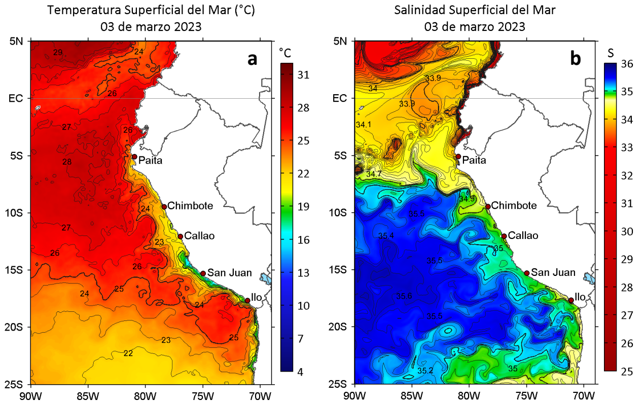
Figura 2. a) Temperatura superficial del mar ( ^{\circ}\text{C} ) y b) Salinidad superficial del mar para el 03 de marzo de 2023. Datos: OSTIA-UKMO-L4-GLOB-v2.0 (UK Met Office, 2012; Donlon et al, 2012) y del GLOBAL_ANALYSIS_FORECAST_PHY_001_024 (Lellouche, J. M. et al, 2013), respectivamente.
