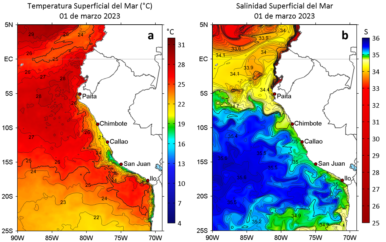
Figura 2. a) Temperatura superficial del mar ( ^{\circ}\text{C} ) y b) Salinidad superficial del mar para el 01 de marzo de 2023. Datos: OSTIA-UKMO-L4-GLOB-v2.0 (UK Met Office, 2012; Donlon et al, 2012) y del GLOBAL_ANALYSIS_FORECAST_PHY_001_024 (Lellouche, J. M. et al, 2013), respectivamente.
