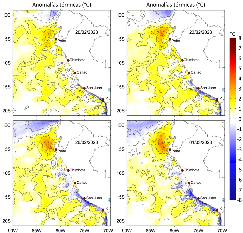
Figura 3. Anomalías de la temperatura superficial del mar ( ^{\circ}\text{C} ) para el a) 20, b) 23 y c) 26 de febrero, así como para el d) 01 de marzo de 2023. Las anomalías se calcularon respecto de la climatología para el periodo 2007-2016. Datos: OSTIA-UKMO-L4-GLOB-v2.0 (UK Met Office, 2012; Donlon et al, 2012).
