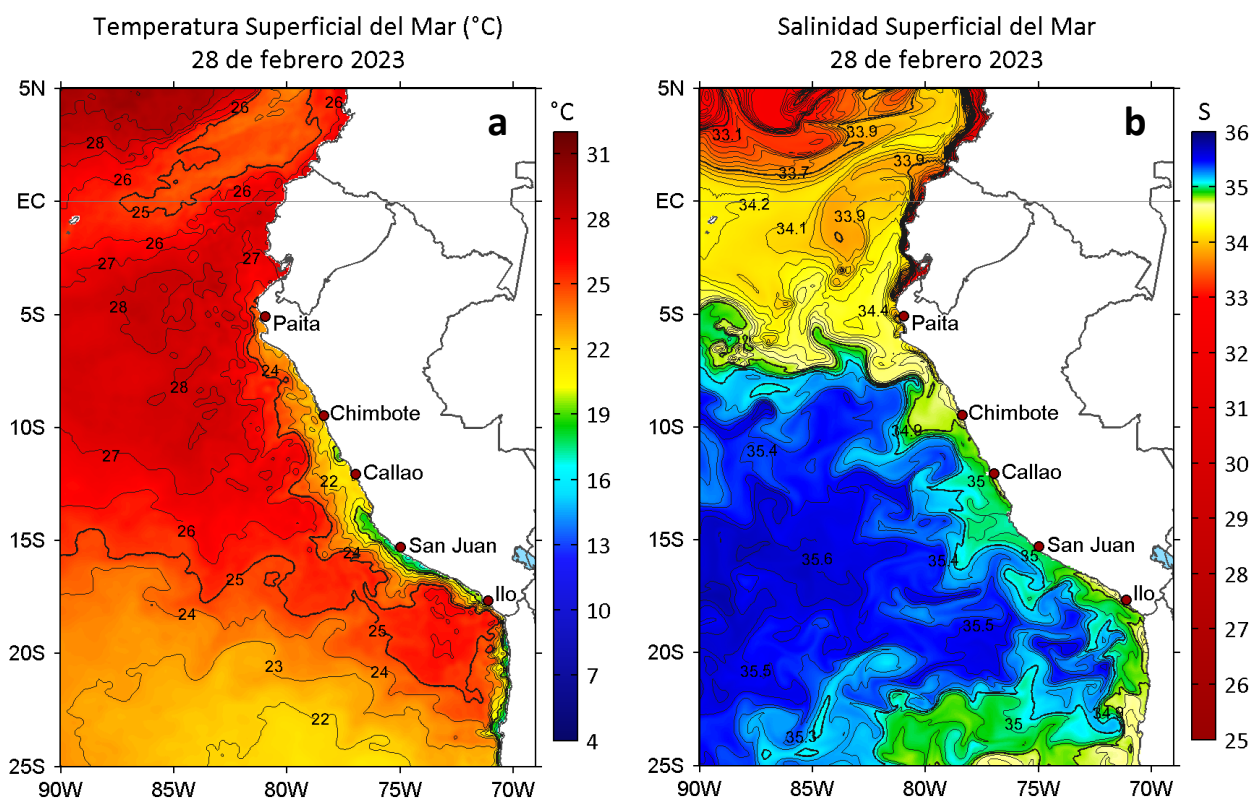
Figura 2. a) Temperatura superficial del mar ( ^{\circ}\text{C} ) y b) Salinidad superficial del mar para el 28 de febrero de 2023. Datos: OSTIA-UKMO-L4-GLOB-v2.0 (UK Met Office, 2012; Donlon et al, 2012) y del GLOBAL_ANALYSIS_FORECAST_PHY_001_024 (Lellouche, J. M. et al, 2013), respectivamente.
