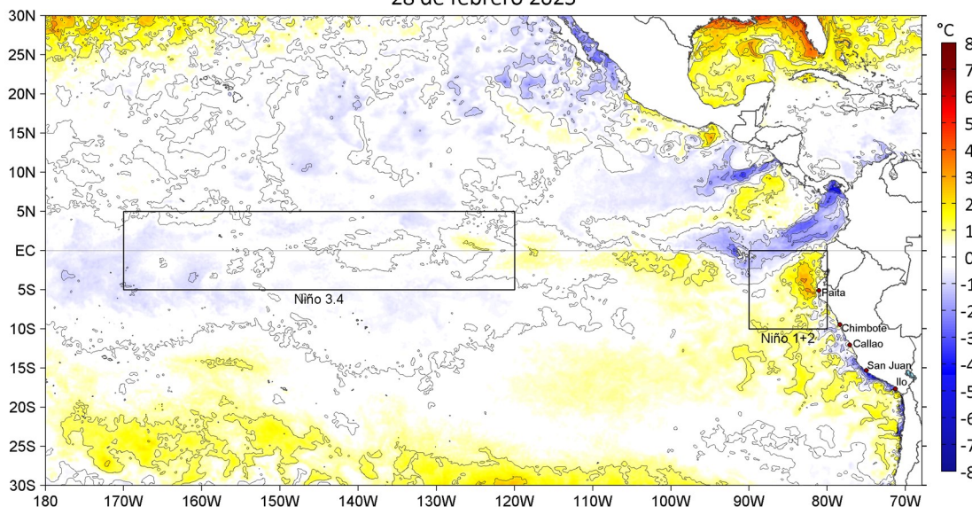
Figura 1. Anomalías de la temperatura superficial del mar (°C) en el océano Pacífico tropical. Las regiones Niño 3.4 (5°N-5°S, 170° W-120°W) y Niño 1+2 (0°-10°S, 90°W-80°W) están delimitadas con una línea de color negro. Las anomalías se estimaron de acuerdo a la climatología para el periodo 2007-2016. Los datos provienen de OSTIA-UKMO-L4-GLOB-v2.0 (UK Met Office, 2012; Donlon et al, 2012) disponibles en https://podaac.jpl.nasa.gov/dataset/OSTIA-UKMO-L4-GLOB-v2.0 .
