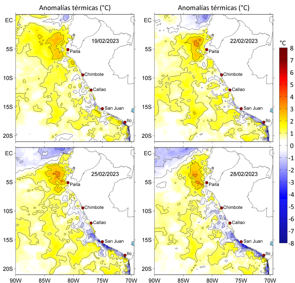
Figura 3. Anomalías de la temperatura superficial del mar ( ^{\circ}\text{C} ) para el a) 19, b) 22, c) 25 y d) 28 de febrero de 2023. Las anomalías se calcularon respecto de la climatología para el periodo 2007-2016. Datos: OSTIA-UKMO-L4-GLOB-v2.0 (UK Met Office, 2012; Donlon et al, 2012).
