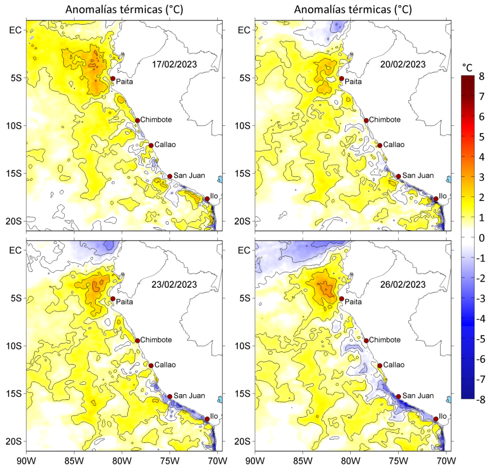
Figura 3. Anomalías de la temperatura superficial del mar (°C) para el a) 17, b) 20, c) 23 y d) 26 de febrero de 2023. Las anomalías se calcularon respecto de la climatología para el periodo 2007-2016. Datos: OSTIA-UKMO-L4-GLOB-v2.0 (UK Met Office, 2012; Donlon et al, 2012).
