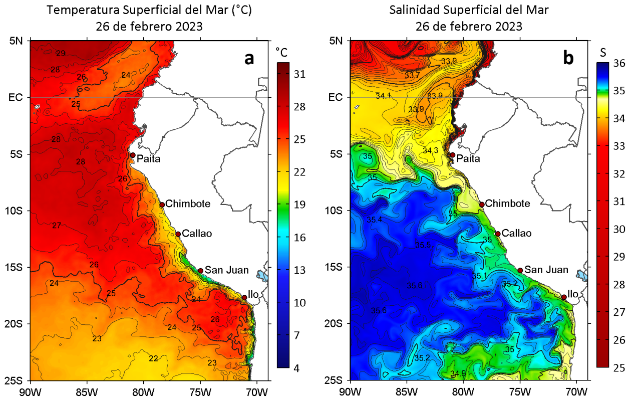
Figura 2. a) Temperatura superficial del mar (C) y b) Salinidad superficial del mar para el 26 de febrero de 2023. Datos: OSTIA-UKMO-L4-GLOB-v2.0 (UK Met Office, 2012; Donlon et al, 2012) y del GLOBAL_ANALYSIS_FORECAST_PHY_001_024 (Lellouche, J. M. et al, 2013), respectivamente.
