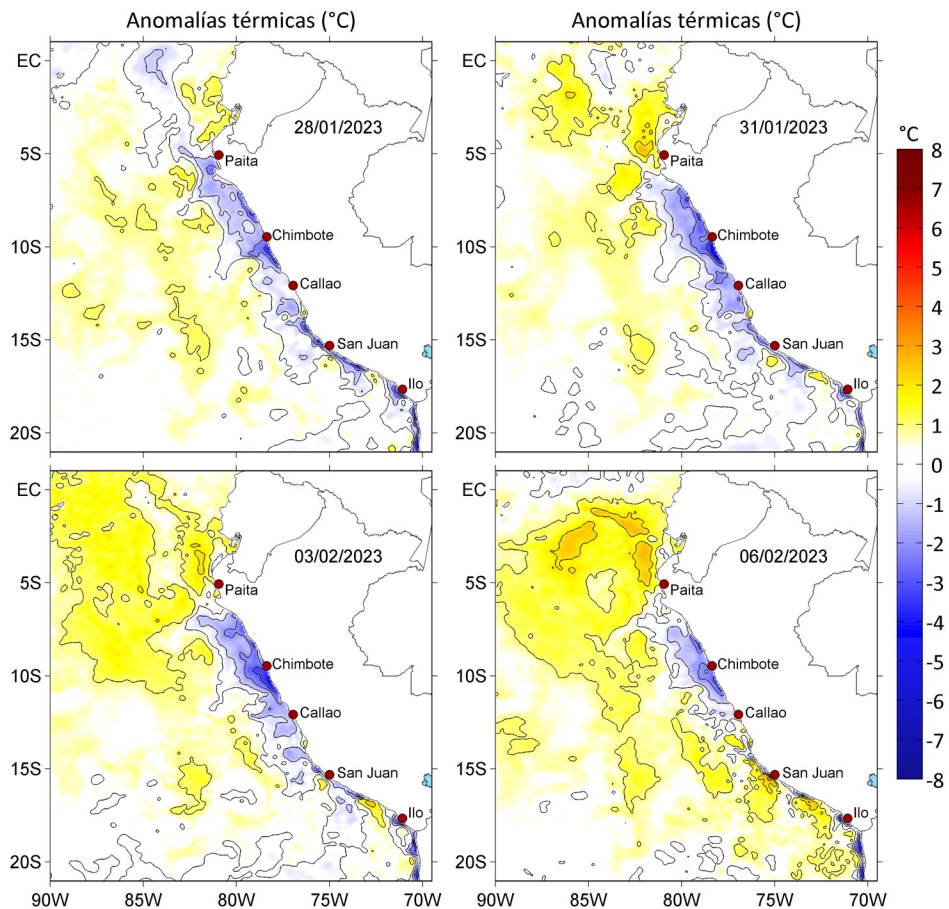
Figura 3. Anomalías de la temperatura superficial del mar (°C) para el a) 28 y b) 31 de enero, así como para el c) 03 y d) 06 de febrero de 2023. Las anomalías se calcularon respecto de la climatología para el periodo 2007-2016. Datos: OSTIA-UKMO-L4-GLOB-v2.0 (UK Met Office, 2012; Donlon et al, 2012).
