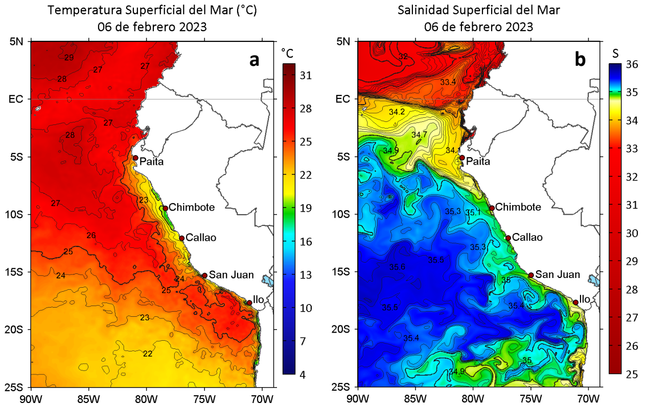
Figura 2. a) Temperatura superficial del mar (C) y b) Salinidad superficial del mar para el 06 de febrero de 2023. Datos: OSTIA-UKMO-L4-GLOB-v2.0 (UK Met Office, 2012; Donlon et al, 2012) y del GLOBAL_ANALYSIS_FORECAST_PHY_001_024 (Lellouche, J. M. et al, 2013), respectivamente.
