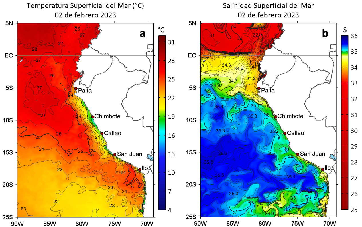
Figura 2. a) Temperatura superficial del mar (C) y b) Salinidad superficial del mar para el 02 de febrero de 2023. Datos: OSTIA-UKMO-L4-GLOB-v2.0 (UK Met Office, 2012; Donlon et al, 2012) y del GLOBAL_ANALYSIS_FORECAST_PHY_001_024 (Lellouche, J. M. et al, 2013), respectivamente.
