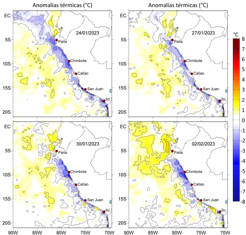
Figura 3. Anomalías de la temperatura superficial del mar (°C) para el a) 24, b) 27 y c) 30 de enero, así como para el d) 02 de febrero de 2023. Las anomalías se calcularon respecto de la climatología para el periodo 2007-2016. Datos: OSTIA-UKMO-L4-GLOB-v2.0 (UK Met Office, 2012; Donlon et al, 2012).
