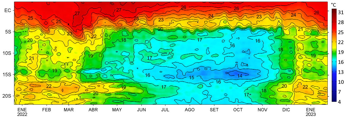
Anomalías de la Temperatura Superficial del mar (°C), franja costera de 60 m.n. 22 de diciembre 2021 - 22 de enero 2023
