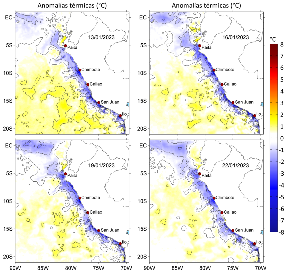
Figura 3. Anomalías de la temperatura superficial del mar (°C) para el a) 13, b) 16, c) 19 y d) 22 de enero de 2023. Las anomalías se calcularon respecto de la climatología para el periodo 2007-2016. Datos: OSTIA-UKMO-L4-GLOB-v2.0 (UK Met Office, 2012; Donlon et al, 2012).
