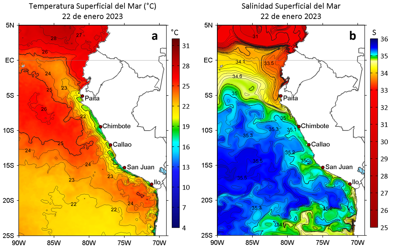
Figura 2. a) Temperatura superficial del mar (°C) y b) Salinidad superficial del mar para el 22 de enero de 2023. Datos: OSTIA-UKMO-L4-GLOB-v2.0 (UK Met Office, 2012; Donlon et al, 2012) y del GLOBAL_ANALYSIS_FORECAST_PHY_001_024 (Lellouche, J. M. et al, 2013), respectivamente.
