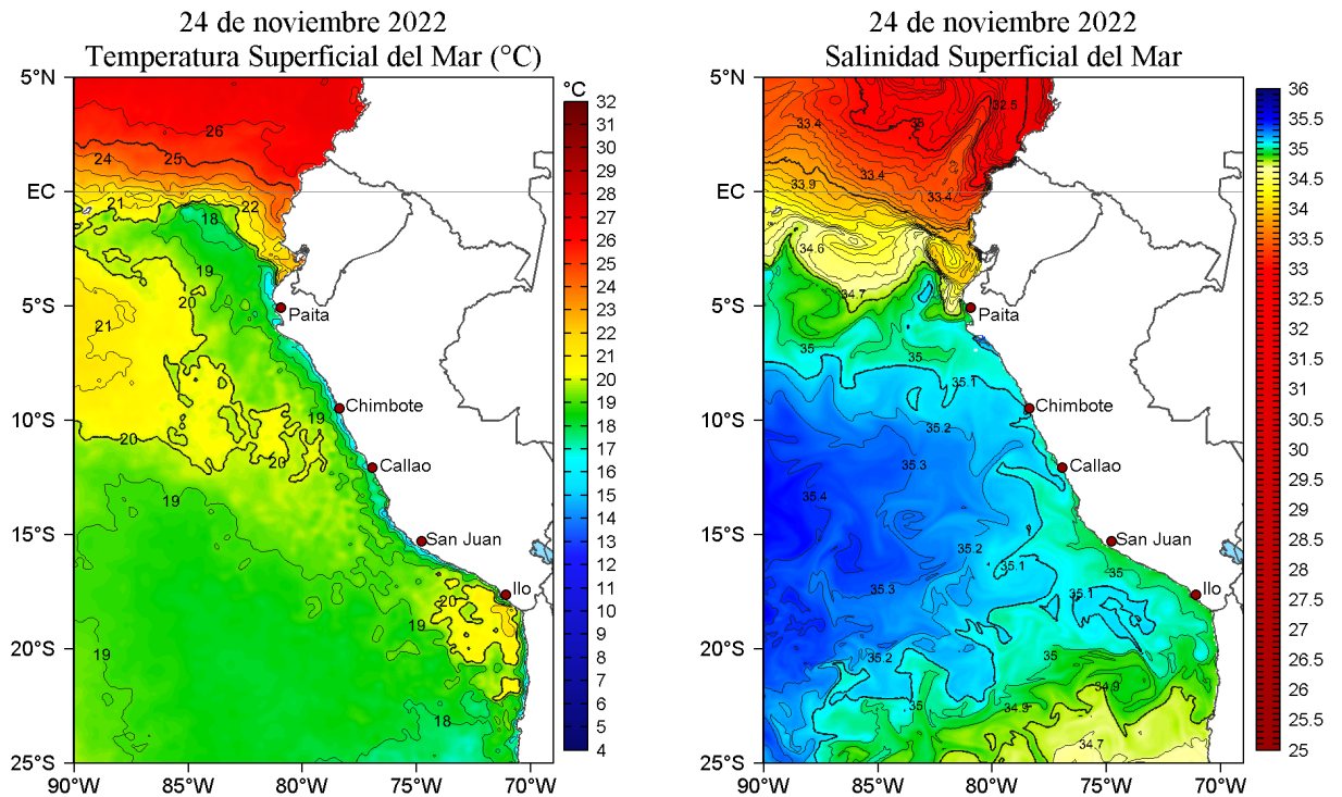
Figura 2. Temperatura superficial del mar (a la izquierda) y Salinidad superficial del mar (a la derecha) para el 24 de noviembre de 2022. Datos: OSTIA-UKMO-L4-GLOB-v2.0 (UK Met Office, 2012; Donlon et al, 2012) y Hybrid Coordinate Ocean Model v. GOFS 3.1 (HYCOM; Halliwell et al., 1998; 2000; Bleck, 2001), respectivamente.
