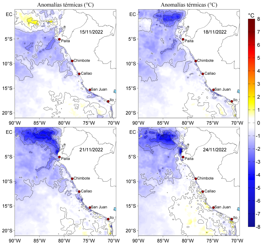
Figura 3. Anomalías de la temperatura superficial del mar (°C) para el 15, 18, 21 y 24 de noviembre de 2022. Las anomalías se calcularon respecto de la climatología para el periodo 2007-2016. Datos: OSTIA-UKMO-L4-GLOB-v2.0 (UK Met Office, 2012; Donlon et al, 2012).
