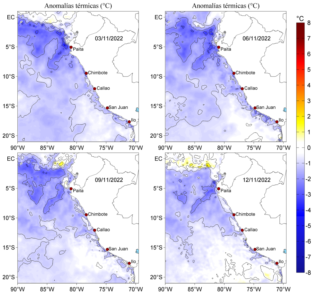
Figura 3. Anomalías de la temperatura superficial del mar ( ^{\circ}\text{C} ) para el 03, 06, 09 y 12 de noviembre de 2022. Las anomalías se calcularon respecto de la climatología para el periodo 2007-2016. Datos: OSTIA-UKMO-L4-GLOB-v2.0 (UK Met Office, 2012; Donlon et al, 2012).
