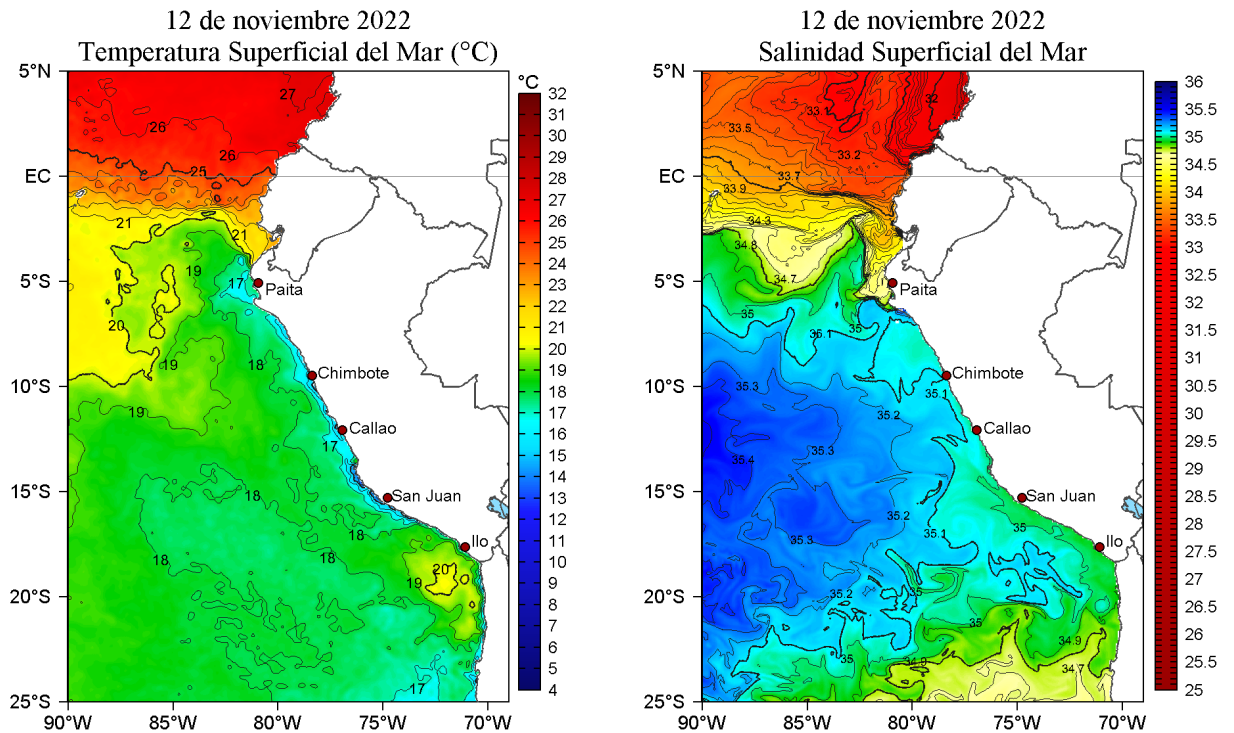
Figura 2. Temperatura superficial del mar (a la izquierda) y Salinidad superficial del mar (a la derecha) para el 12 de noviembre de 2022. Datos: OSTIA-UKMO-L4-GLOB-v2.0 (UK Met Office, 2012; Donlon et al, 2012) y Hybrid Coordinate Ocean Model v. GOFS 3.1 (HYCOM; Halliwell et al., 1998; 2000; Bleck, 2001), respectivamente.
