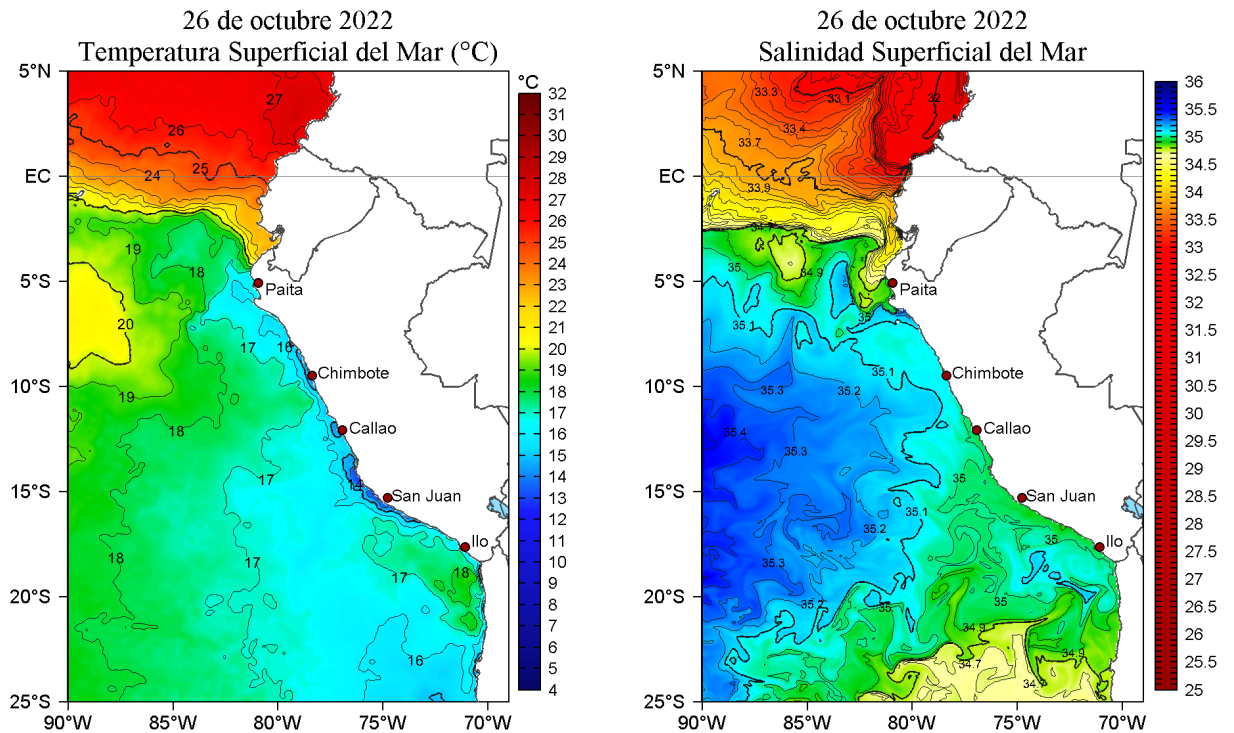
Figura 2. Temperatura superficial del mar (a la izquierda) y Salinidad superficial del mar (a la derecha) para el 26 de octubre de 2022. Datos: OSTIA-UKMO-L4-GLOB-v2.0 (UK Met Office, 2012; Donlon et al, 2012) y Hybrid Coordinate Ocean Model v. GOFS 3.1 (HYCOM; Halliwell et al., 1998; 2000; Bleck, 2001), respectivamente.
