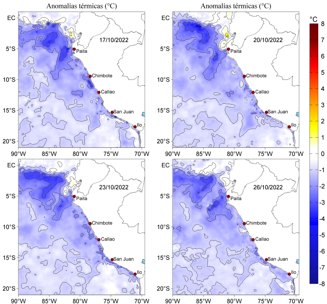
Figura 3. Anomalías de la temperatura superficial del mar ( ^{\circ}\text{C} ) para el 17, 20, 23 y 26 de octubre de 2022. Las anomalías se calcularon respecto de la climatología para el periodo 2007-2016. Datos: OSTIA-UKMO-L4-GLOB-v2.0 (UK Met Office, 2012; Donlon et al, 2012).
