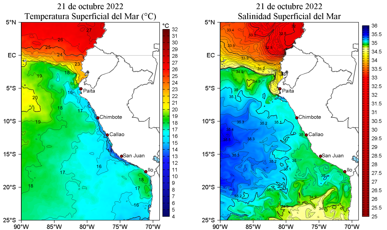
Figura 2. Temperatura superficial del mar (a la izquierda) y Salinidad superficial del mar (a la derecha) para el 21 de octubre de 2022. Datos: OSTIA-UKMO-L4-GLOB-v2.0 (UK Met Office, 2012; Donlon et al, 2012) y Hybrid Coordinate Ocean Model v. GOFS 3.1 (HYCOM; Halliwell et al., 1998; 2000; Bleck, 2001), respectivamente.
