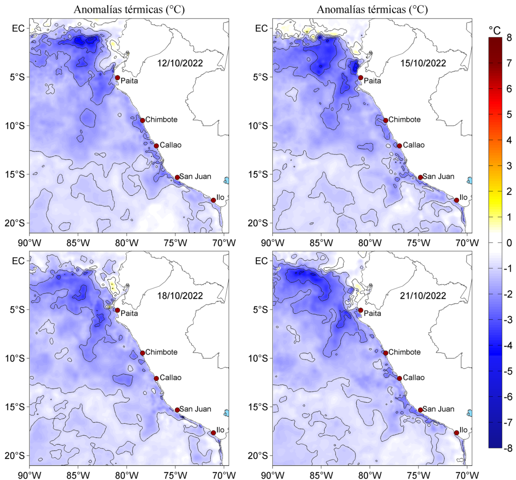
Figura 3. Anomalías de la temperatura superficial del mar (°C) para el 12, 15, 18 y 21 de octubre de 2022. Las anomalías se calcularon respecto de la climatología para el periodo 2007-2016. Datos: OSTIA-UKMO-L4-GLOB-v2.0 (UK Met Office, 2012; Donlon et al, 2012).
