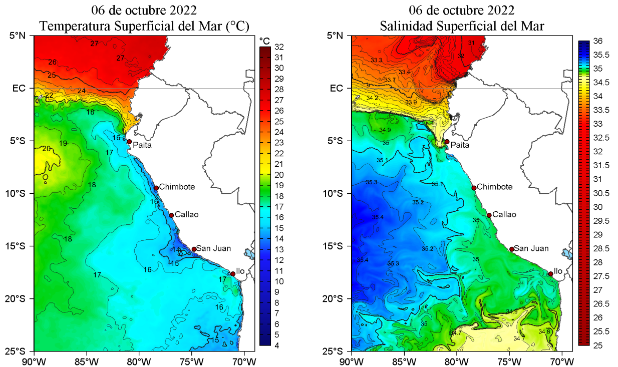
Figura 2. Temperatura superficial del mar (a la izquierda) y Salinidad superficial del mar (a la derecha) para el 06 de octubre de 2022. Datos: OSTIA-UKMO-L4-GLOB-v2.0 (UK Met Office, 2012; Donlon et al, 2012) y Hybrid Coordinate Ocean Model v. GOFS 3.1 (HYCOM; Halliwell et al., 1998; 2000; Bleck, 2001), respectivamente.
