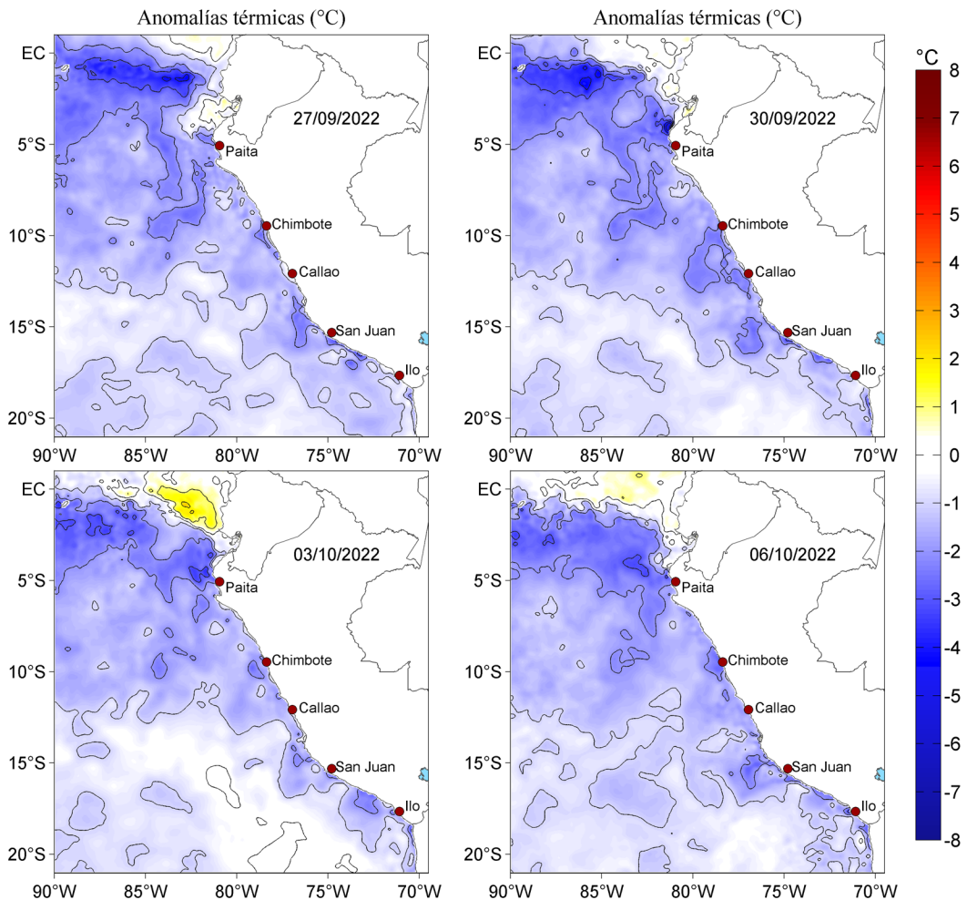
Figura 3. Anomalías de la temperatura superficial del mar (°C) para el 27 y 30 de setiembre, así como para el 03 y 06 de octubre de 2022. Las anomalías se calcularon respecto de la climatología para el periodo 2007-2016. Datos: OSTIA-UKMO-L4-GLOB-v2.0 (UK Met Office, 2012; Donlon et al, 2012).
