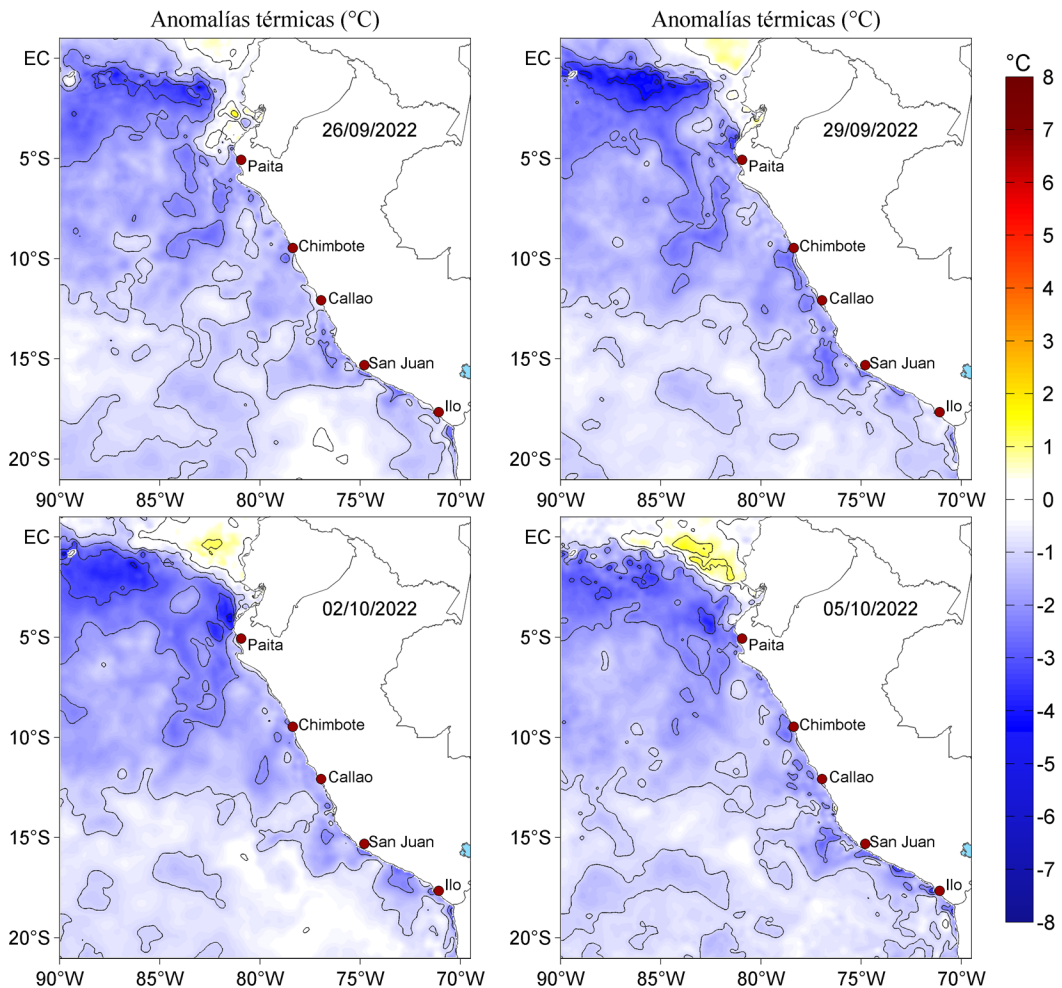
Figura 3. Anomalías de la temperatura superficial del mar (°C) para el 26 y 29 de setiembre, así como para el 02 y 05 de octubre de 2022. Las anomalías se calcularon respecto de la climatología para el periodo 2007-2016. Datos: OSTIA-UKMO-L4-GLOB-v2.0 (UK Met Office, 2012; Donlon et al, 2012).
