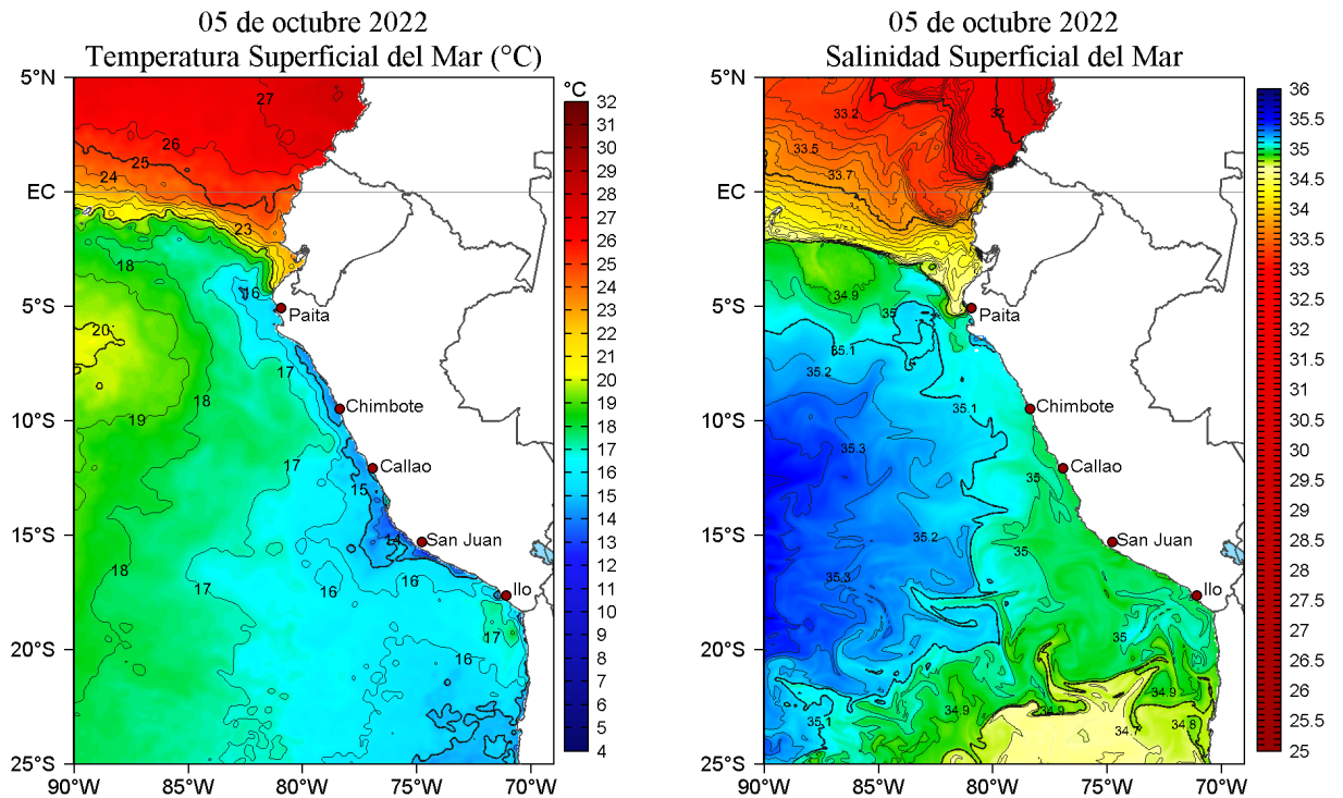
Figura 2. Temperatura superficial del mar (a la izquierda) y Salinidad superficial del mar (a la derecha) para el 05 de octubre de 2022. Datos: OSTIA-UKMO-L4-GLOB-v2.0 (UK Met Office, 2012; Donlon et al, 2012) y Hybrid Coordinate Ocean Model v. GOFS 3.1 (HYCOM; Halliwell et al., 1998; 2000; Bleck, 2001), respectivamente.
