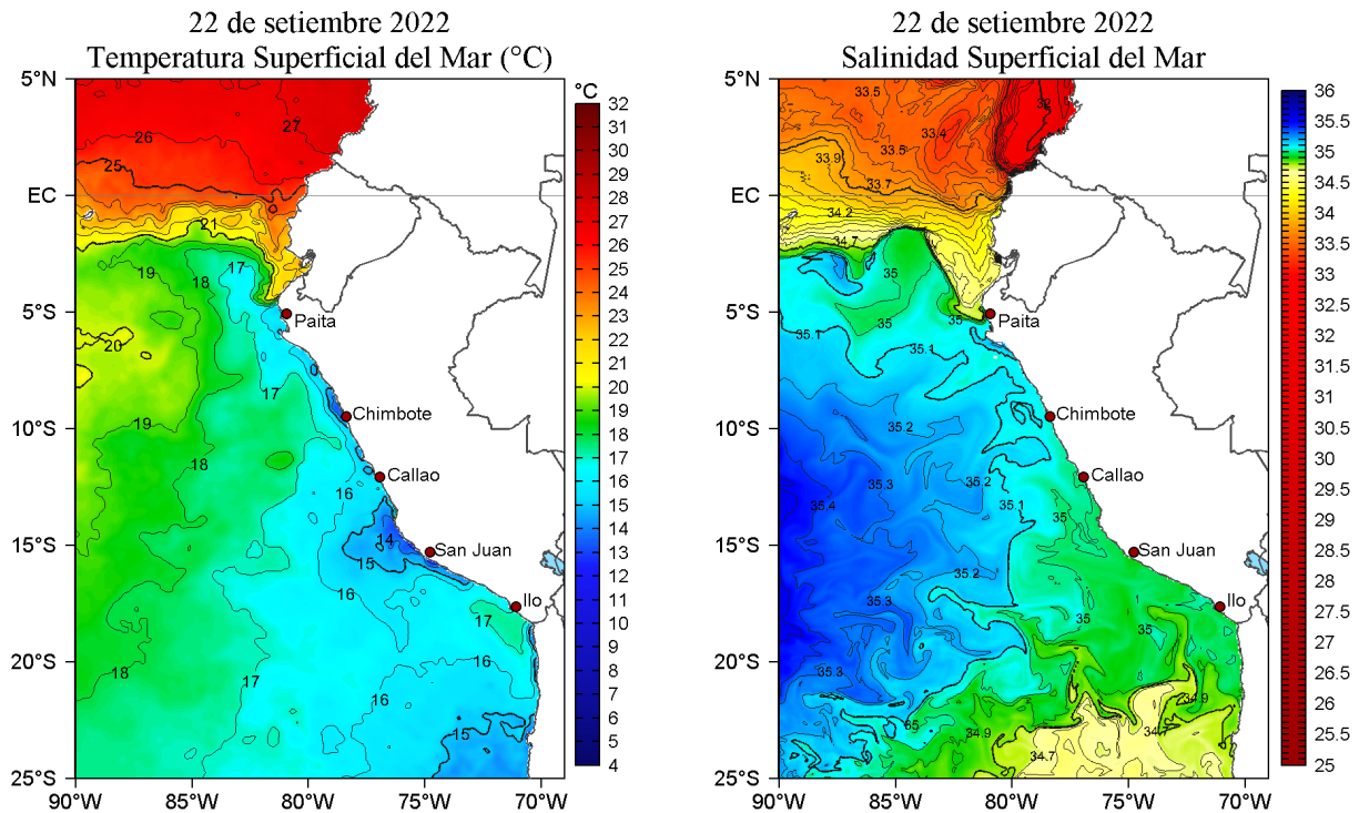
Figura 2. Temperatura superficial del mar (a la izquierda) y Salinidad superficial del mar (a la derecha) para el 22 de setiembre de 2022. Datos: OSTIA-UKMO-L4-GLOB-v2.0 (UK Met Office, 2012; Donlon et al, 2012) y Hybrid Coordinate Ocean Model v. GOFS 3.1 (HYCOM; Halliwell et al., 1998; 2000; Bleck, 2001), respectivamente.
