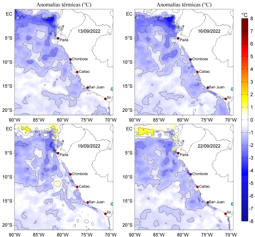
Figura 3. Anomalías de la temperatura superficial del mar (°C) para el 13, 16, 19 y 22 de setiembre de 2022. Las anomalías se calcularon respecto de la climatología para el periodo 2007-2016. Datos: OSTIA-UKMO-L4-GLOB-v2.0 (UK Met Office, 2012; Donlon et al, 2012).
