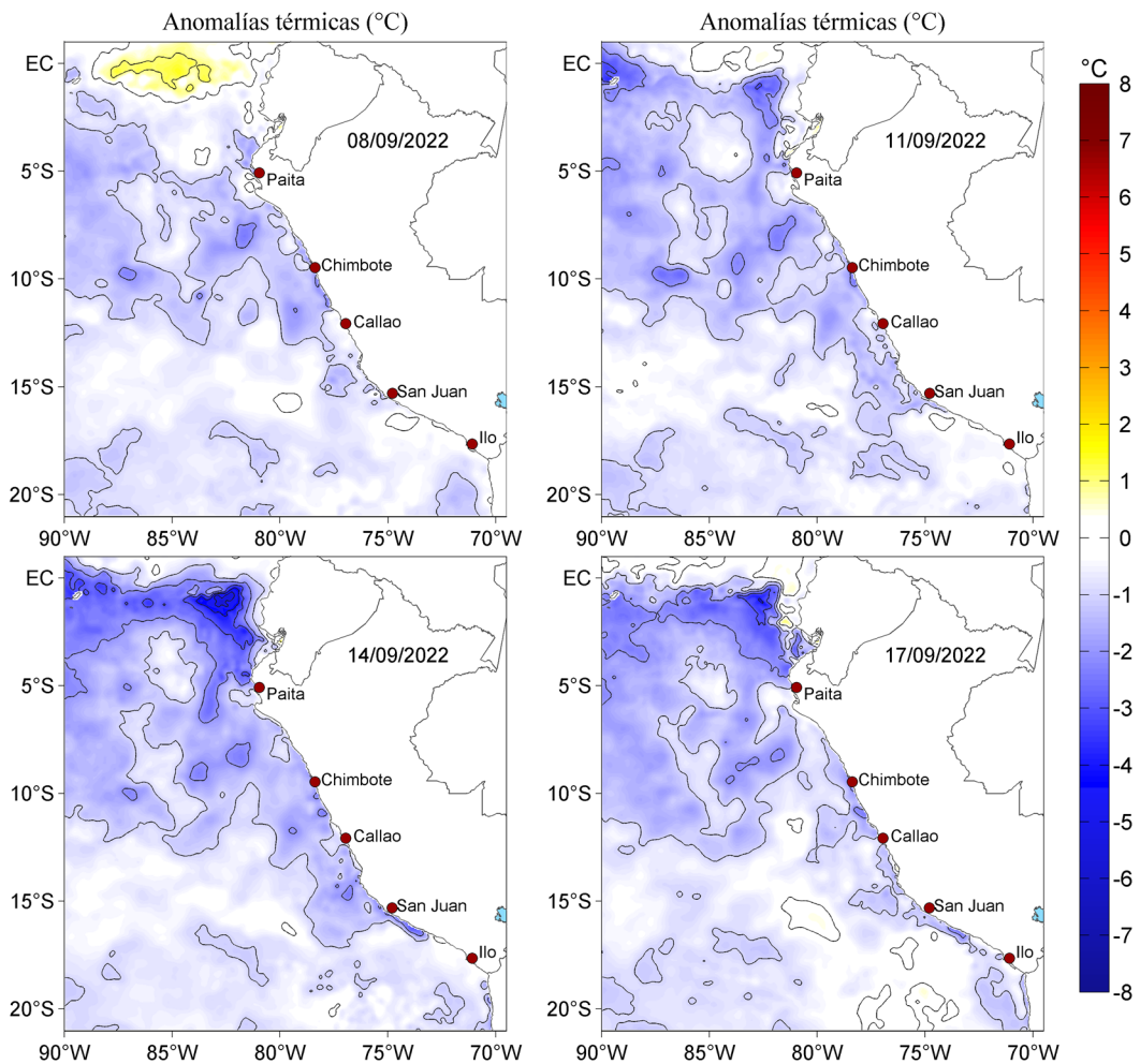
Figura 3. Anomalías de la temperatura superficial del mar (°C) para el 08, 11, 14 y 17 de setiembre de 2022. Las anomalías se calcularon respecto de la climatología para el periodo 2007-2016. Datos: OSTIA-UKMO-L4-GLOB-v2.0 (UK Met Office, 2012; Donlon et al, 2012).
