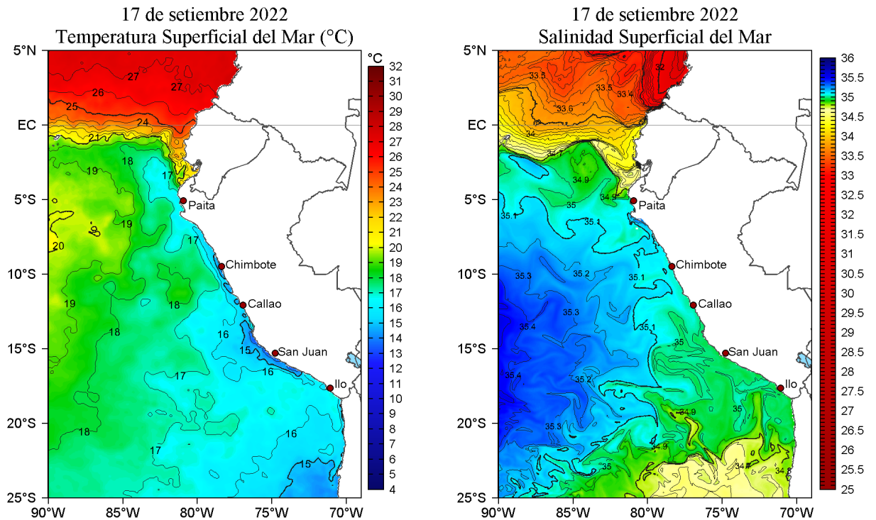
Figura 2. Temperatura superficial del mar (a la izquierda) y Salinidad superficial del mar (a la derecha) para el 17 de setiembre de 2022. Datos: OSTIA-UKMO-L4-GLOB-v2.0 (UK Met Office, 2012; Donlon et al, 2012) y Hybrid Coordinate Ocean Model v. GOFS 3.1 (HYCOM; Halliwell et al., 1998; 2000; Bleck, 2001), respectivamente.
