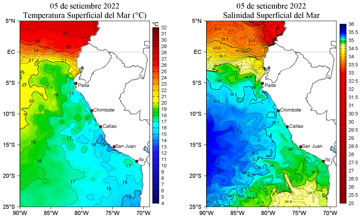
Figura 2. Temperatura superficial del mar (a la izquierda) y Salinidad superficial del mar (a la derecha) para el 05 de setiembre de 2022. Datos: OSTIA-UKMO-L4-GLOB-v2.0 (UK Met Office, 2012; Donlon et al, 2012) y Hybrid Coordinate Ocean Model v. GOFS 3.1 (HYCOM; Halliwell et al., 1998; 2000; Bleck, 2001), respectivamente.
