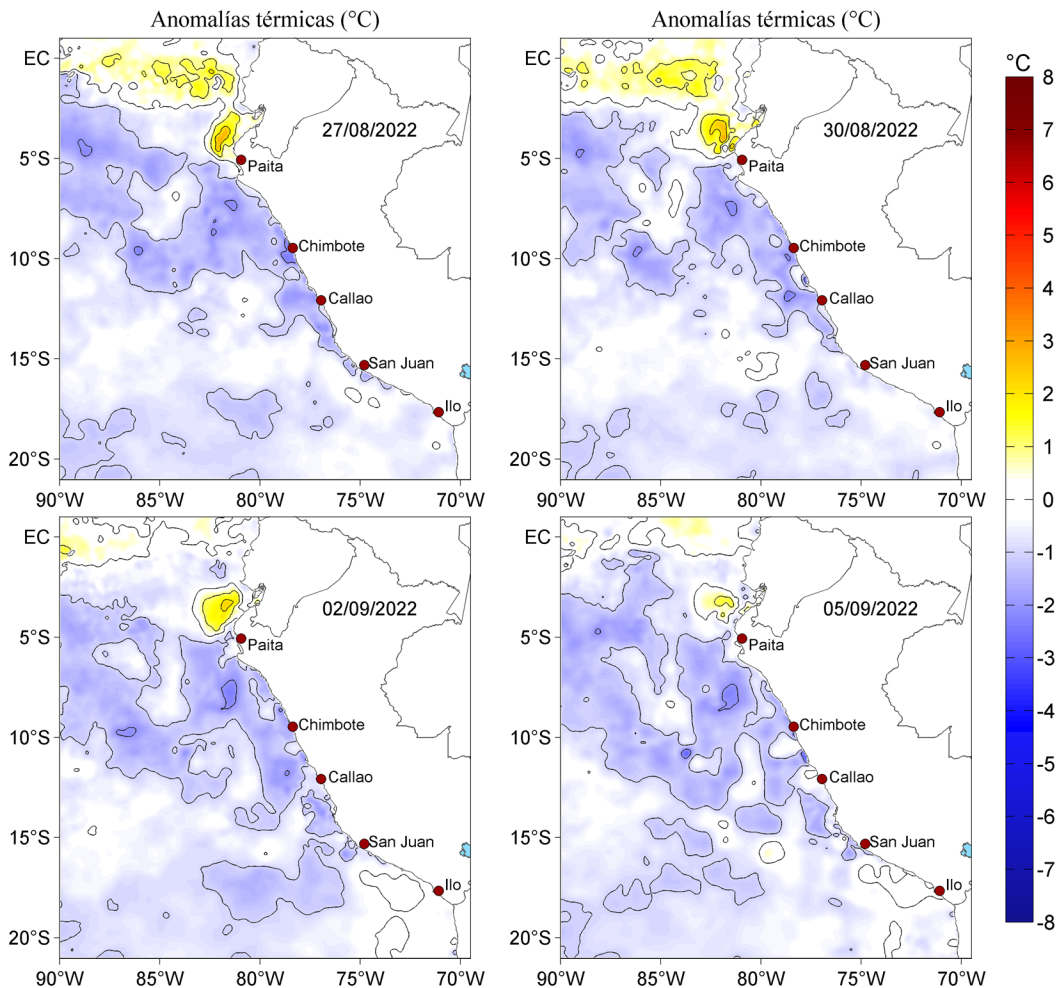
Figura 3. Anomalías de la temperatura superficial del mar (°C) para el 27 y 30 de agosto, así como para el 02 y 05 de setiembre de 2022. Las anomalías se calcularon respecto de la climatología para el periodo 2007-2016. Datos: OSTIA-UKMO-L4-GLOB-v2.0 (UK Met Office, 2012; Donlon et al, 2012).
