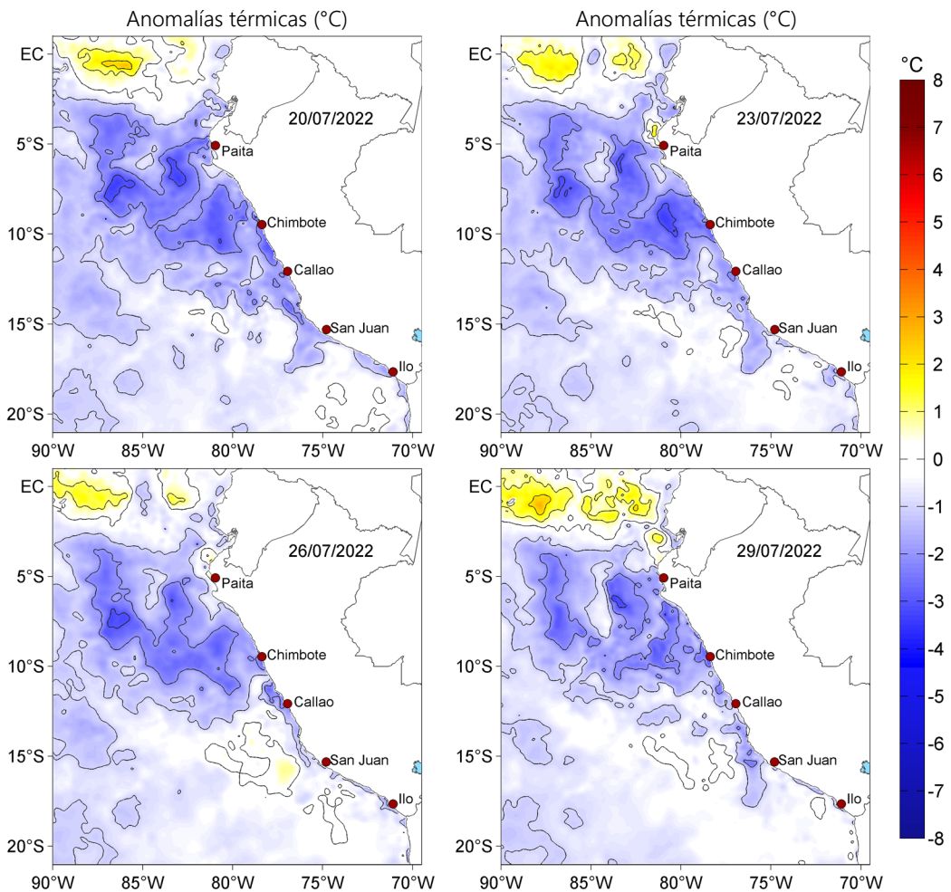
Figura 3. Anomalías de la temperatura superficial del mar (°C) para el 20, 23, 26 y 29 de julio de 2022. Las anomalías se calcularon respecto de la climatología para el periodo 2007-2016. Datos: OSTIA-UKMO-L4-GLOB-v2.0 (UK Met Office, 2012; Donlon et al, 2012).
