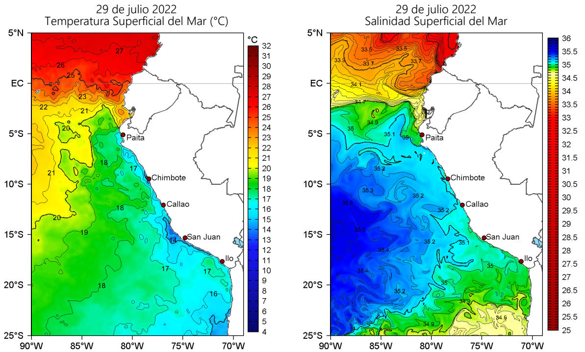
Figura 2. Temperatura superficial del mar (a la izquierda) y Salinidad superficial del mar (a la derecha) para el 29 de julio de 2022. Datos: OSTIA-UKMO-L4-GLOB-v2.0 (UK Met Office, 2012; Donlon et al, 2012) y Hybrid Coordinate Ocean Model v. GOFS 3.1 (HYCOM; Halliwell et al., 1998; 2000; Bleck, 2001), respectivamente.
