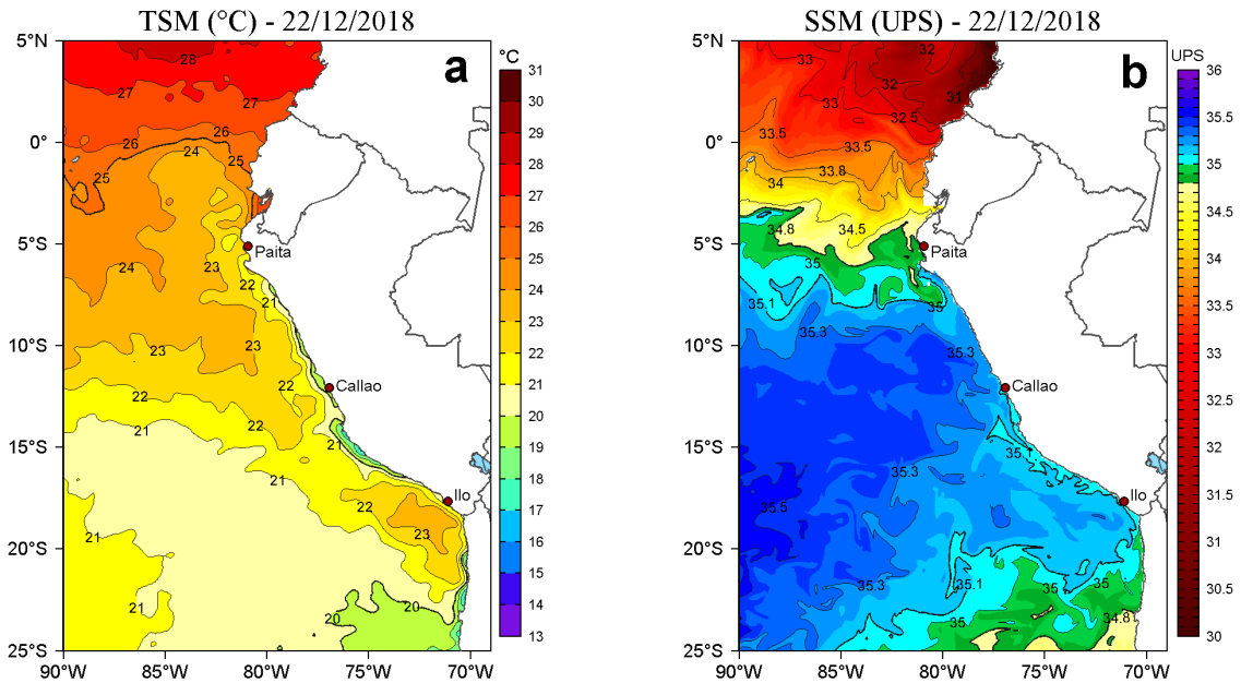
Figura 2. a) Temperatura superficial del mar (TSM, °C) y b) Salinidad superficial del mar (SSM, UPS) para el 22 de diciembre de 2018. Datos: OSTIA-UKMO-L4-GLOB-v2.0 (UK Met Office, 2012; Donlon et al, 2012) disponible en https://podaac.jpl.nasa.gov/dataset/OSTIA-UKMO-L4-GLOB-v2.0 para (a) y Hybrid Coordinate Ocean Model v. GOFS 3.1 (HYCOM; Halliwell et al., 1998; 2000; Bleck, 2001) para (b). Procesamiento: LHF/AFIOF/DGIOCC/IMARPE.
