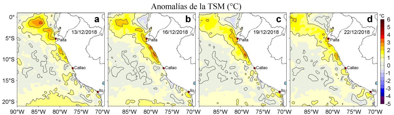
Figura 3. Anomalías de la temperatura superficial del mar (TSM, °C) para los días: a) 13, b) 16, c) 19 y d) 22 de diciembre de 2018. Las anomalías se calcularon respecto de la climatología para el periodo 2007-2016. Datos: OSTIA-UKMO-L4-GLOB-v2.0 (UK Met Office, 2012; Donlon et al, 2012). Procesamiento: LHF/AFIOF/DGIOCC/IMARPE.
