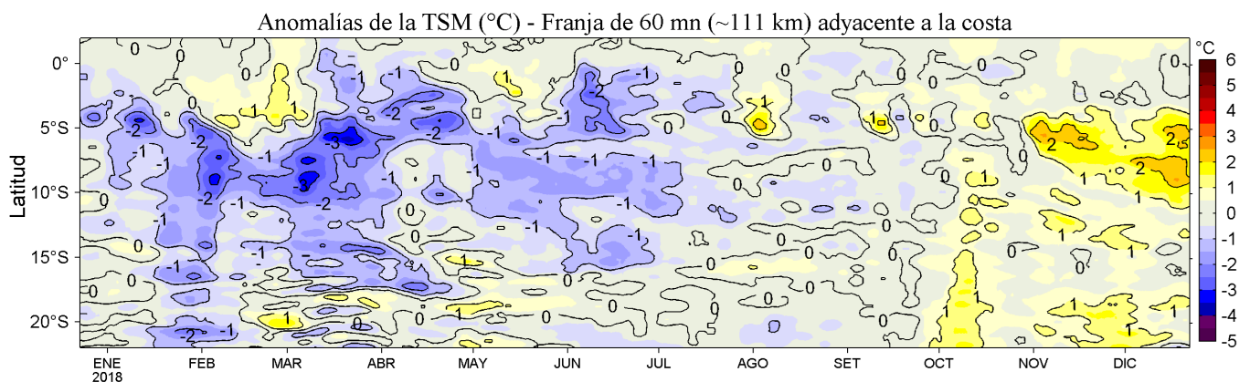
Figura 4. Variación promedio de las anomalías de la temperatura superficial del mar (TSM, °C) para una franja de 60 mn (~111 km) adyacente al litoral peruano para los últimos doce meses al 22 de diciembre de 2018. Datos: OSTIA-UKMO-L4-GLOB-v2.0 (UK Met. Office, 2012; Donlon et al, 2012) disponible en https://podaac.jpl.nasa.gov/dataset/OSTIA-UKMO-L4-GLOB-v2.0 ). Las anomalías se calcularon con respecto al periodo 2007-2016. Procesamiento: LHF/AFIOF/DGIOCC/IMARPE.
