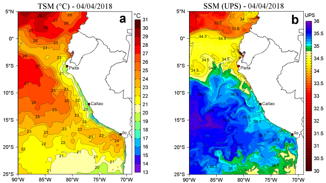
Figura 2. a) Temperatura Superficial del Mar (°C) y b) Salinidad Superficial del Mar (UPS) para el 04 de abril de 2018. Datos: OSTIA-UKMO-L4-GLOB-v2.0 (UK Met Office, 2012; Donlon et al, 2012) disponible en https://podaac.jpl.nasa.gov/dataset/OSTIA-UKMO-L4-GLOB-v2.0 para (a) y Hybrid Coordinate Ocean Model (HYCOM; Halliwell et al., 1998; 2000; Bleck, 2001) para (b). Procesamiento: LHF/AFIOF/DGIOCC/IMARPE.
