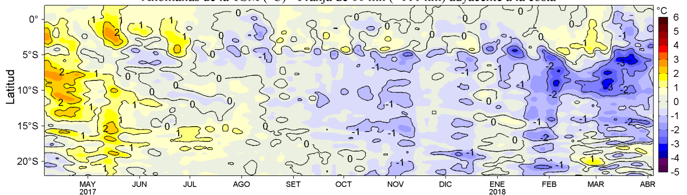
Figura 4. Variación promedio de las anomalías de la Temperatura Superficial del Mar (°C) para una franja de 60 mn (~111 km) adyacente al litoral peruano para los últimos doce meses al 04 de abril de 2018. Datos: OSTIA-UKMO-L4-GLOB-v2.0 (UK Met. Office, 2012; Donlon et al, 2012) disponible en https://podaac.jpl.nasa.gov/dataset/OSTIA-UKMO-L4-GLOB-v2.0 . Las anomalías se calcularon con respecto al periodo 2007-2016. Procesamiento: LHF/AFIOF/DGIOCC/IMARPE.
