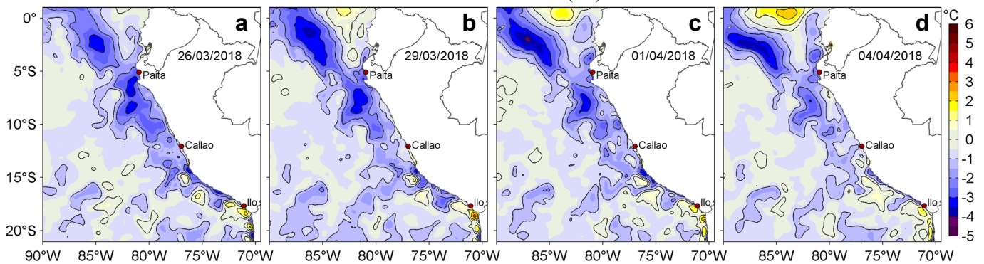
Figura 3. Anomalías de la Temperatura Superficial del Mar (°C) para los días: a) 26, b) 29 de marzo, c) 01 y d) 04 de abril de 2018. Las anomalías se calcularon respecto de la climatología para el periodo 2007-2016. Datos: OSTIA-UKMO-L4-GLOB-v2.0 (UK Met Office, 2012; Donlon et al, 2012). Procesamiento: LHF/AFIOF/DGIOCC/IMARPE.
