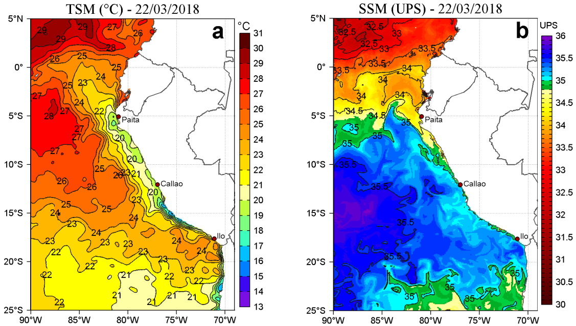
Figura 2. a) Temperatura Superficial del Mar ( ^{\circ}\text{C} ) y b) Salinidad Superficial del Mar (UPS) para el 22 de marzo de 2018. Datos: OSTIA-UKMO-L4-GLOB-v2.0 (UK Met Office, 2012; Donlon et al, 2012) disponible en https://podaac.jpl.nasa.gov/dataset/OSTIA-UKMO-L4-GLOB-v2.0 para (a) y Hybrid Coordinate Ocean Model (HYCOM; Halliwell et al., 1998; 2000; Bleck, 2001) para (b). Procesamiento: LHFM/AFIOF/DGIOCC/IMARPE.
