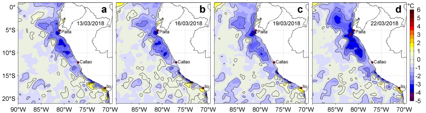
Figura 3. Anomalías de la Temperatura Superficial del Mar ( ^{\circ}\text{C} ) para los días: a) 13, b) 16, c) 19 y d) 22 de marzo de 2018. Las anomalías se calcularon respecto de la climatología para el periodo 2007-2016. Datos: OSTIA-UKMO-L4-GLOB-v2.0 (UK Met Office, 2012; Donlon et al, 2012). Procesamiento: LHFM/AFIOF/DGIOCC/IMARPE.
