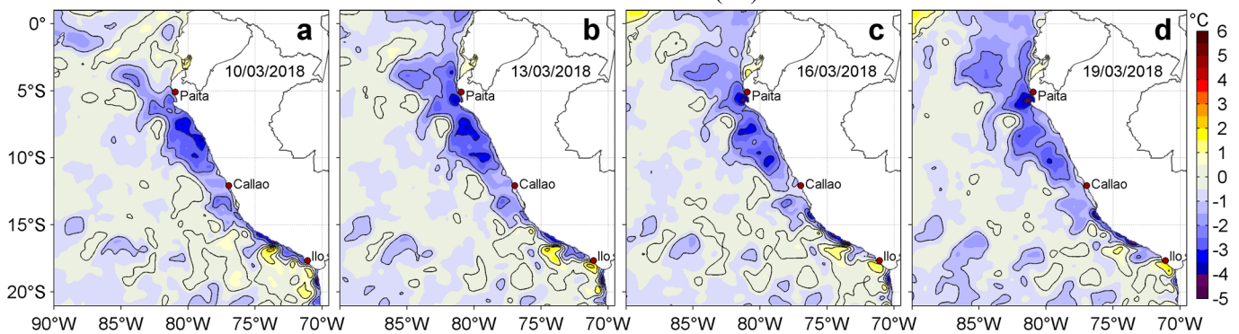
Figura 3. Anomalías de la Temperatura Superficial del Mar (°C) para los días: a) 10, b) 13, c) 16 y d) 19 de marzo de 2018. Las anomalías se calcularon respecto de la climatología para el periodo 2007-2016. Datos: OSTIA-UKMO-L4-GLOB-v2.0 (UK Met Office, 2012; Donlon et al, 2012). Procesamiento: LHF/AFIOF/DGIOCC/IMARPE.
