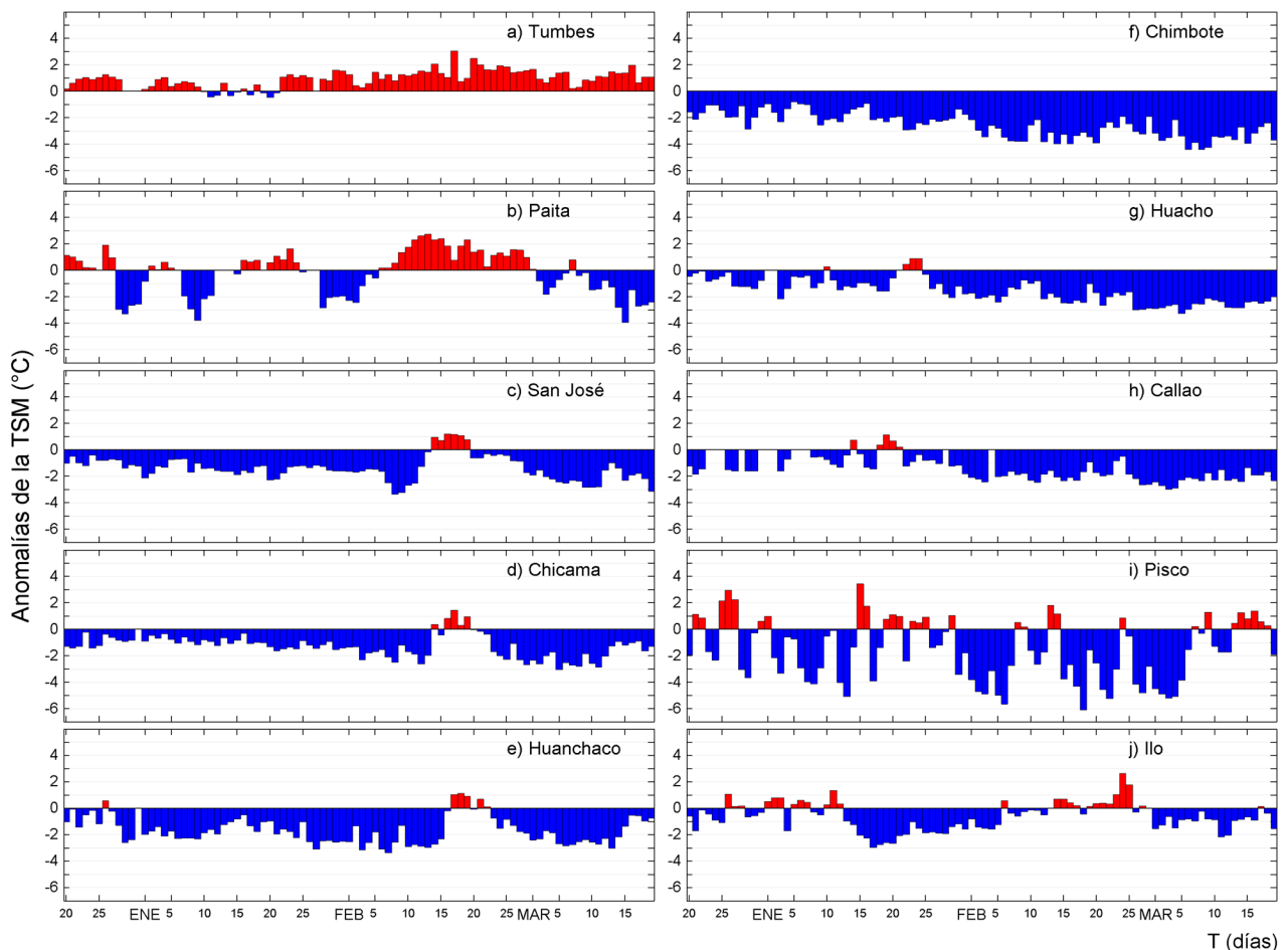
Figura 5. Variación del promedio diario de las anomalías de la TSM (°C) en la red de estaciones costeras que administra IMARPE en el litoral peruano durante el último trimestre. Las anomalías se calcularon respecto del promedio climatológico pentadal (5 días) para el periodo que se indica en la Tabla 1. Datos y procesamiento: LHFM/AFIOF/DGIOCC/IMARPE.
