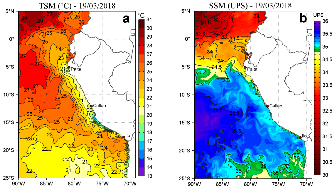
Figura 2. a) Temperatura superficial del mar (°C) y b) Salinidad superficial del mar (UPS) para el 19 de marzo de 2018. Datos: OSTIA-UKMO-L4-GLOB-v2.0 (UK Met Office, 2012; Donlon et al, 2012) disponible en https://podaac.jpl.nasa.gov/dataset/OSTIA-UKMO-L4-GLOB-v2.0 para (a) y Hybrid Coordinate Ocean Model (HYCOM; Halliwell et al., 1998; 2000; Bleck, 2001) para (b). Procesamiento: LHF/AFIOF/DGIOCC/IMARPE.
