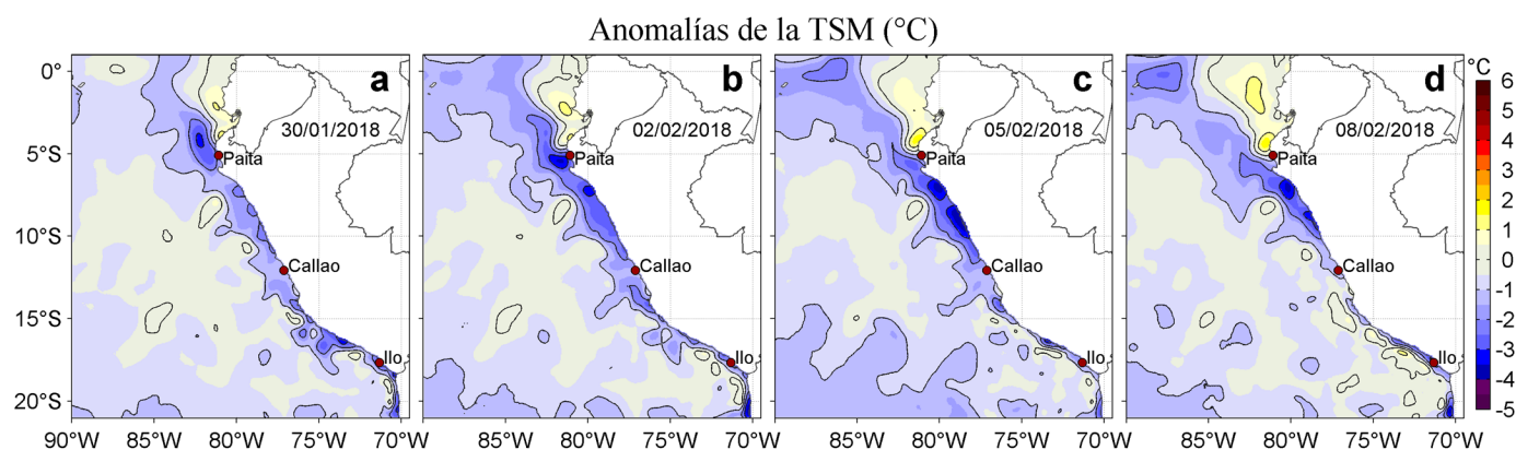
Figura 3. Anomalías de la Temperatura Superficial del Mar ( ^{\circ}\text{C} ) para los días: a) 30 de enero, b) 02, c) 05 y d) 08 de febrero de 2018. Las anomalías se calcularon respecto de la climatología para el periodo 2007-2016. Datos: OSTIA-UKMO-L4-GLOB-v2.0 (UK Met Office, 2012; Donlon et al, 2012). Procesamiento: LHF/AFIOF/DGIOCC/IMARPE.
