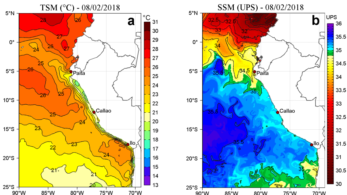
Figura 2. a) Temperatura Superficial del Mar ( ^{\circ}\text{C} ) y b) Salinidad Superficial del Mar (UPS) para el 08 de febrero de 2018. Datos: OSTIA-UKMO-L4-GLOB-v2.0 (UK Met Office, 2012; Donlon et al, 2012) disponible en https://podaac.jpl.nasa.gov/dataset/OSTIA-UKMO-L4-GLOB-v2.0 para (a) y Hybrid Coordinate Ocean Model (HYCOM; Halliwell et al., 1998; 2000; Bleck, 2001) para (b). Procesamiento: LHF/AFIOF/DGIOCC/IMARPE.
