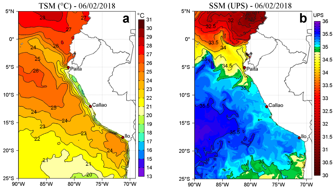
Figura 2. a) Temperatura superficial del mar ( ^{\circ}\text{C} ) y b) Salinidad superficial del mar (UPS) para el 06 de febrero de 2018. Datos: OSTIA-UKMO-L4-GLOB-v2.0 (UK Met Office, 2012; Donlon et al, 2012) disponible en https://podaac.jpl.nasa.gov/dataset/OSTIA-UKMO-L4-GLOB-v2.0 para (a) y Hybrid Coordinate Ocean Model (HYCOM; Halliwell et al., 1998; 2000; Bleck, 2001) para (b). Procesamiento: LHF/AFIOF/DGIOCC/IMARPE.
