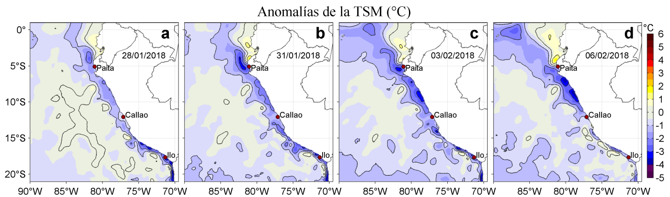
Figura 3. Anomalías de la Temperatura Superficial del Mar ( ^{\circ}\text{C} ) para los días: a) 28, b) 31 de enero, c) 03 y d) 06 de febrero de 2018. Las anomalías se calcularon respecto de la climatología para el periodo 2007-2016. Datos: OSTIA-UKMO-L4-GLOB-v2.0 (UK Met Office, 2012; Donlon et al, 2012). Procesamiento: LHF/AFIOF/DGIOCC/IMARPE.
