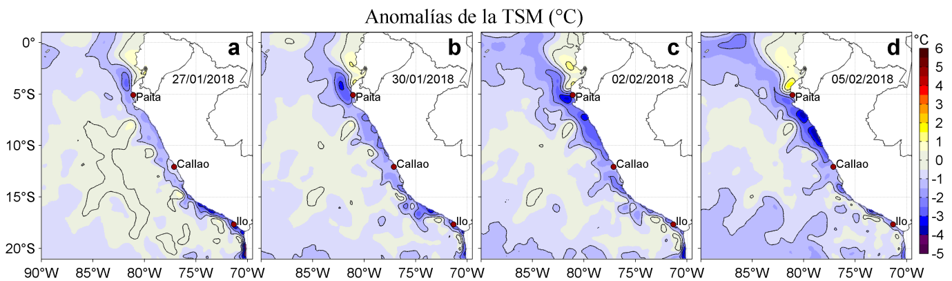
Figura 3. Anomalías de la Temperatura Superficial del Mar ( ^{\circ}\text{C} ) para los días: a) 27, b) 30 de enero, c) 02 y d) 05 de febrero de 2018. Las anomalías se calcularon respecto de la climatología para el periodo 2007-2016. Datos: OSTIA-UKMO-L4-GLOB-v2.0 (UK Met Office, 2012; Donlon et al, 2012). Procesamiento: LHF/AFIOF/DGIOCC/IMARPE.
