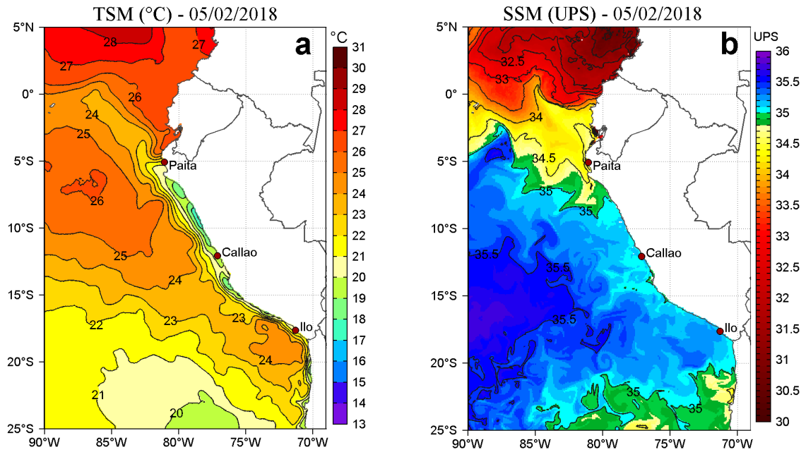
Figura 2. a) Temperatura superficial del mar ( ^{\circ}\text{C} ) y b) Salinidad superficial del mar (UPS) para el 05 de febrero de 2018. Datos: OSTIA-UKMO-L4-GLOB-v2.0 (UK Met Office, 2012; Donlon et al, 2012) disponible en https://podaac.jpl.nasa.gov/dataset/OSTIA-UKMO-L4-GLOB-v2.0 para (a) y Hybrid Coordinate Ocean Model (HYCOM; Halliwell et al., 1998; 2000; Bleck, 2001) para (b). Procesamiento: LHF/AFIOF/DGIOCC/IMARPE.
