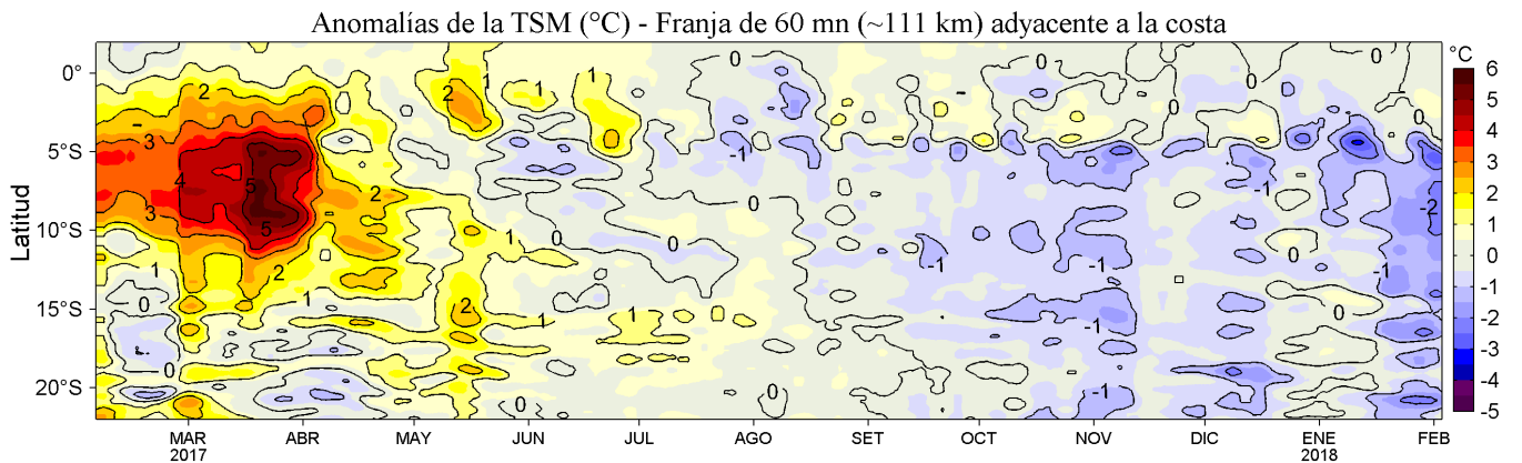
Figura 4. Variación promedio de las anomalías de la Temperatura Superficial del Mar (°C) para una franja de 60 mn (~111 km) adyacente al litoral peruano para los últimos doce meses al 03 de febrero de 2018. Datos: OSTIA-UKMO-L4-GLOB-v2.0 (UK Met. Office, 2012; Donlon et al, 2012) disponible en https://podaac.jpl.nasa.gov/dataset/OSTIA-UKMO-L4-GLOB-v2.0 . Las anomalías se calcularon con respecto al periodo 2007-2016. Procesamiento: LHFM/AFIOF/DGIOCC/IMARPE.
