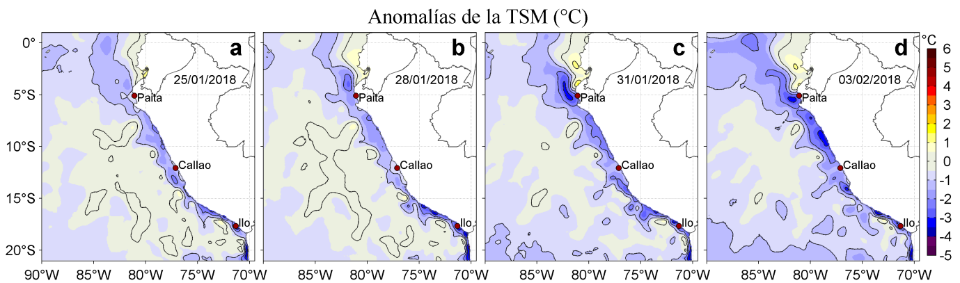
Figura 3. Anomalías de la Temperatura Superficial del Mar (°C) para los días: a) 25, b) 28, c) 31 de enero de 2018 y d) 03 de febrero de 2018. Las anomalías se calcularon respecto de la climatología para el periodo 2007-2016. Datos: OSTIA-UKMO-L4-GLOB-v2.0 (UK Met Office, 2012; Donlon et al, 2012). Procesamiento: LHFM/AFIOF/DGIOCC/IMARPE.
