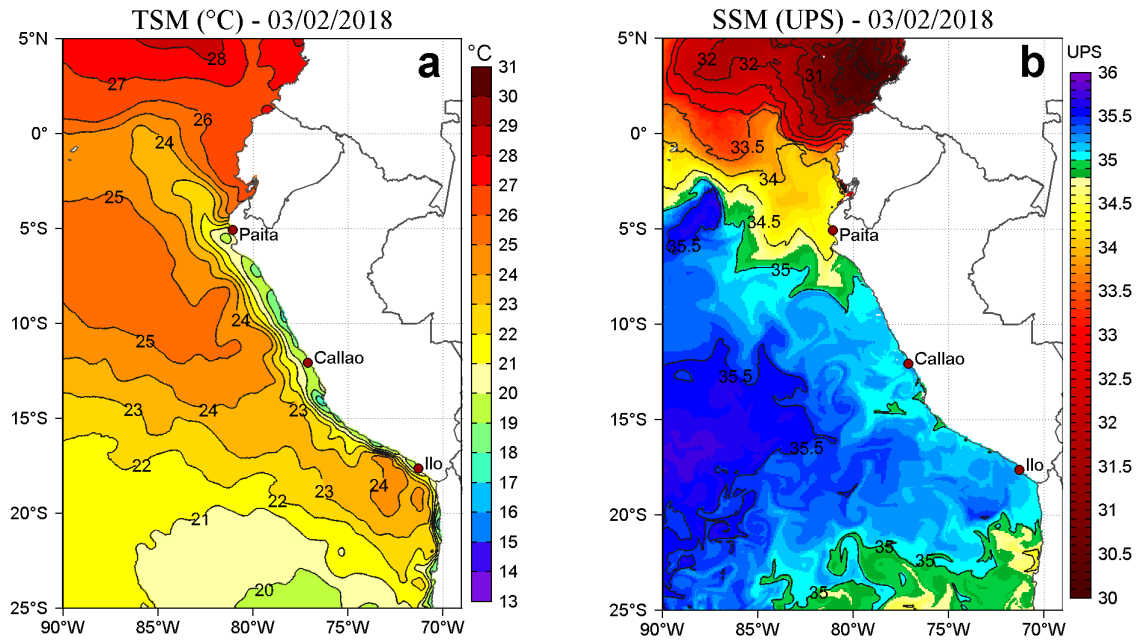
Figura 2. a) Temperatura superficial del mar (°C) y b) Salinidad superficial del mar (UPS) para el 03 de febrero de 2018. Datos: OSTIA-UKMO-L4-GLOB-v2.0 (UK Met Office, 2012; Donlon et al, 2012) disponible en https://podaac.jpl.nasa.gov/dataset/OSTIA-UKMO-L4-GLOB-v2.0 para (a) y Hybrid Coordinate Ocean Model (HYCOM; Halliwell et al., 1998; 2000; Bleck, 2001) para (b). Procesamiento: LHFM/AFIOF/DGIOCC/IMARPE.
