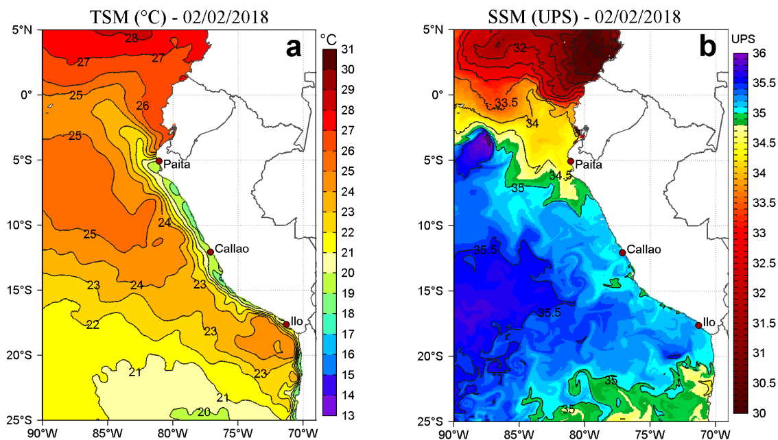
Figura 2. a) Temperatura superficial del mar (°C) y b) Salinidad superficial del mar (UPS) para el 02 de febrero de 2018. Datos: OSTIA-UKMO-L4-GLOB-v2.0 (UK Met Office, 2012; Donlon et al, 2012) disponible en https://podaac.jpl.nasa.gov/dataset/OSTIA-UKMO-L4-GLOB-v2.0 para (a) y Hybrid Coordinate Ocean Model (HYCOM; Halliwell et al., 1998; 2000; Bleck, 2001) para (b). Procesamiento: LHFM/AFIOF/DGIOCC/IMARPE.
