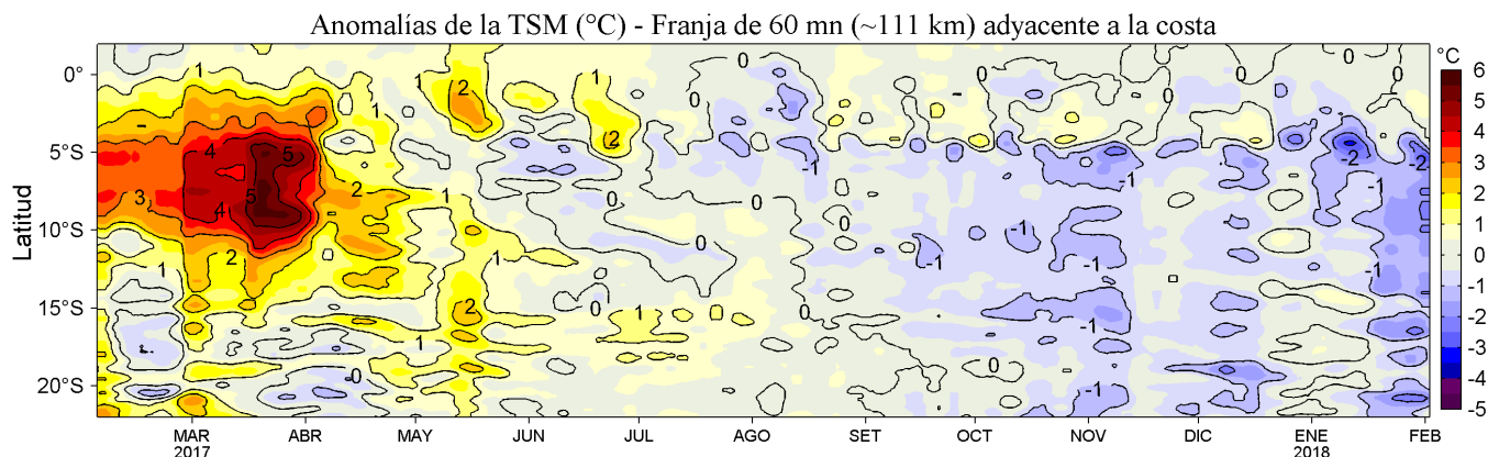
Figura 4. Variación promedio de las anomalías de la Temperatura Superficial del Mar (°C) para una franja de 60 mn (~111 km) adyacente al litoral peruano para los últimos doce meses al 02 de febrero de 2018. Datos: OSTIA-UKMO-L4-GLOB-v2.0 (UK Met. Office, 2012; Donlon et al, 2012) disponible en https://podaac.jpl.nasa.gov/dataset/OSTIA-UKMO-L4-GLOB-v2.0 . Las anomalías se calcularon con respecto al periodo 2007-2016. Procesamiento: LHFM/AFIOF/DGIOCC/IMARPE.
