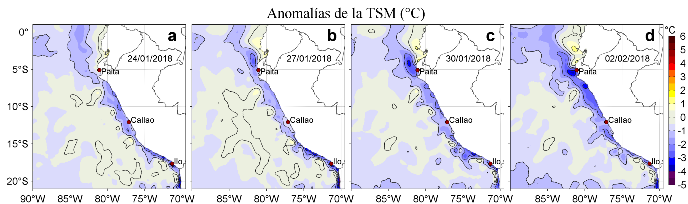
Figura 3. Anomalías de la Temperatura Superficial del Mar (°C) para los días: a) 24, b) 27, c) 30 de enero de 2018 y d) 02 de febrero de 2018. Las anomalías se calcularon respecto de la climatología para el periodo 2007-2016. Datos: OSTIA-UKMO-L4-GLOB-v2.0 (UK Met Office, 2012; Donlon et al, 2012). Procesamiento: LHFM/AFIOF/DGIOCC/IMARPE.
