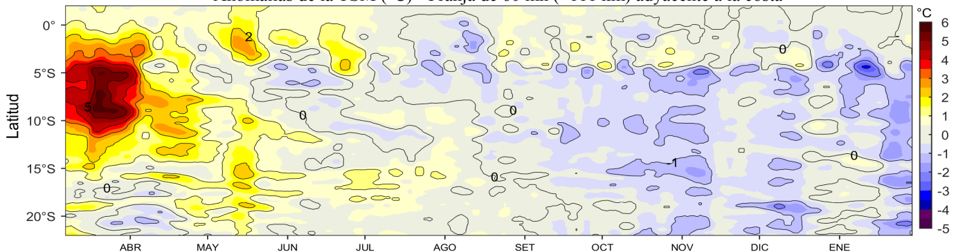
Figura 4. Variación promedio de las anomalías de la Temperatura Superficial del Mar (°C) para una franja de 60 mn (~111 km) adyacente al litoral peruano para los últimos doce meses al 29 de enero de 2018. Datos: OSTIA-UKMO-L4-GLOB-v2.0 (UK Met. Office, 2012; Donlon et al, 2012) disponible en https://podaac.jpl.nasa.gov/dataset/OSTIA-UKMO-L4-GLOB-v2.0 . Las anomalías se calcularon con respecto al periodo 2007-2016. Procesamiento: LHF/AFIOF/DGIOCC/IMARPE.
