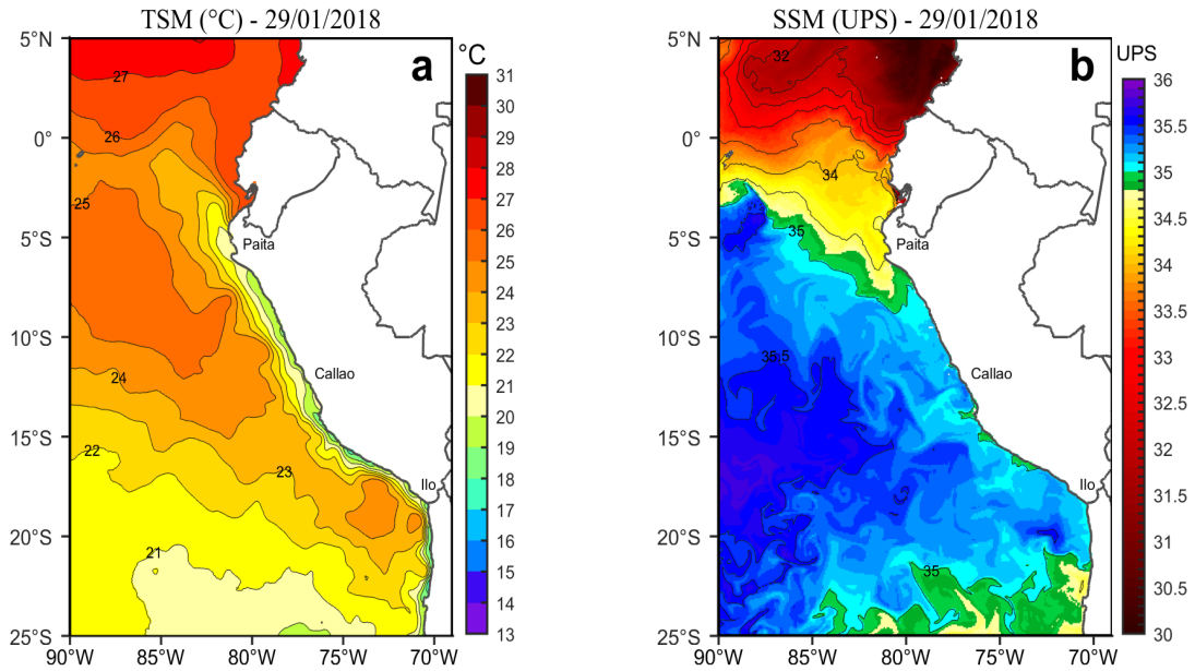
Figura 2. a) Temperatura superficial del mar (°C) y b) Salinidad superficial del mar (UPS) para el 29 de enero de 2018. Datos: OSTIA-UKMO-L4-GLOB-v2.0 (UK Met Office, 2012; Donlon et al, 2012) disponible en https://podaac.jpl.nasa.gov/dataset/OSTIA-UKMO-L4-GLOB-v2.0 para (a) y Hybrid Coordinate Ocean Model (HYCOM; Halliwell et al., 1998; 2000; Bleck, 2001) para (b). Procesamiento: LHF/AFIOF/DGIOCC/IMARPE.
