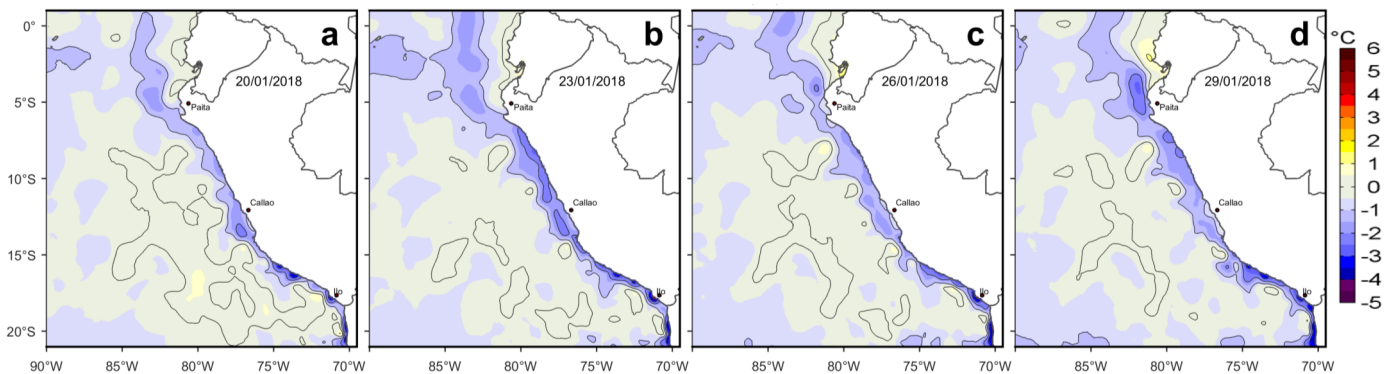
Figura 3. Anomalías de la Temperatura Superficial del Mar (°C) para los días: a) 20, b) 23, c) 26 y d) 29 de enero de 2018. Las anomalías se calcularon respecto de la climatología para el periodo 2007-2016. Datos: OSTIA-UKMO-L4-GLOB-v2.0 (UK Met Office, 2012; Donlon et al, 2012). Procesamiento: LHF/AFIOF/DGIOCC/IMARPE.
