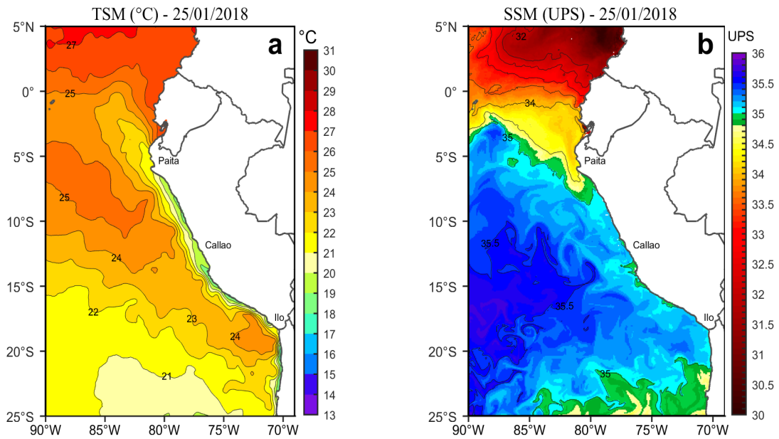
Figura 2. a) Temperatura superficial del mar ( ^{\circ}\text{C} ) y b) Salinidad superficial del mar (UPS) para el 25 de enero de 2018. Datos: OSTIA-UKMO-L4-GLOB-v2.0 (UK Met Office, 2012; Donlon et al, 2012) disponible en https://podaac.jpl.nasa.gov/dataset/OSTIA-UKMO-L4-GLOB-v2.0 para (a) y Hybrid Coordinate Ocean Model (HYCOM; Halliwell et al., 1998; 2000; Bleck, 2001) para (b). Procesamiento: LHF/AFIOF/DGIOCC/IMARPE.
