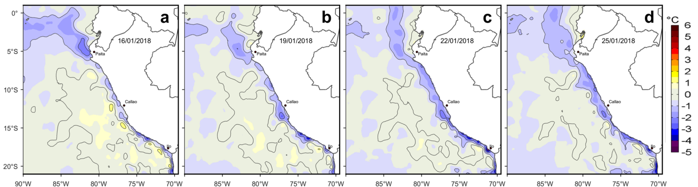
Figura 3. Anomalías de la Temperatura Superficial del Mar ( ^{\circ}\text{C} ) para los días: a) 16, b) 19, c) 22 y d) 25 de enero de 2018. Las anomalías se calcularon respecto de la climatología para el periodo 2007-2016. Datos: OSTIA-UKMO-L4-GLOB-v2.0 (UK Met Office, 2012; Donlon et al, 2012). Procesamiento: LHF/AFIOF/DGIOCC/IMARPE.
