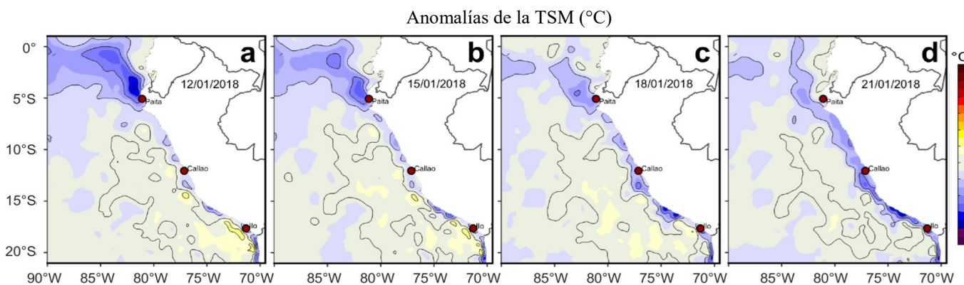
Figura 3. Anomalías de la Temperatura Superficial del Mar ( ^{\circ}\text{C} ) para los días: a) 12, b) 15, c) 18 y d) 21 de enero de 2018. Las anomalías se calcularon respecto de la climatología para el periodo 2007-2016. Datos: OSTIA-UKMO-L4-GLOB-v2.0 (UK Met Office, 2012; Donlon et al, 2012). Procesamiento: LHF/AFIOF/DGIOCC/IMARPE.
