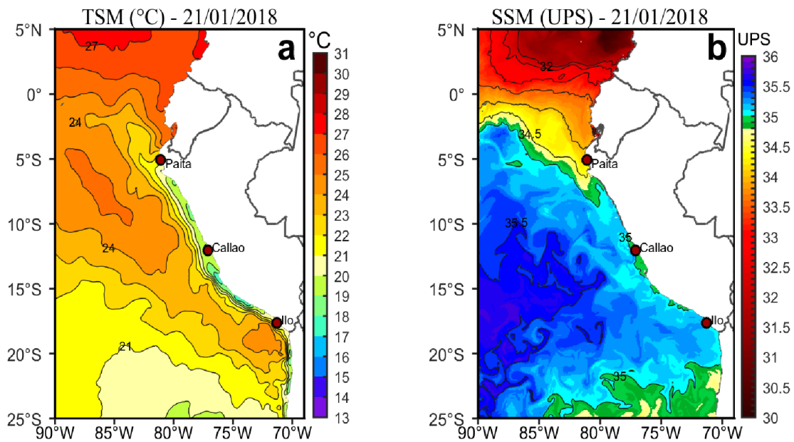
Figura 2. a) Temperatura superficial del mar ( ^{\circ}\text{C} ) y b) Salinidad superficial del mar (UPS) para el 21 de enero de 2018. Datos: OSTIA-UKMO-L4-GLOB-v2.0 (UK Met Office, 2012; Donlon et al, 2012) disponible en https://podaac.jpl.nasa.gov/dataset/OSTIA-UKMO-L4-GLOB-v2.0 para (a) y Hybrid Coordinate Ocean Model (HYCOM; Halliwell et al., 1998; 2000; Bleck, 2001) para (b). Procesamiento: LHF/AFIOF/DGIOCC/IMARPE.
